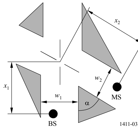
图3 对 NLoS2 情况的参数的规定
