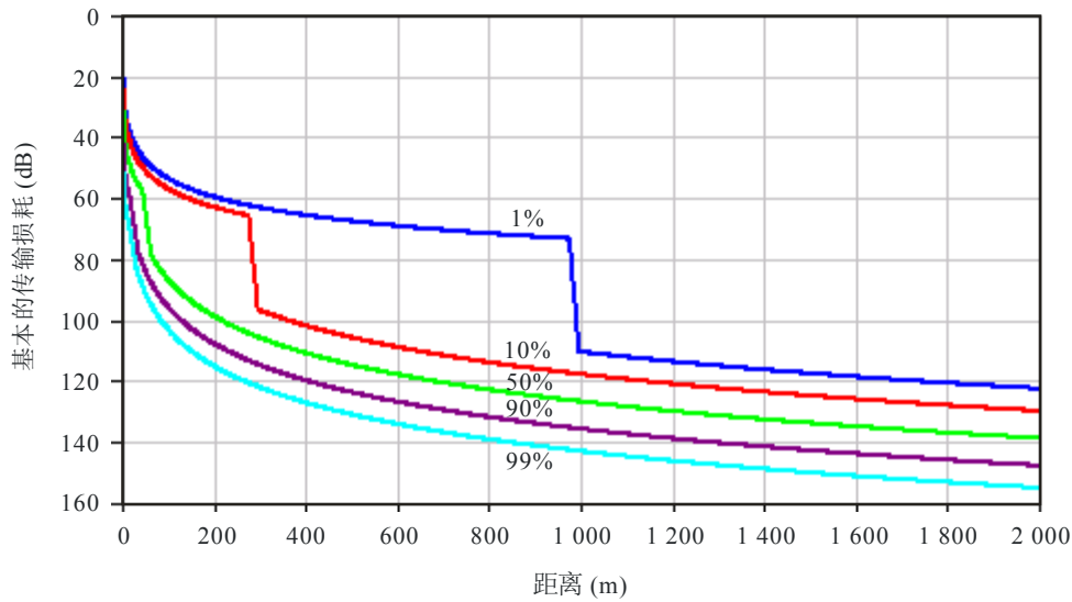
图5 不超过1%、10%、50%、90%和99%位置的基本传输损耗曲线 (频率=400 MHz, 郊区)
