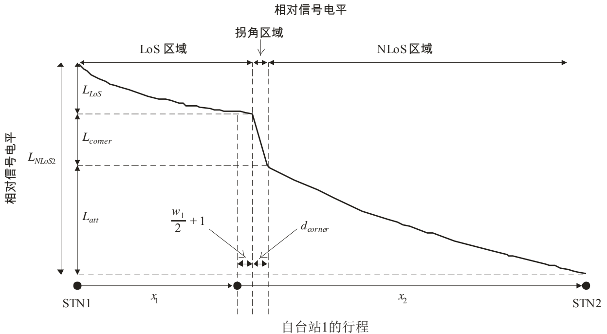
图4 2-16 GHz频率范围内低台站高度情况下 沿街道峡谷传播的典型趋势
