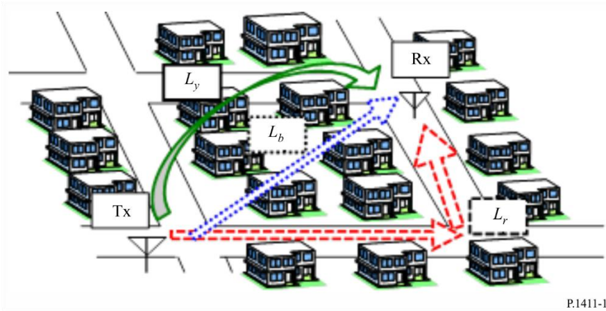
FIGURE 10 Modèle de propagation pour des trajets entre des terminaux situés au-dessous de la hauteur des toits
