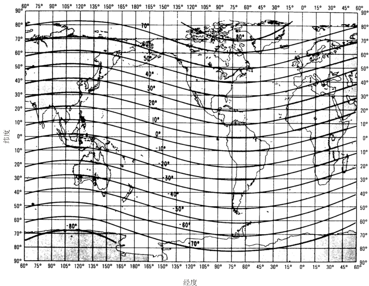
图 2 地磁纬度
