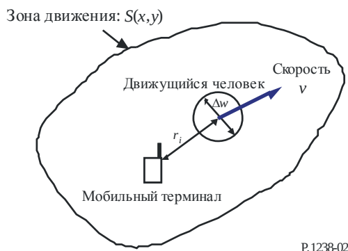
РИСУНОК 2 Модель системы
