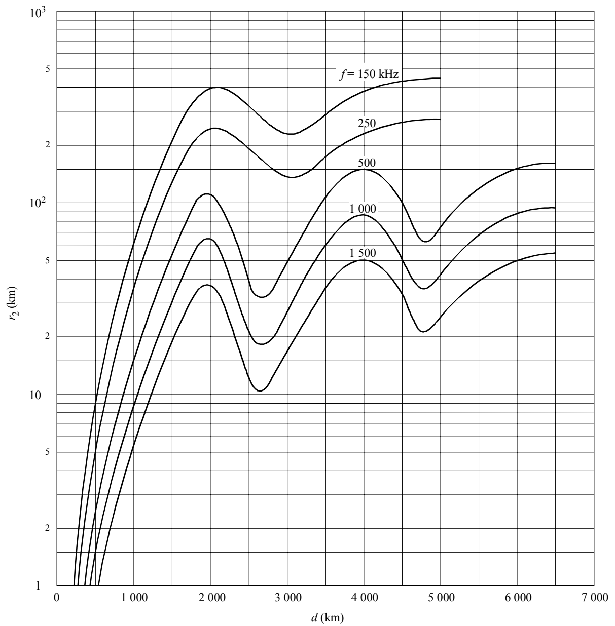
FIGURE 8b Valeurs de r_2 pour diverses fréquences
