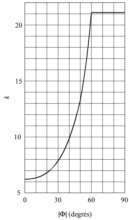
FIGURE 9 Coefficient d'affaiblissement de transmission de référence
