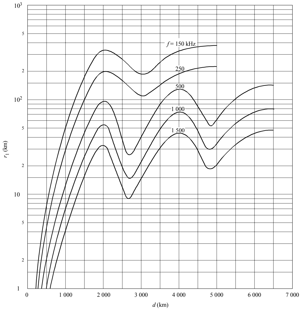
FIGURE 8a Valeurs de r_1 pour diverses fréquences
