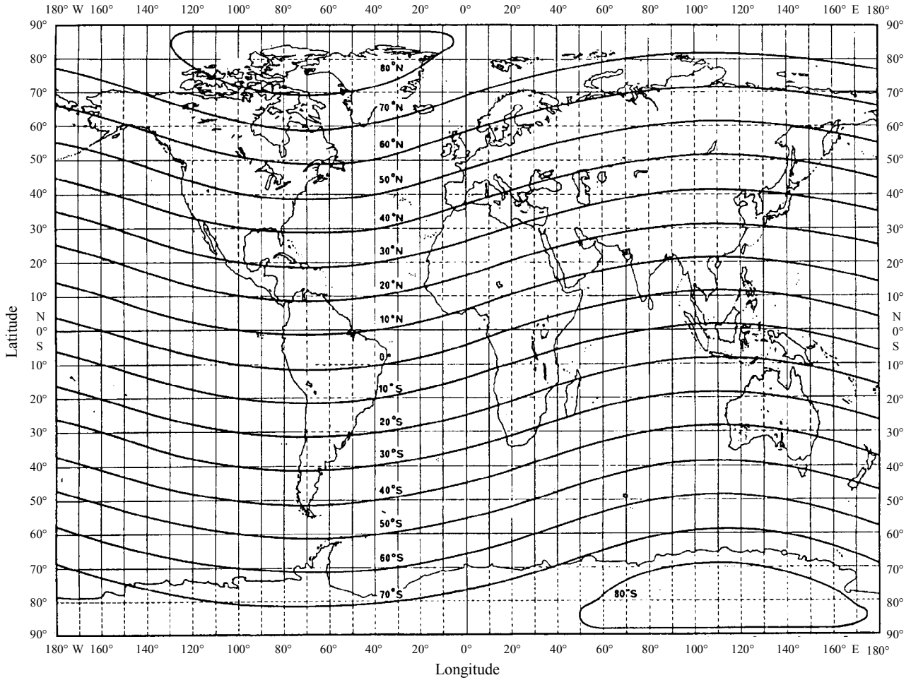
FIGURE 10 Latitudes géomagnétiques
