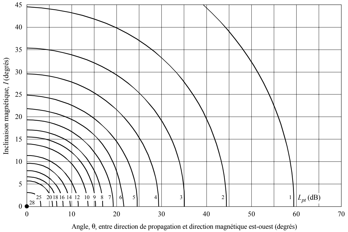
FIGURE 7 Surcroît d'affaiblissement par couplage de polarisation L_p (pour une seule extrémité)
