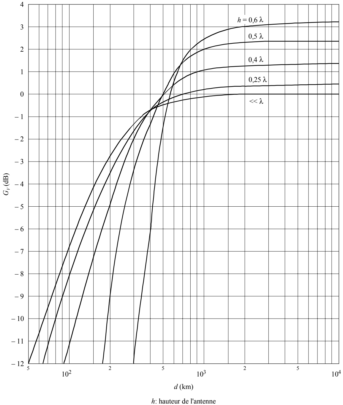
FIGURE 1 Gain de l'antenne d'émission ( G_r ) pour des antennes verticales simples au-dessus d'un sol parfait
