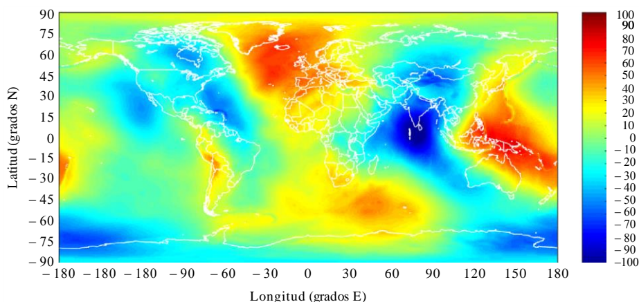
FIGURA 5 EGM2008 (m)
