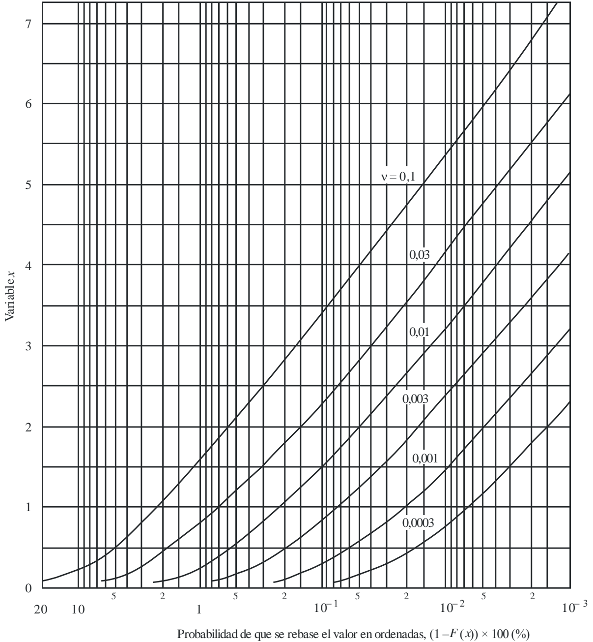
FIGURA 5 Distribución gamma ( \alpha = 1, \nu \leq 0,1 )
