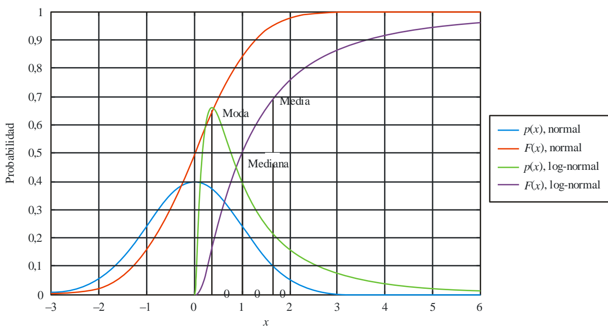
FIGURA 1 Distribución normal y log-normal
