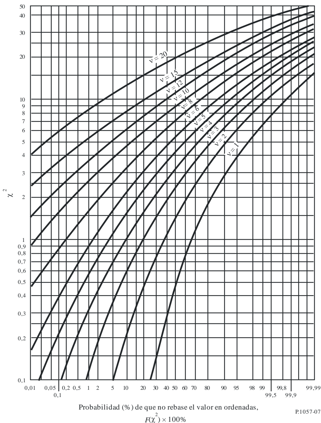
FIGURA 7 Distribución \chi^2
