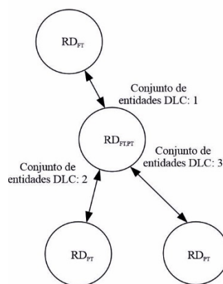
FIGURA 62 Conjuntos de entidades DLC para los RD en modo FT y PT
