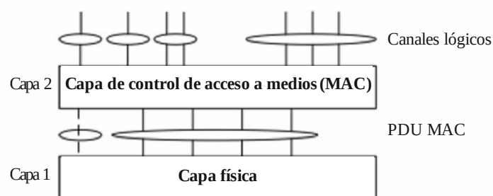
FIGURA 58 Arquitectura del protocolo de interfaz de la interfaz radioeléctrica
