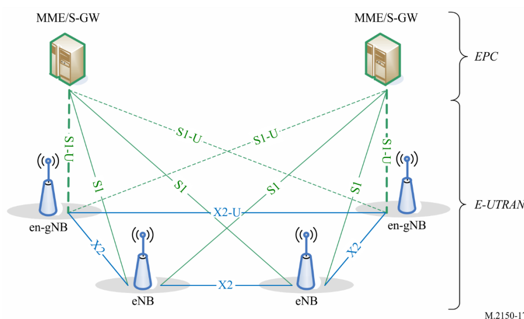
FIGURA 17 Arquitectura general de EN-DC
