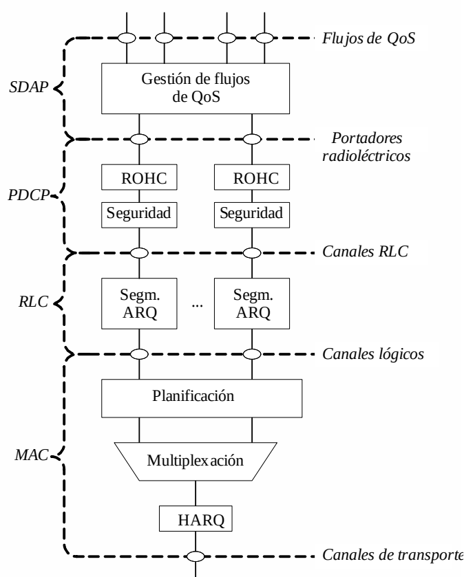
FIGURA 73 Estructura de la capa 2 del enlace ascendente
