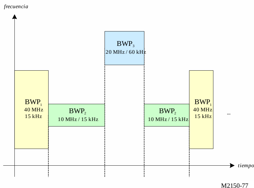
FIGURA 77 Ejemplo de BA
