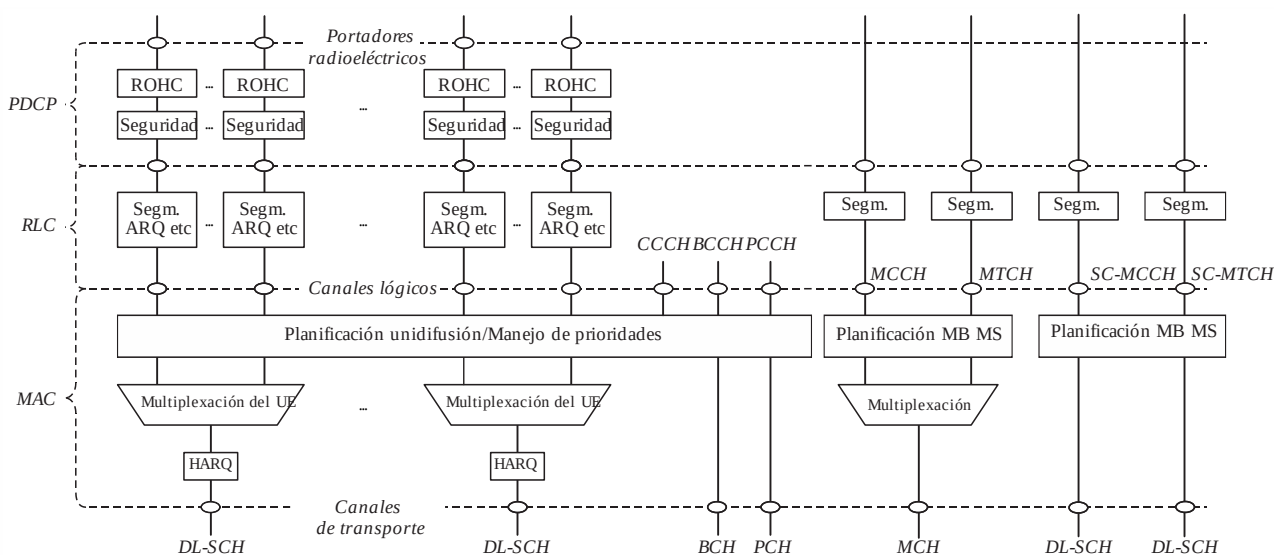
FIGURA 2 Estructura del protocolo L2 del enlace descendente
