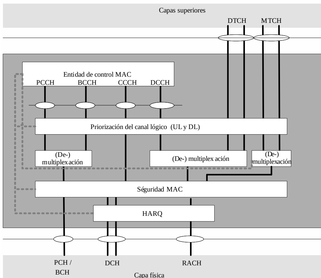
FIGURA 60 Resumen de la estructura de la capa MAC
