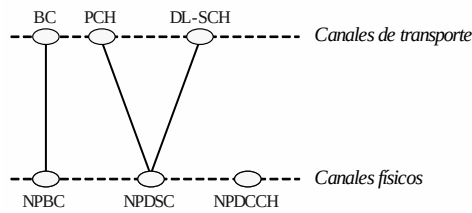
FIGURA 7 Configuración del canal NB-IoT descendente
