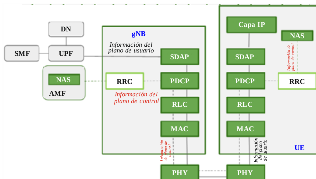
FIGURA 44 Arquitectura de la capa lógica de la RIT de la TSDSI
