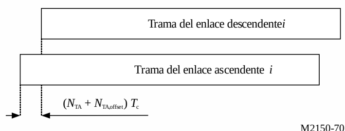
FIGURA 70 Relación de temporización entre el enlace ascendente y el descendente
