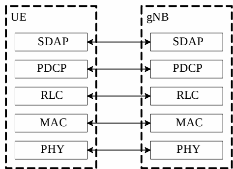
FIGURA 66 Pila de protocolos del plano de usuario
