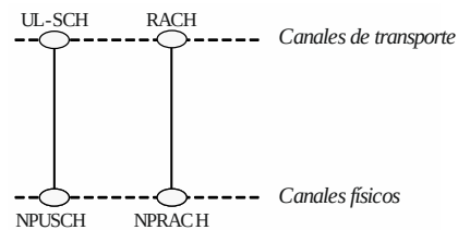
FIGURA 8 Configuración del canal NB-IoT ascendente
