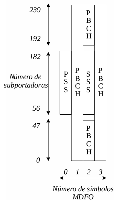
FIGURA 71 Estructura de tiempo-frecuencia del SSB
