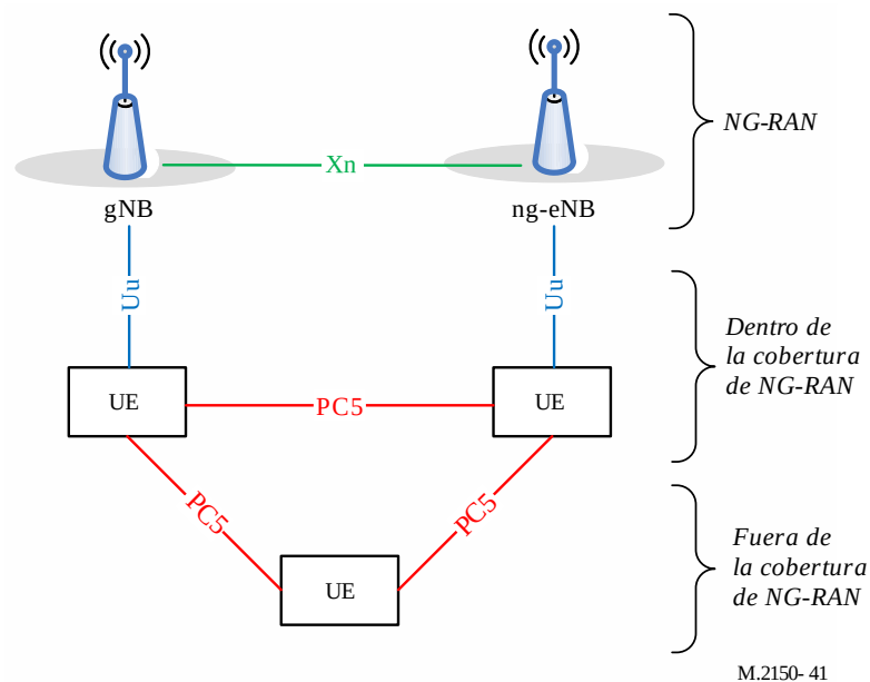
FIGURA 41 Arquitectura que soporta la interfaz PC5
