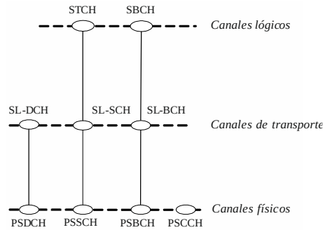
FIGURA 6 Configuración del canal lateral
