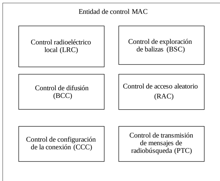
FIGURA 61 Entidad de control MAC
