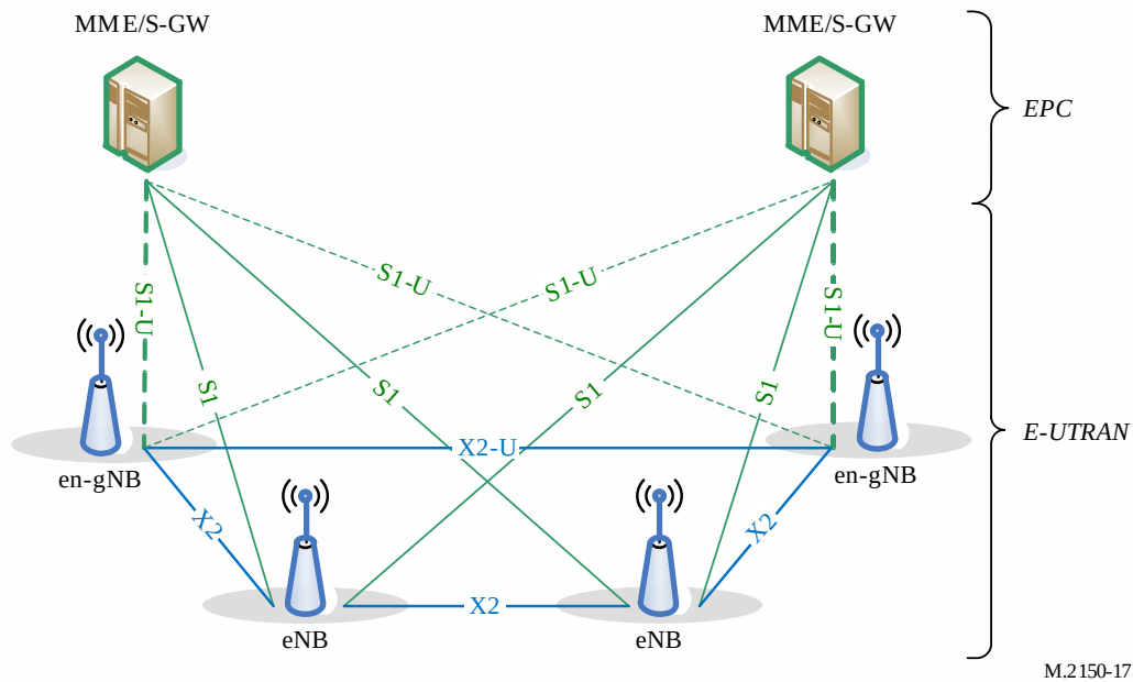
图17 EN-DC总体架构
