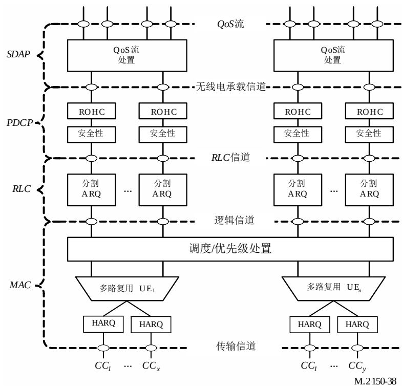
配置了CA的DL的第2层结构
