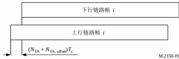
上行链路-下行链路定时关系
