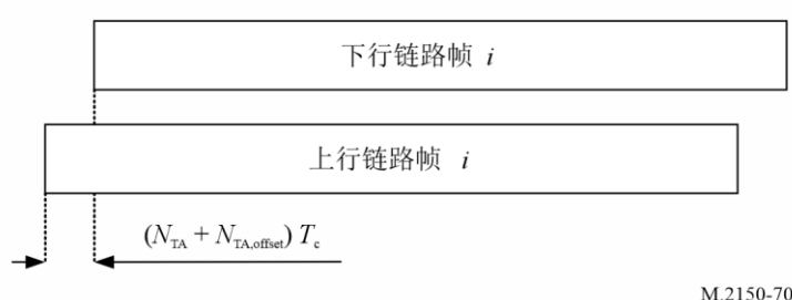
图70 上行链路的时间关系
