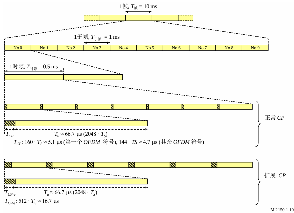
E-UTRA/LTE RIT的时域结构
