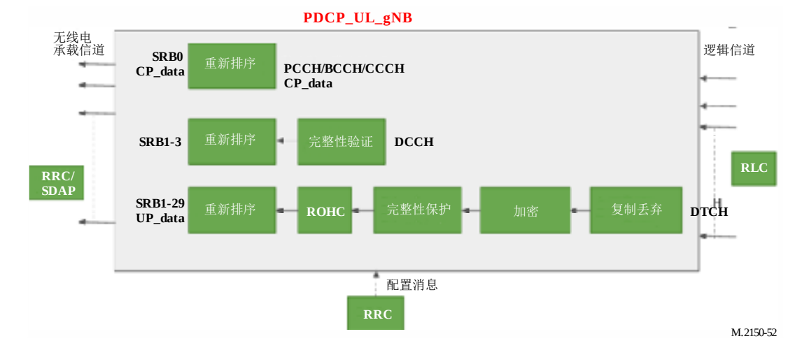
PDCP的上行链路架构
