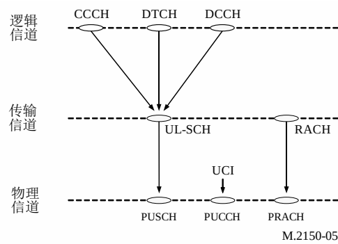
图6 侧链路信道映射
