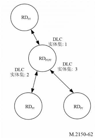
图62 在FT和PT模式下运行的RD的DLC实体集
