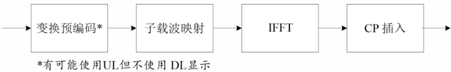
带可选DFT扩频的CP-OFDM发射机框图
