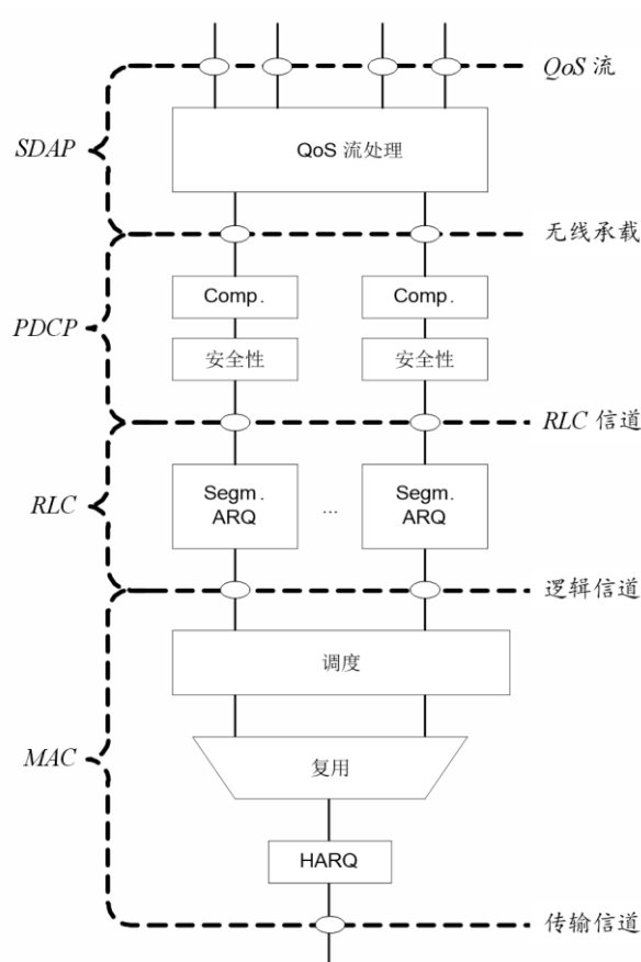
上行链路第2层的结构
