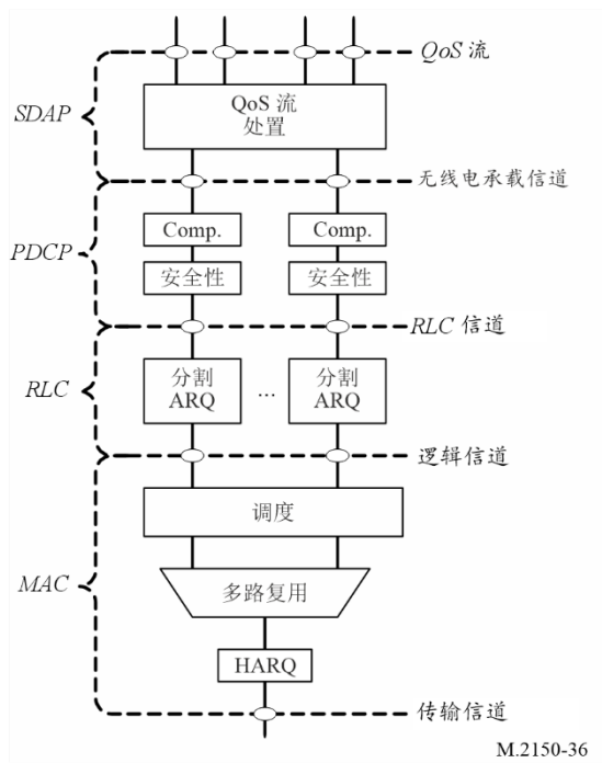
上行链路第2层结构
