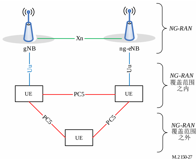
支持PC5接口的NG-RAN架构
