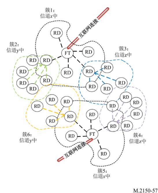
多FT场景中簇的形成示例
