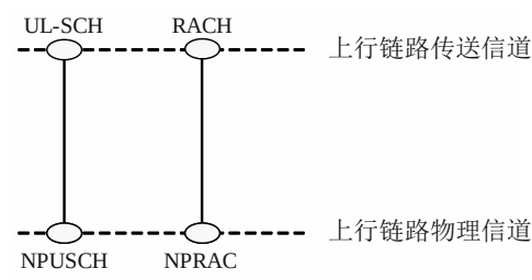
图8 NB-IoT UL信道映射
