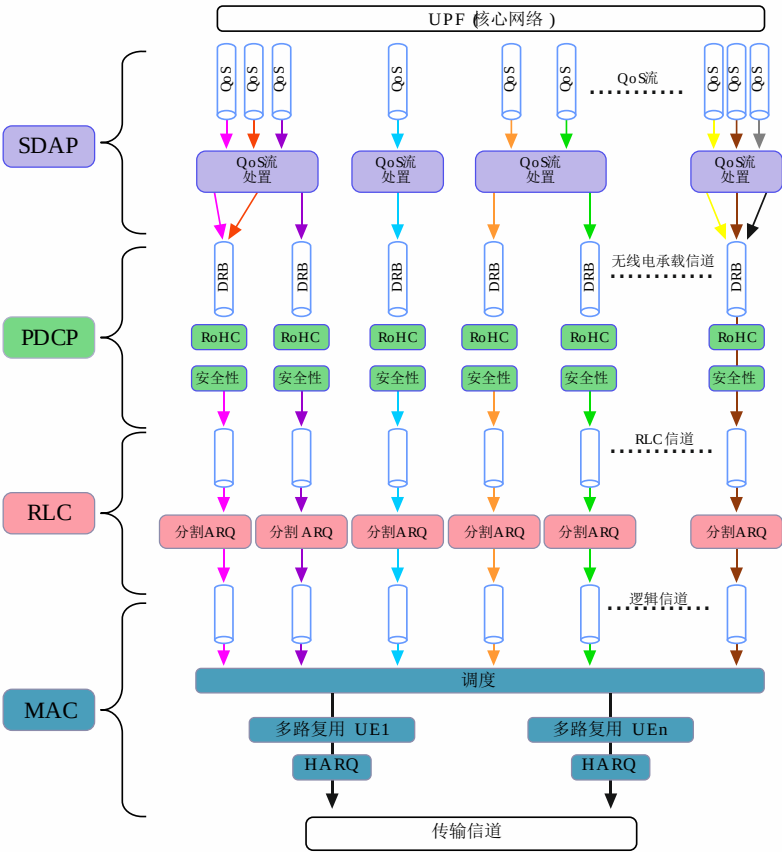
第2层的下行链路用户平面架构
