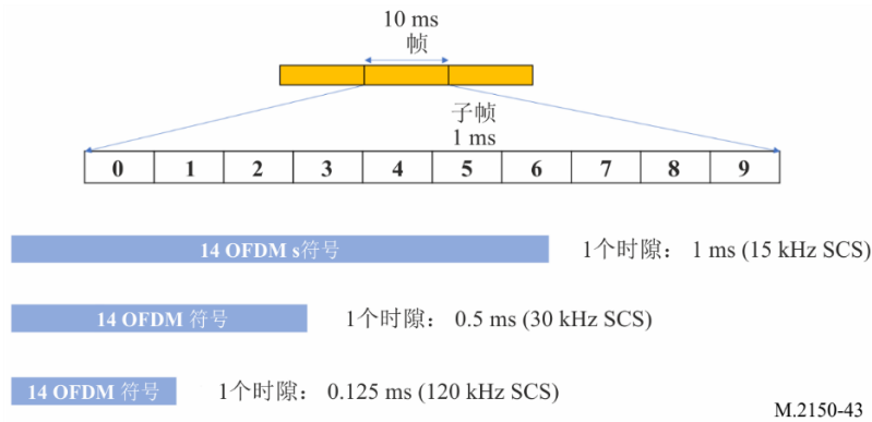
时域中的帧结构
