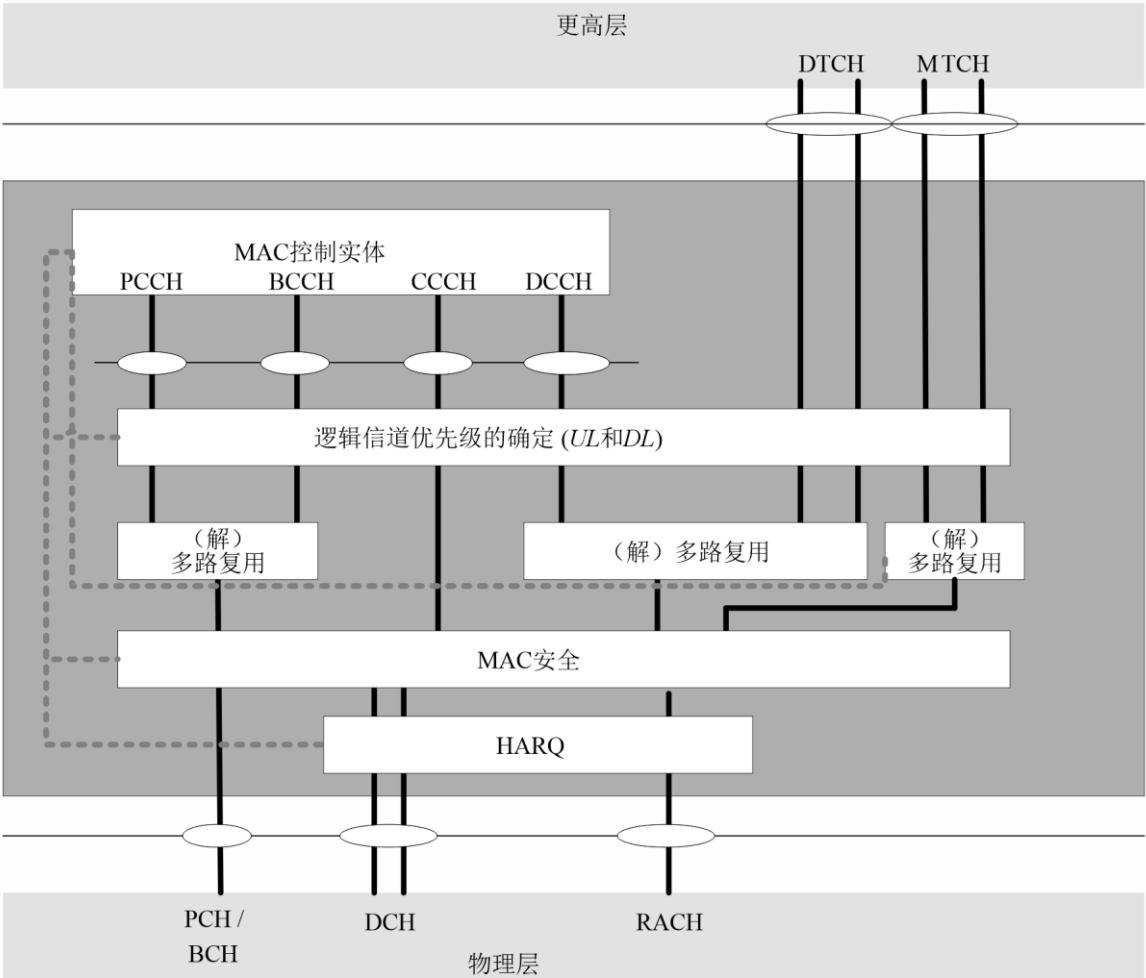
图60 MAC结构概述
