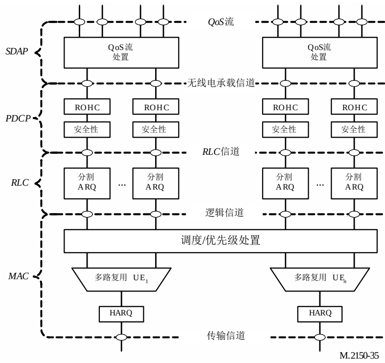
下行链路第2层结构
