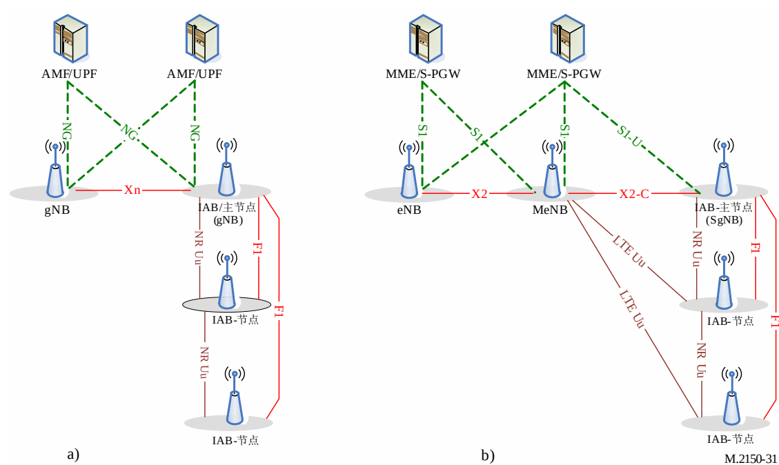
IAB架构；a) 使用5GCN的SA模式的IAB节点；b) 使用EN-DC的IAB节点
