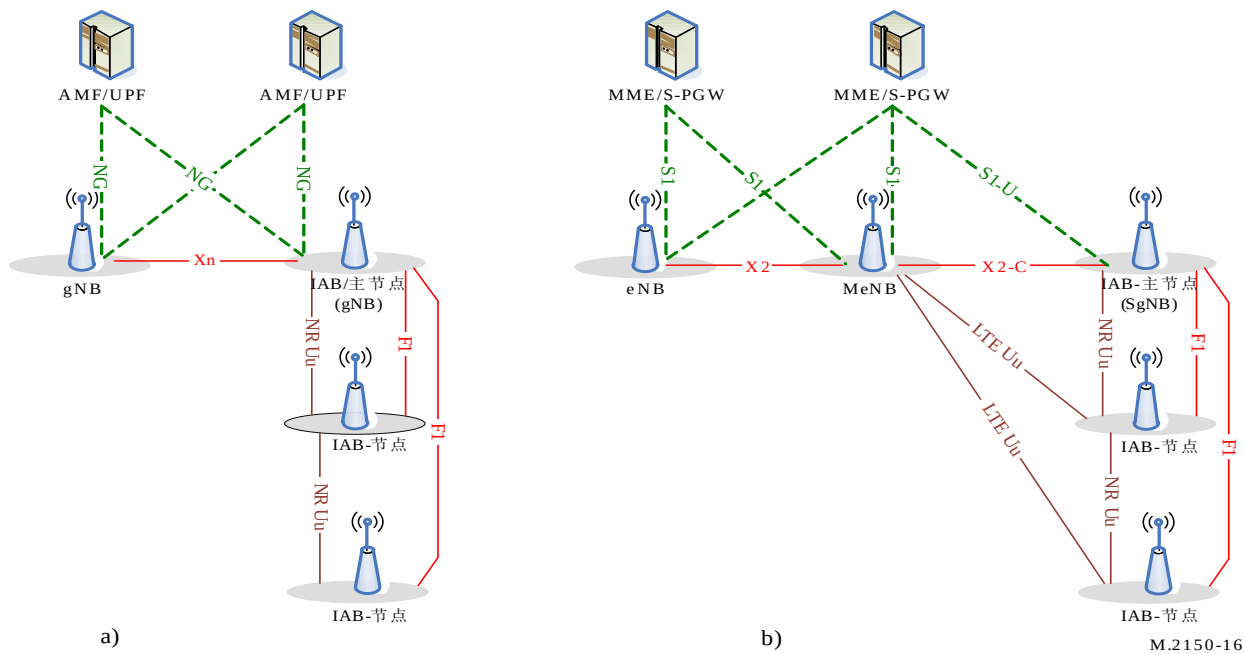
IAB架构：a) 使用5GCN的SA模式的IAB节点；b) 使用EN-DC的IAB节点
