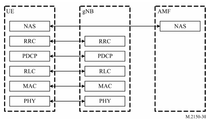
控制平面协议栈
