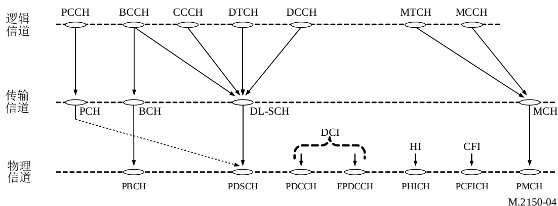
下行链路信道映射
