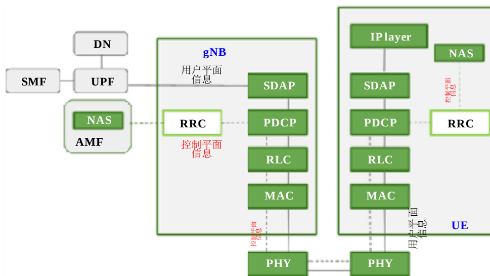
TSDSI RIT逻辑层的架构
