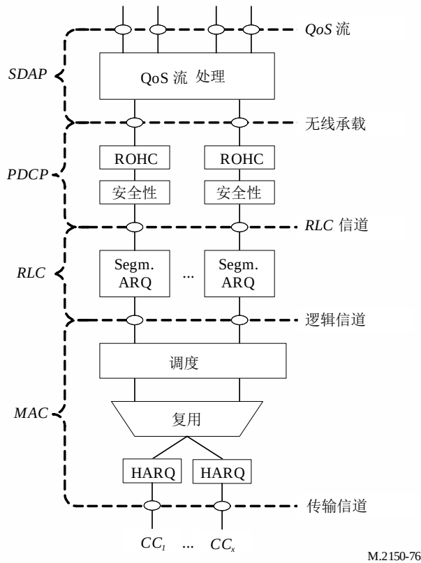
配置了CA的UL第2层结构
