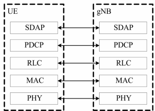
图66 用户平面协议栈
