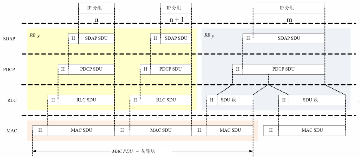
图74 数据流示例
