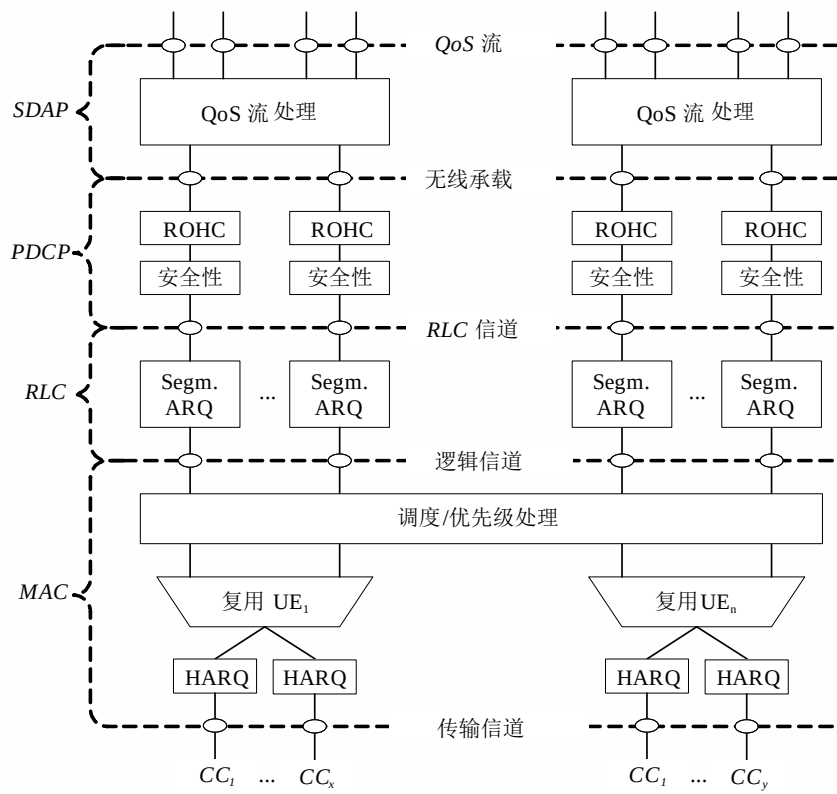
图75 配置了CA的DL第2层结构
