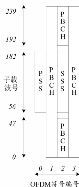
SSB的时频结构
