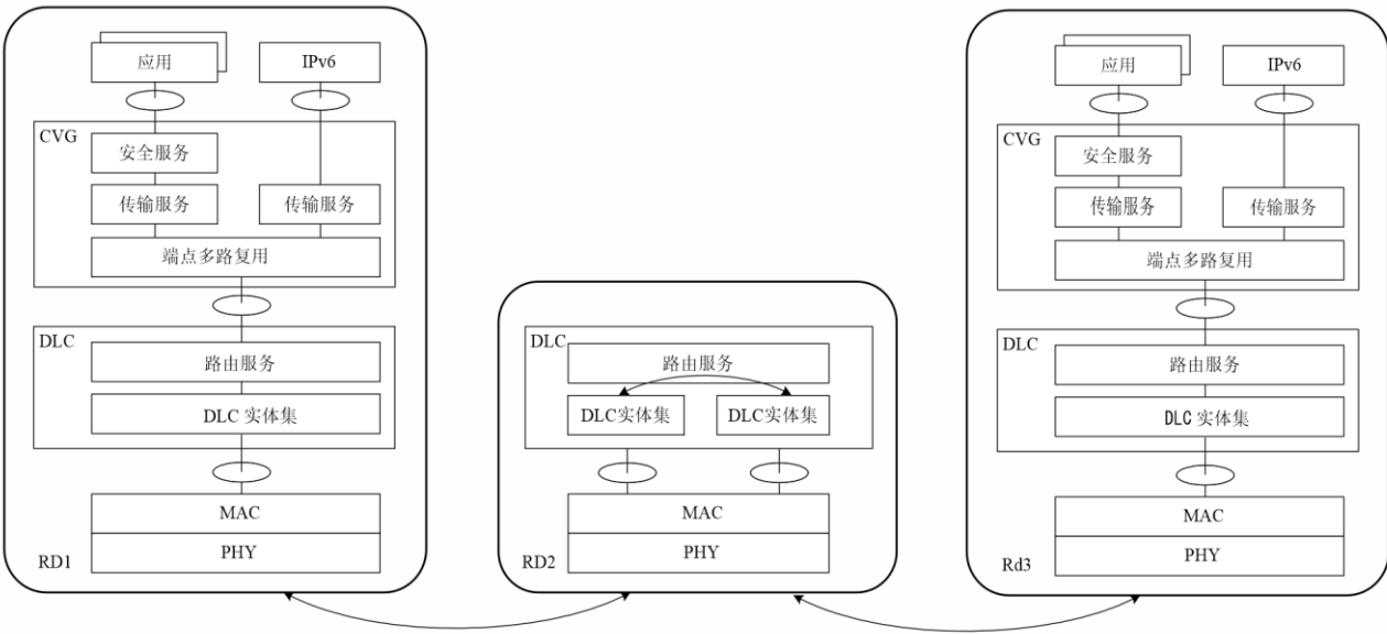
图59 整体协议架构的图示
