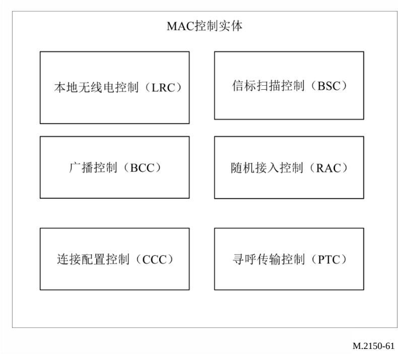
MAC控制实体
