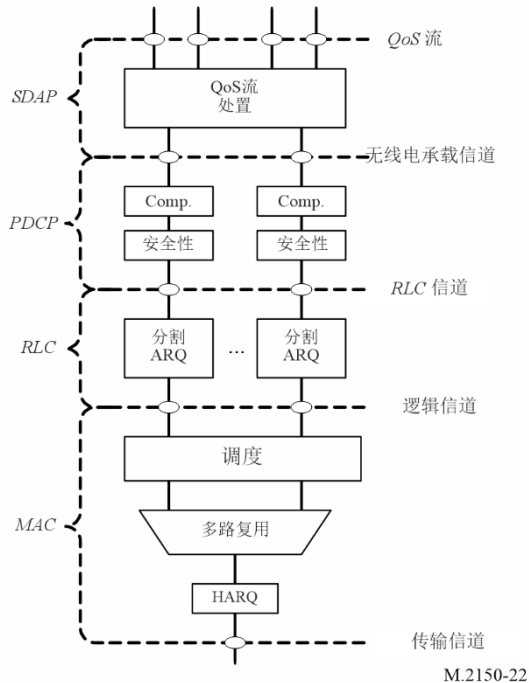
上行链路第2层结构
