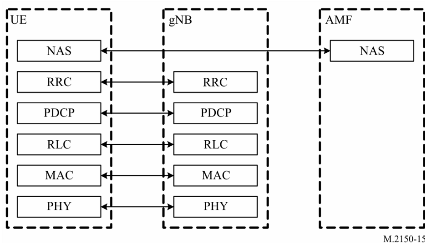
控制平面协议栈
