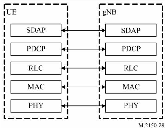
图29 用户平面协议栈
