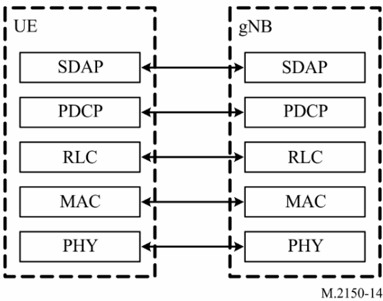
图14 用户平面协议栈
