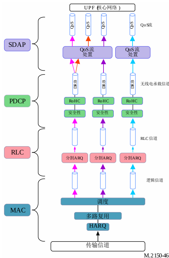
第2层的上行链路用户平面架构
