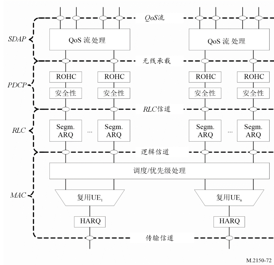
下行链路第2层的结构
