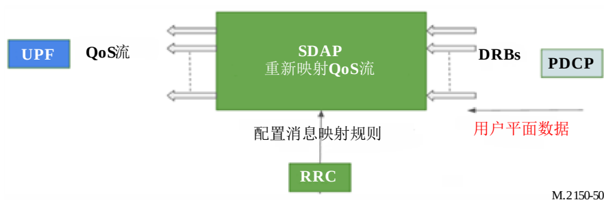
SDAP上行链路架构
