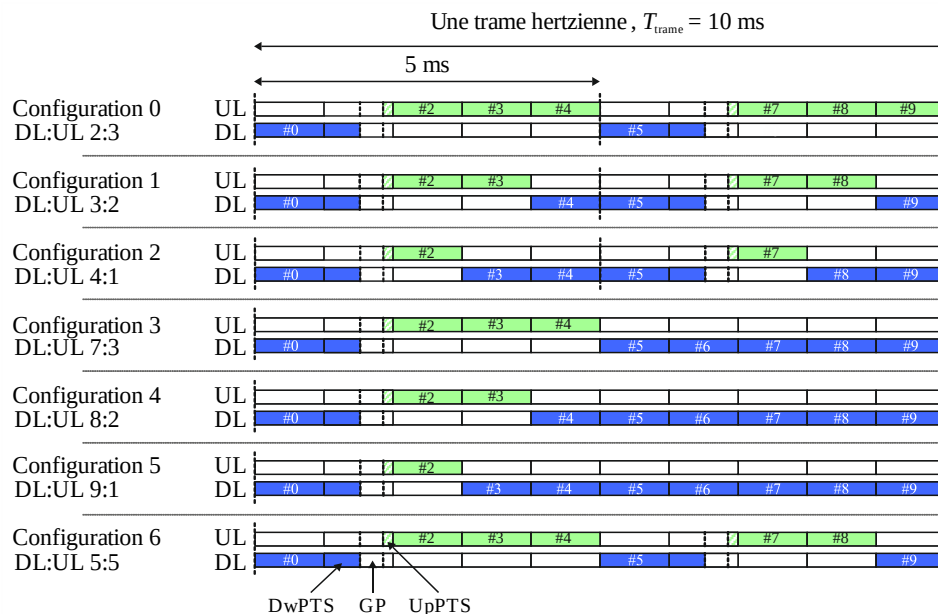
FIGURE 12 Attributions asymétriques entre liaisons montante et descendante que permet le système RIT DRT
