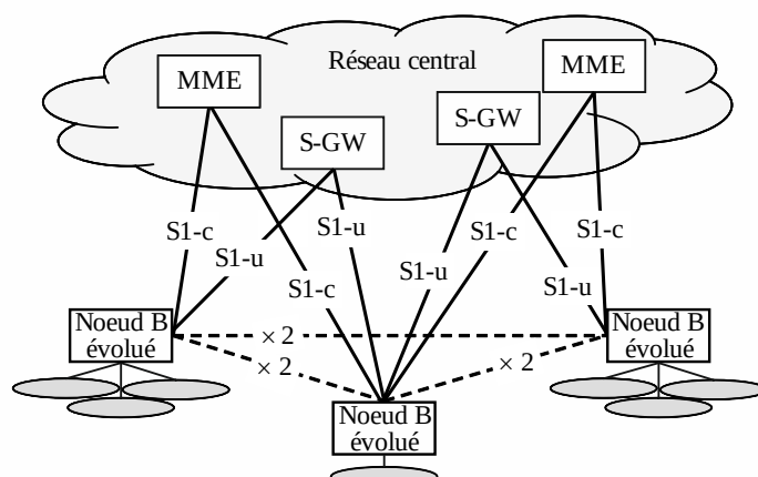
FIGURE 1 Interfaces des réseaux d'accès radioélectrique
