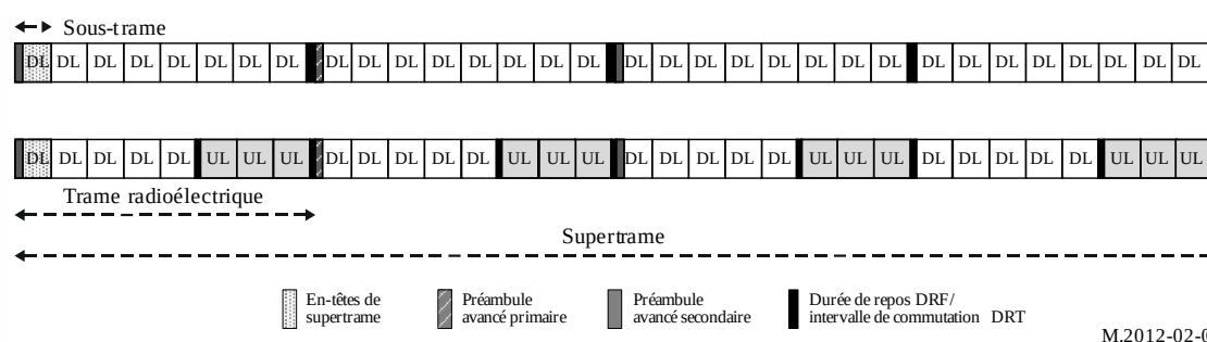
FIGURE 18 Structure des préambules évolués
