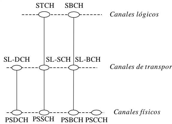
FIGURA 1.6 Configuración del canal lateral
