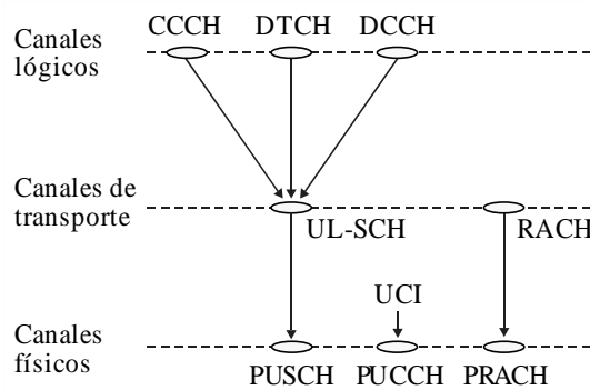
FIGURA 1.5 Configuración del canal ascendente
