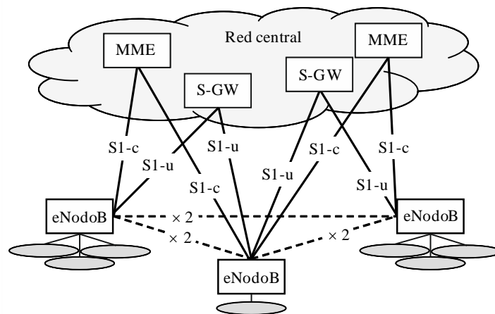
Interfaces de la red de acceso radioeléctrico
