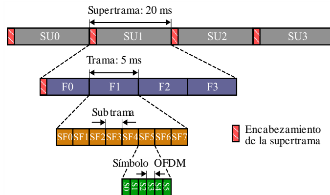
Estructura de la trama básica
