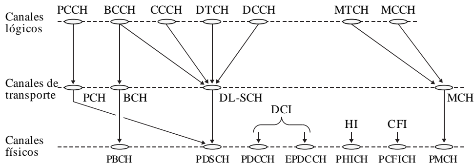
FIGURA 1.4 Configuración del canal descendente
