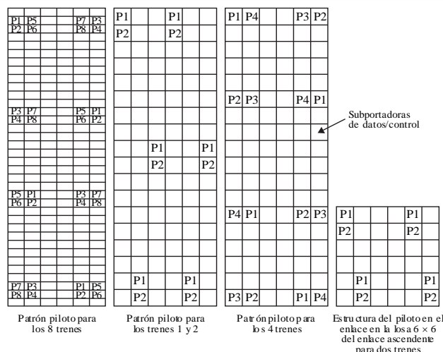
FIGURA 2.4 Estructura de piloto para los flujos 1, 2, 4 y 8 de la subtrama tipo 1
