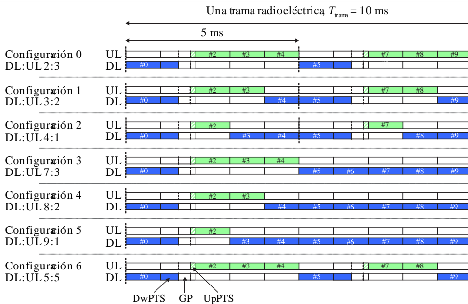
FIGURA 1.10 Asimetría de los enlaces ascendente y descendente soportada por la RIT TDD
