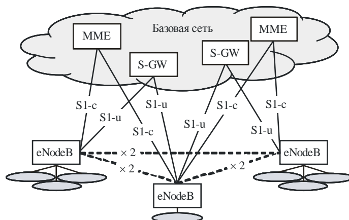
РИСУНОК 1.1 Интерфейсы сети радиодоступа
