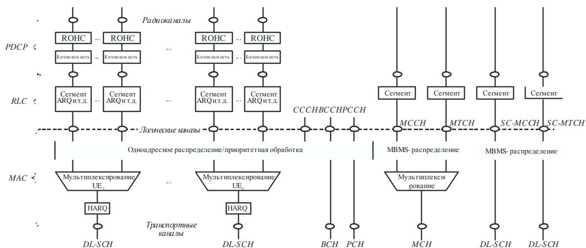
РИСУНОК 1.2 Структура протокола L2 на линии вниз
