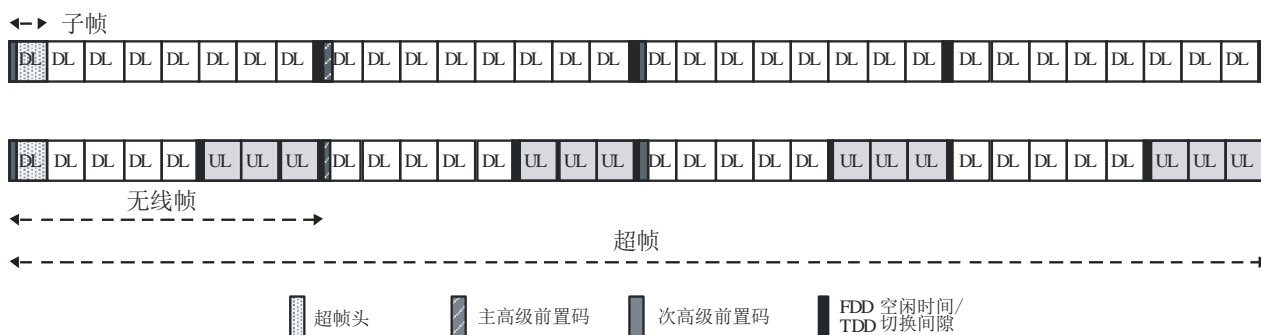
先进前置码的结构
