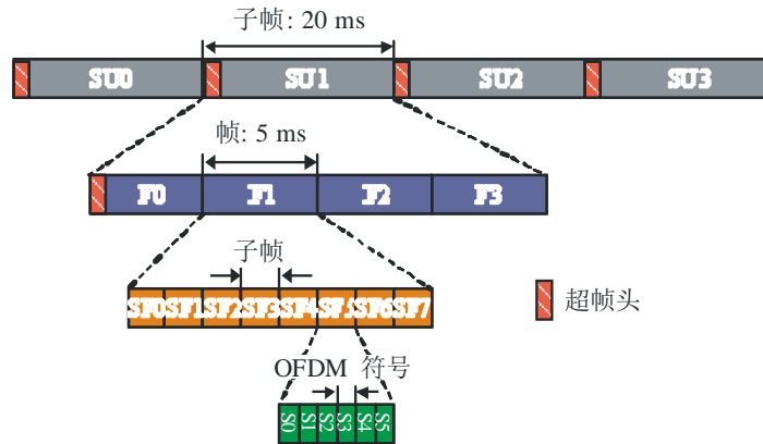
基本帧的结构
