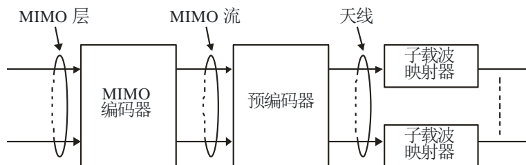
MIMO结构
