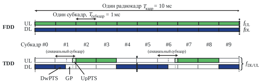
РИСУНОК 1.9 Частотно-временная структура для случаев FDD и TDD на линии вверх и линии вниз
