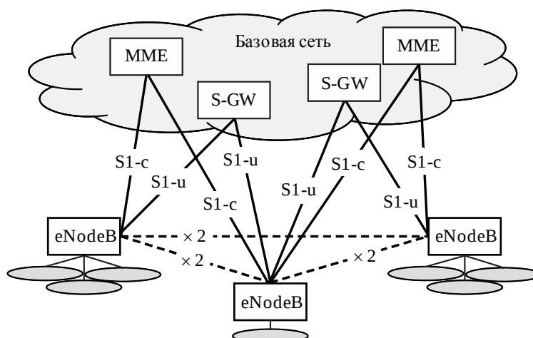
РИСУНОК 1.1 Интерфейсы сети радиодоступа
