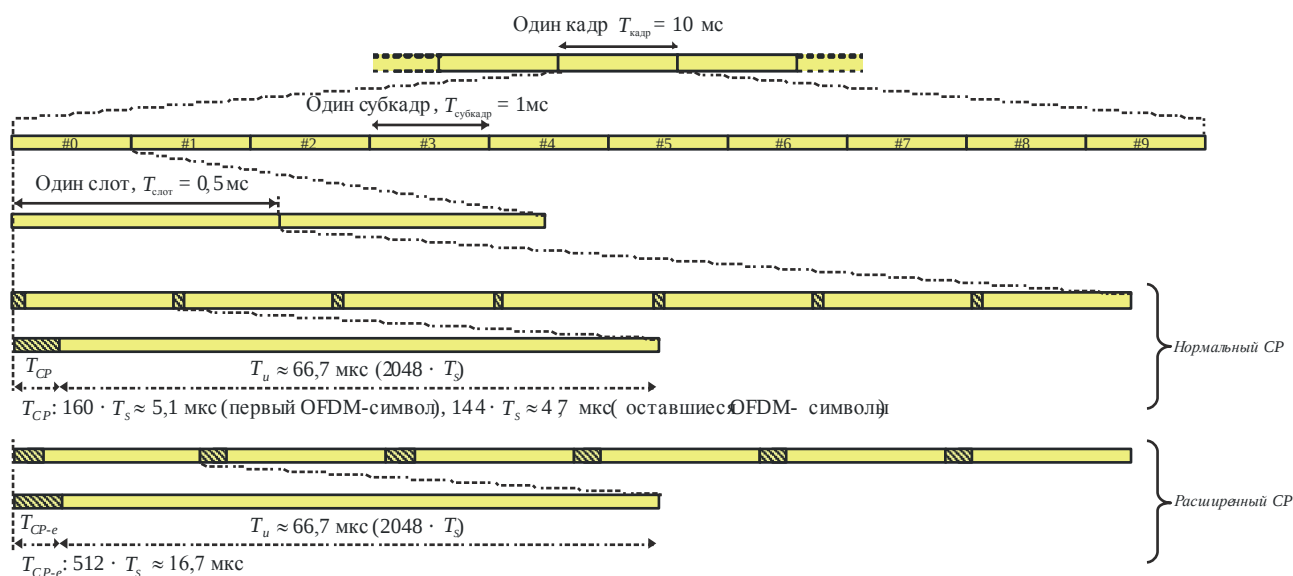
РИСУНОК 1.8 Временная структура LTE-Advanced
