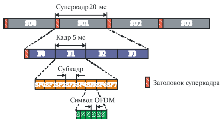
Базовая структура кадра
