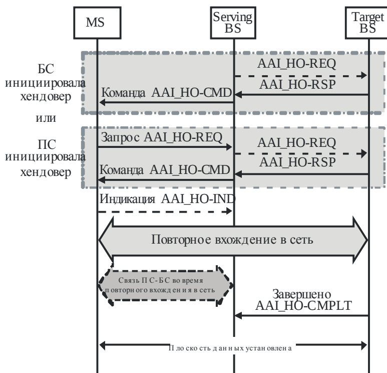
РИСУНОК 2.10 Процедуры хендовера
