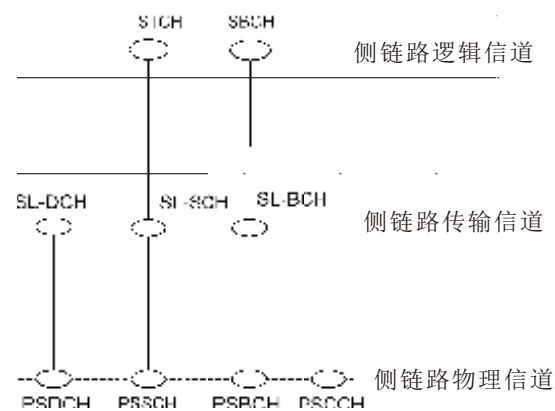
侧链路信道映射
