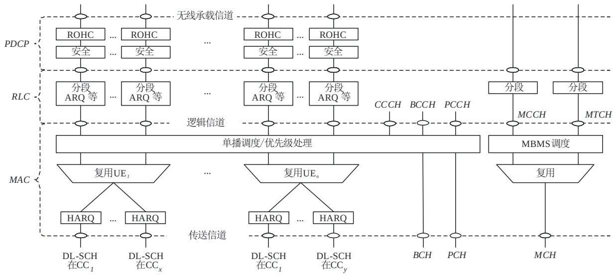
图1.2 下行链路L2协议的结构
