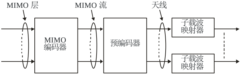
MIMO结构
