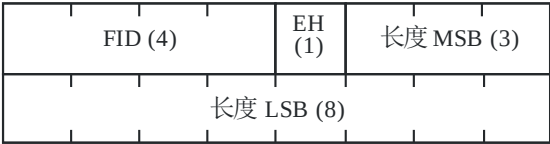
图2.9 先进通用MAC头
