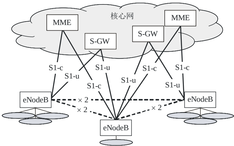
图1.1 无线接入网接口
