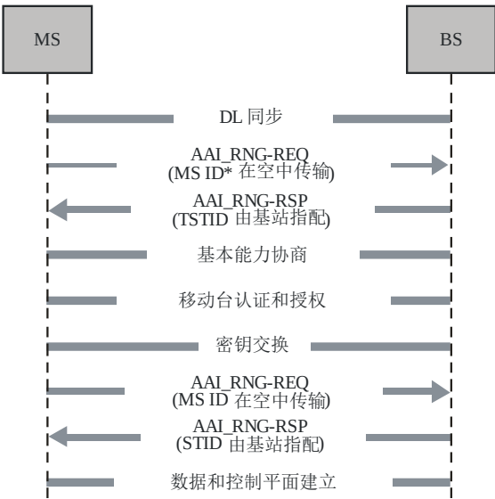
图2.8 网络登录程序
