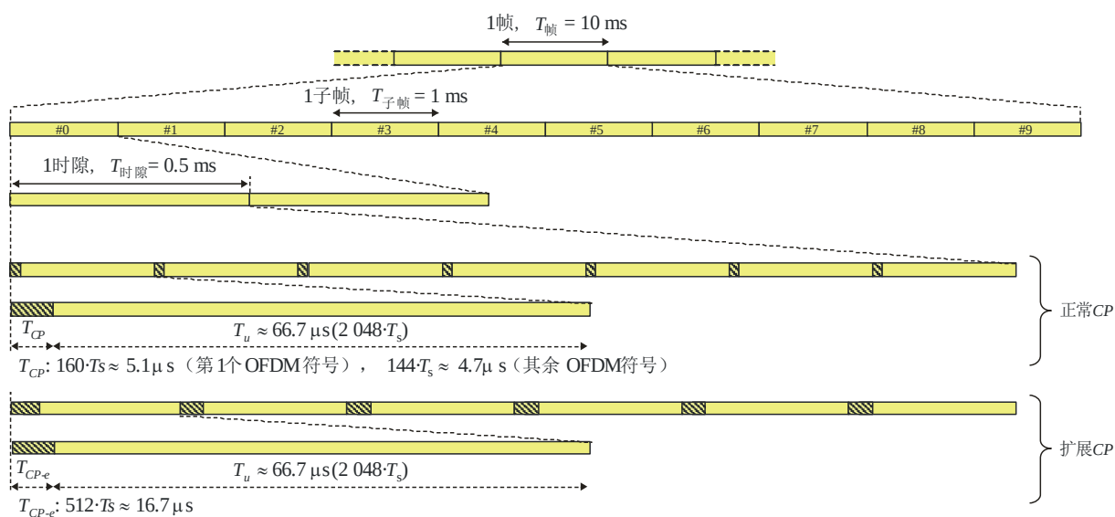
LTE-Advanced的时域结构
