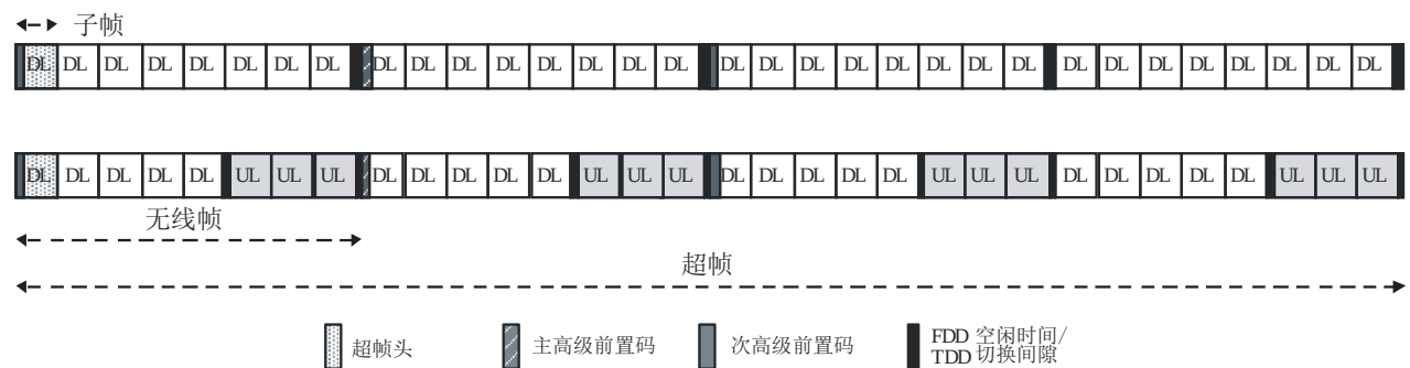
先进前置码的结构
