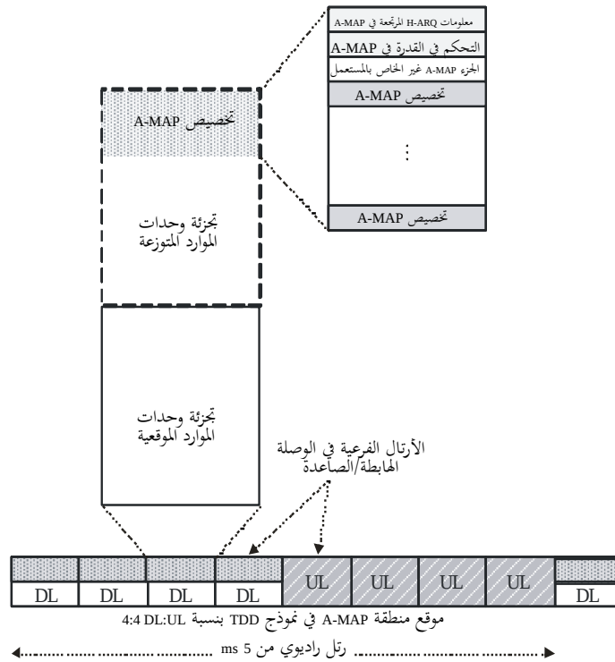
موقع وبنية جزء التطبيق المتنقل المتقدم A-MAP (مثال)
