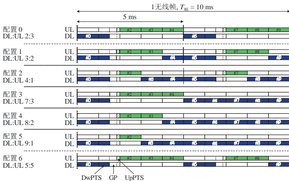
图1.9 由TDD RIT的支持上行一下行不对称性
