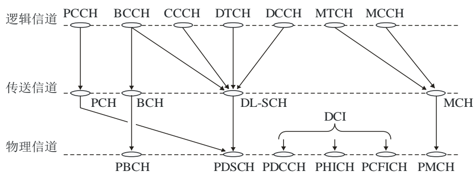
图1.4 下行信道映射
