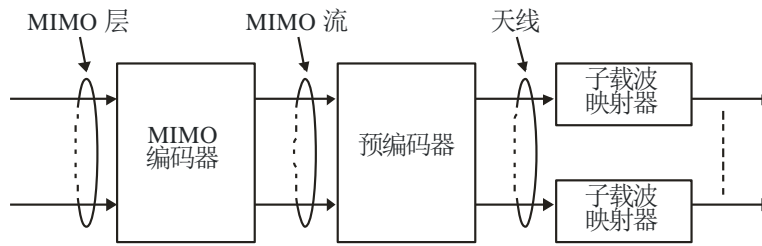
MIMO结构
