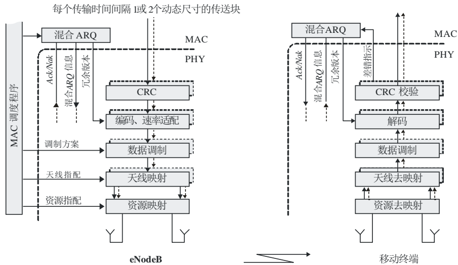
在一个分量载波上DL-SCH的简化物理层处理
