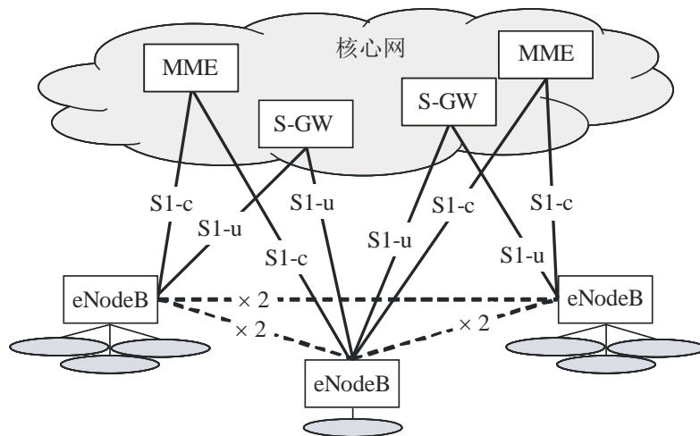
无线接入网接口
