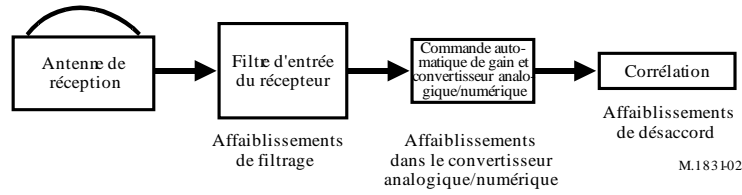
Modèle simplifié de récepteur d'utilisateur
