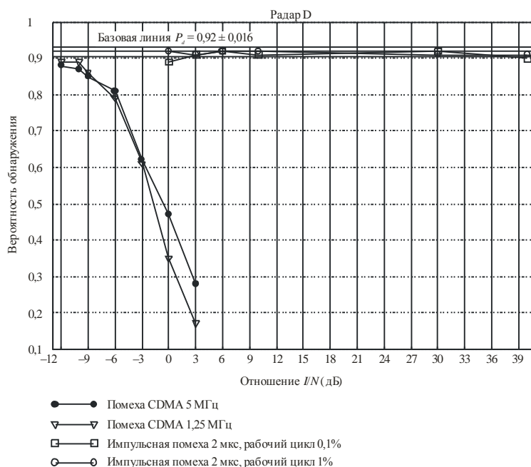
Кривые вероятности обнаружения для радара D
