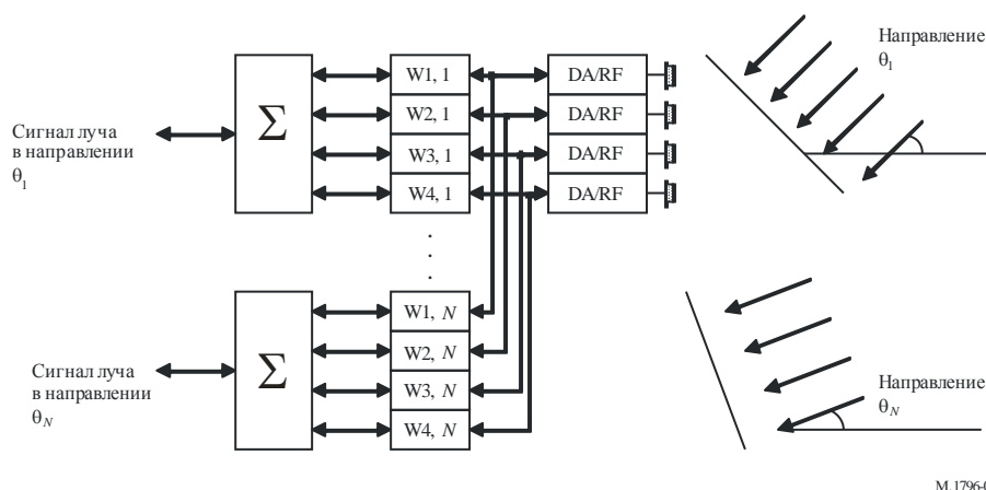
РИСУНОК 1 Многолучевая антенна
