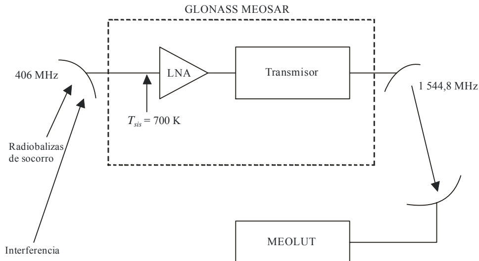
FIGURA 10 Repetidor GLONASS MEOSAR con interferencia en el enlace ascendente
