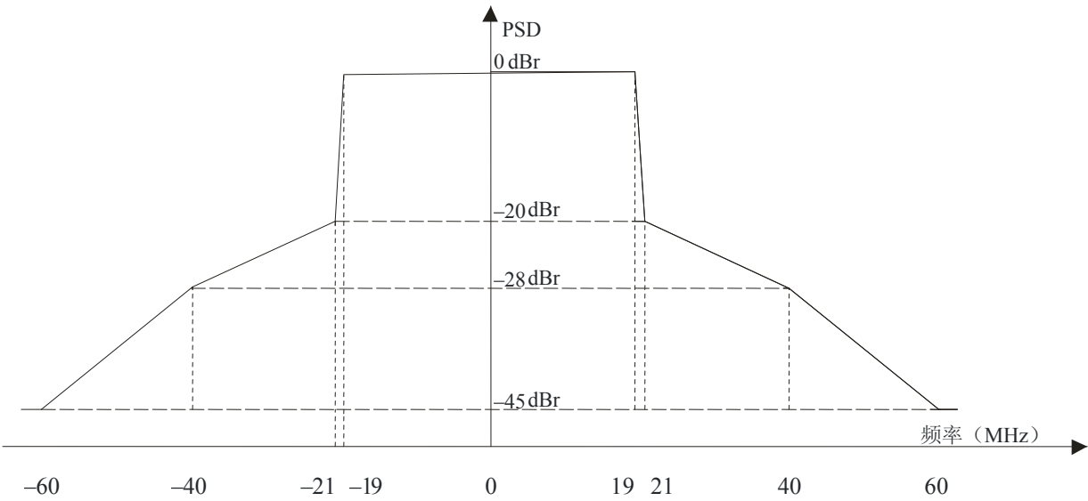
图 3 40 MHz的 802.11n频道的发射频谱掩模
