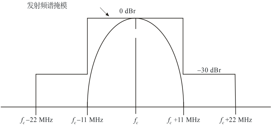
图 4 802.11b的发射频谱掩模
