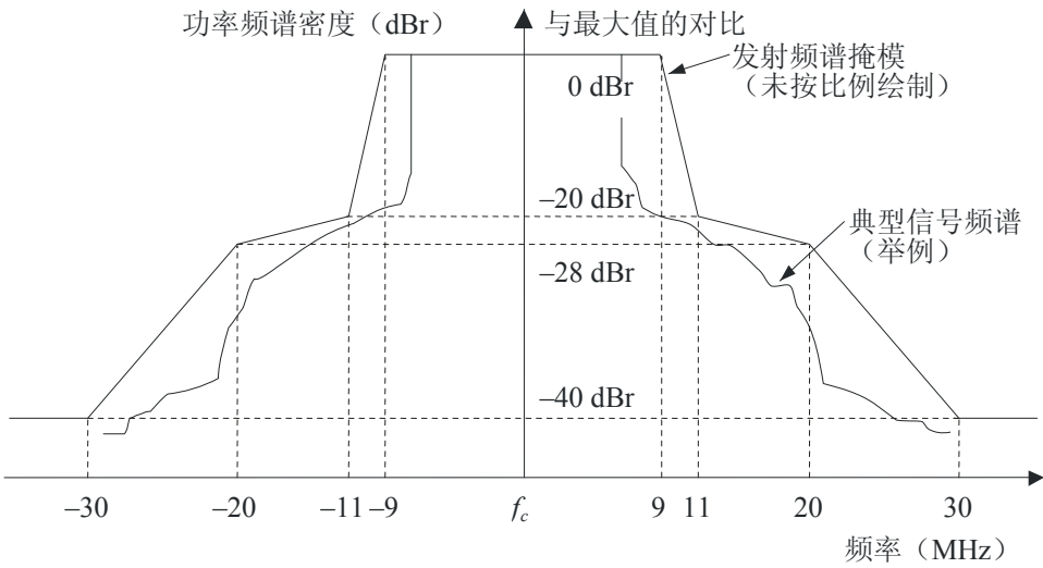
图 1 802.11a、11g、11j、HIPERLAN2和HiSWANa系统的 OFDM发射频谱掩模
