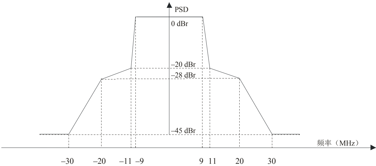
图 2 20 MHz 802.11n传输的发射频谱掩模
