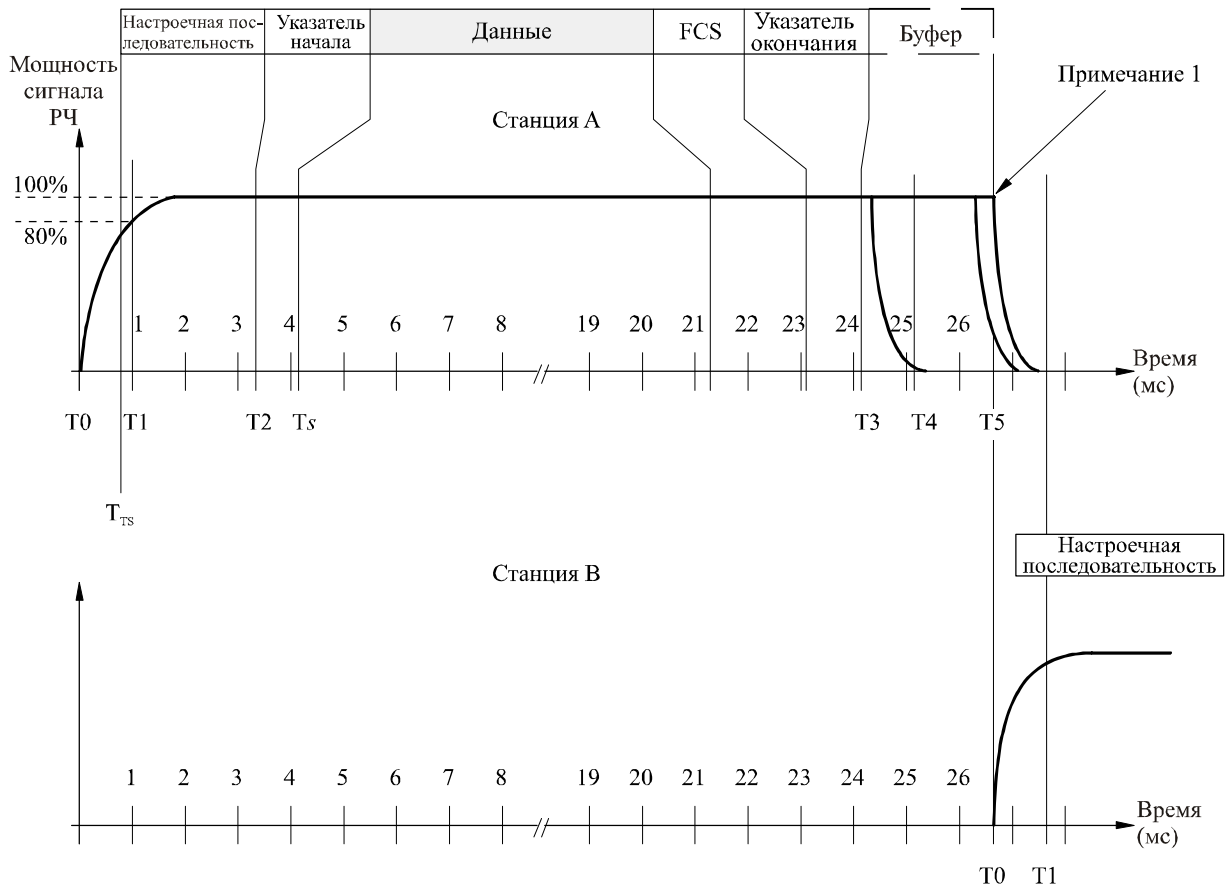
РИСУНОК 8 Временная диаграмма передачи
