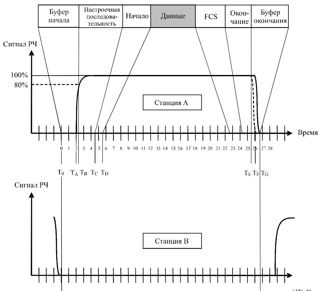
Временная диаграмма передачи
