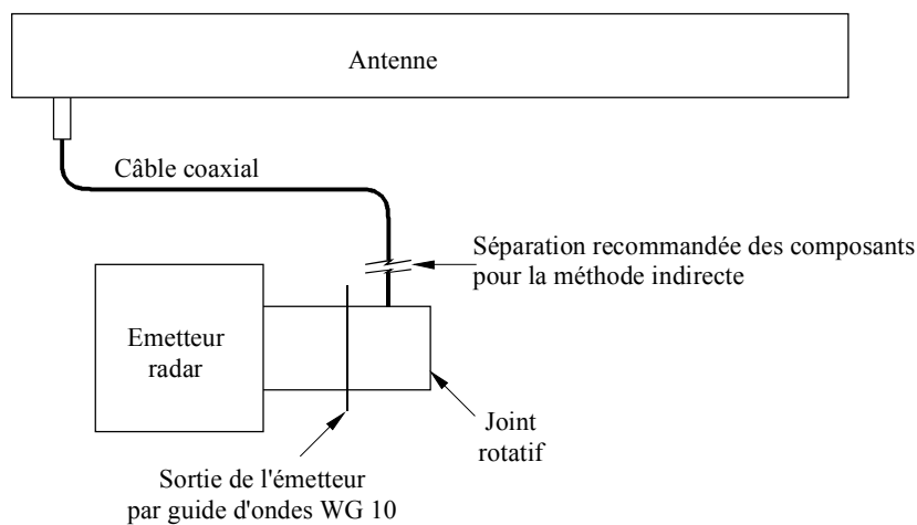
FIGURE 5 Système type de radar
