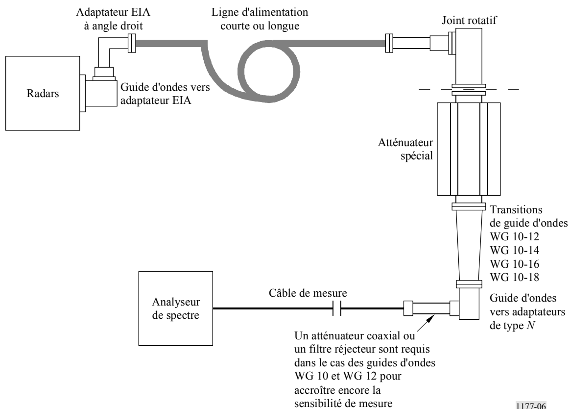
FIGURE 6 Mesure à l'accès du joint rotatif
