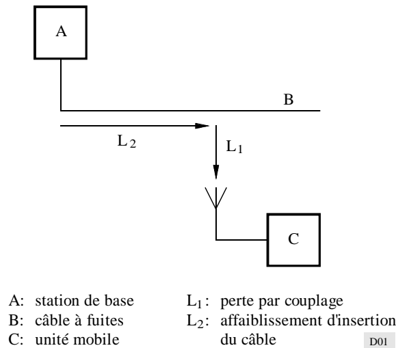
FIGURE 1 Système de base
