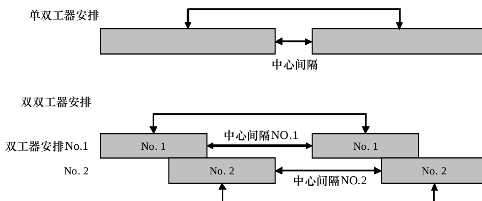
FDD 频率安排中的双双工安排
