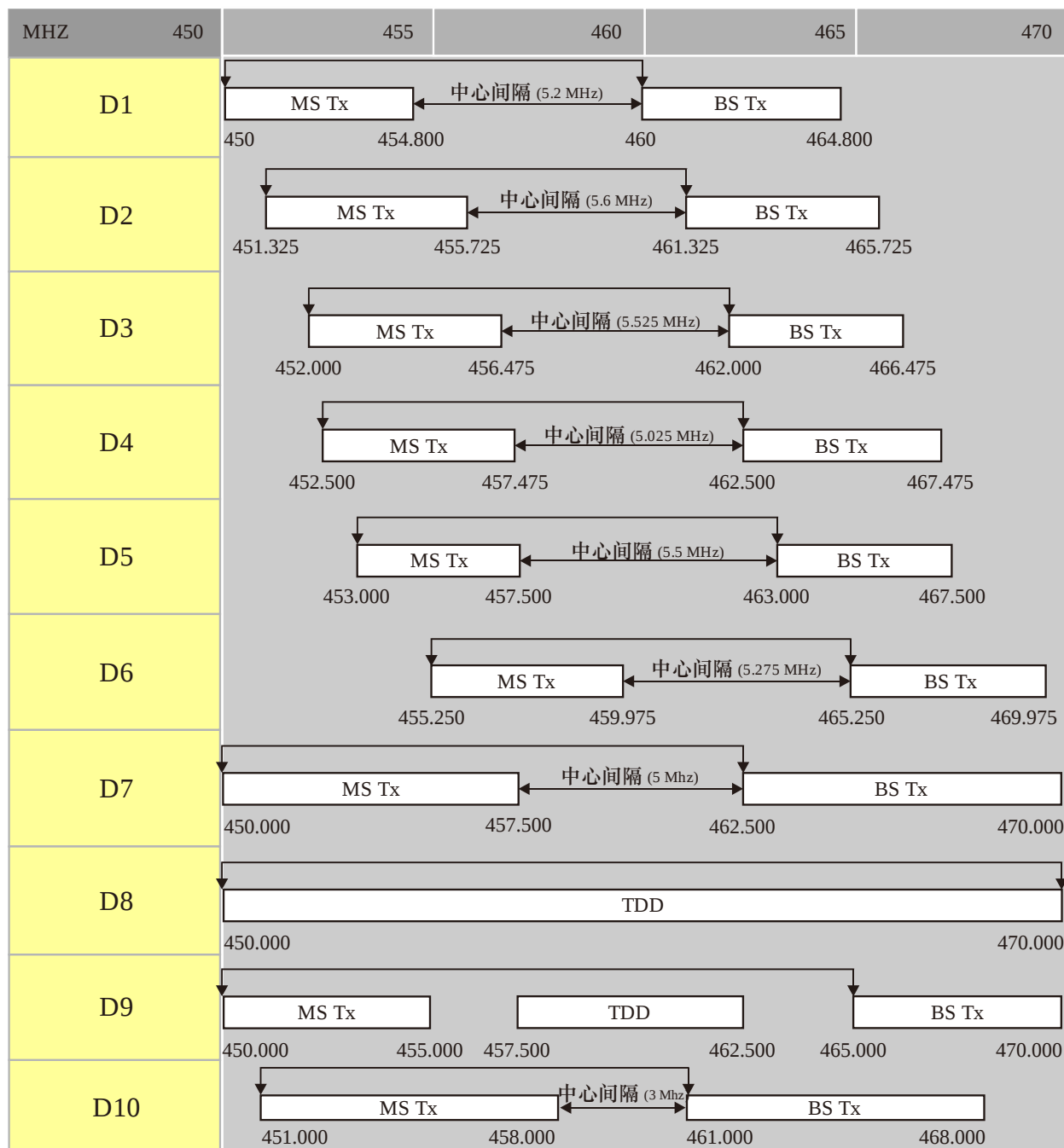
图2 中心间隔
