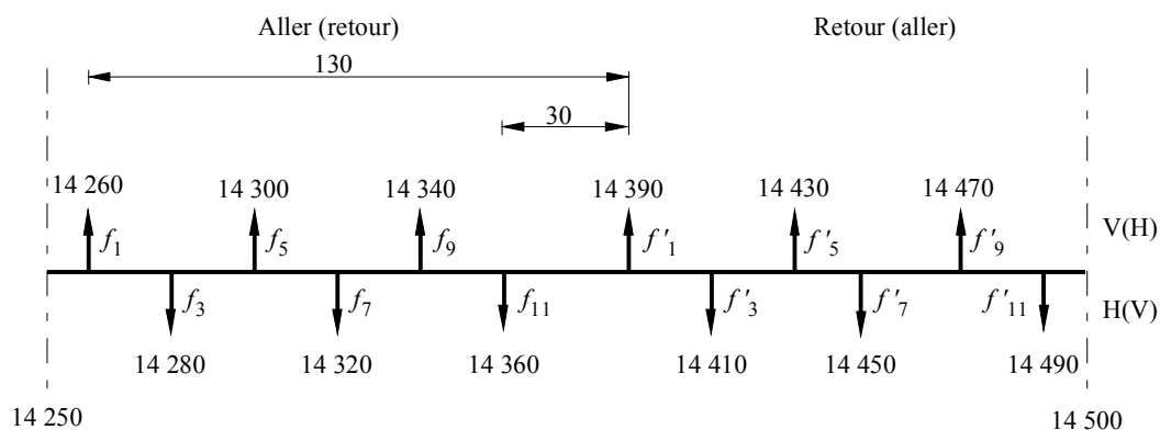
FIGURE 5 Disposition des canaux radioélectriques pour des FWS fonctionnant dans la bande des 14 GHz avec un espacement de 20 MHz (Fréquences en MHz)
