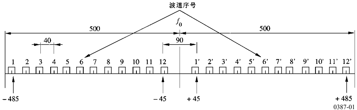
图1 按照做出建议1.1工作于11 GHz频带的高容量 固定无线系统的射频波道配置 (所有频率单位为 MHz)
