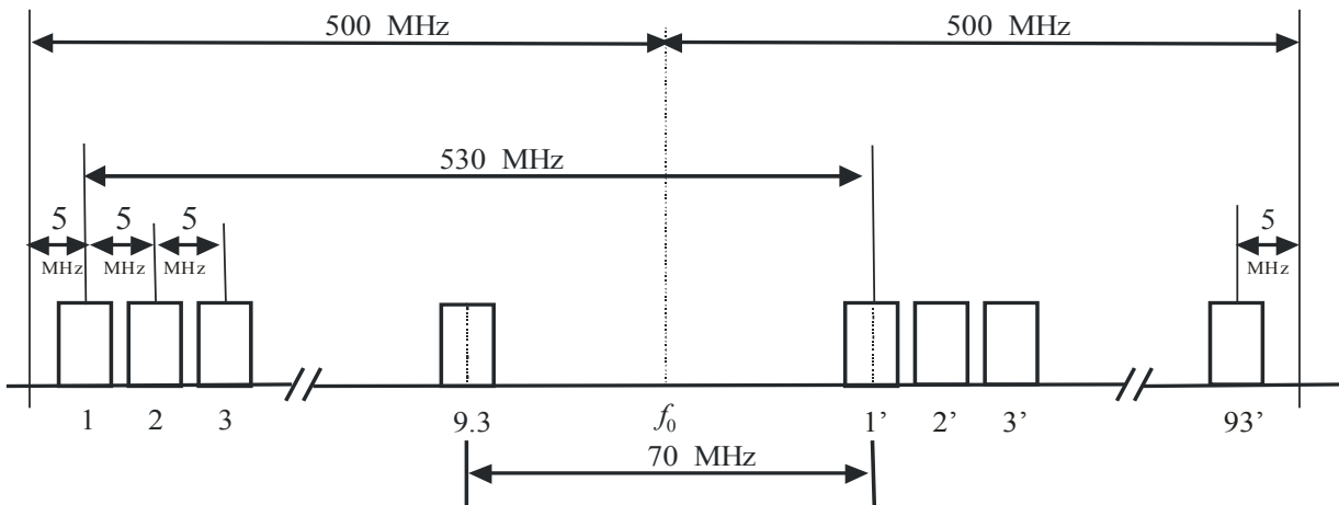
c) 载波间隔为 5 MHz 的系统
