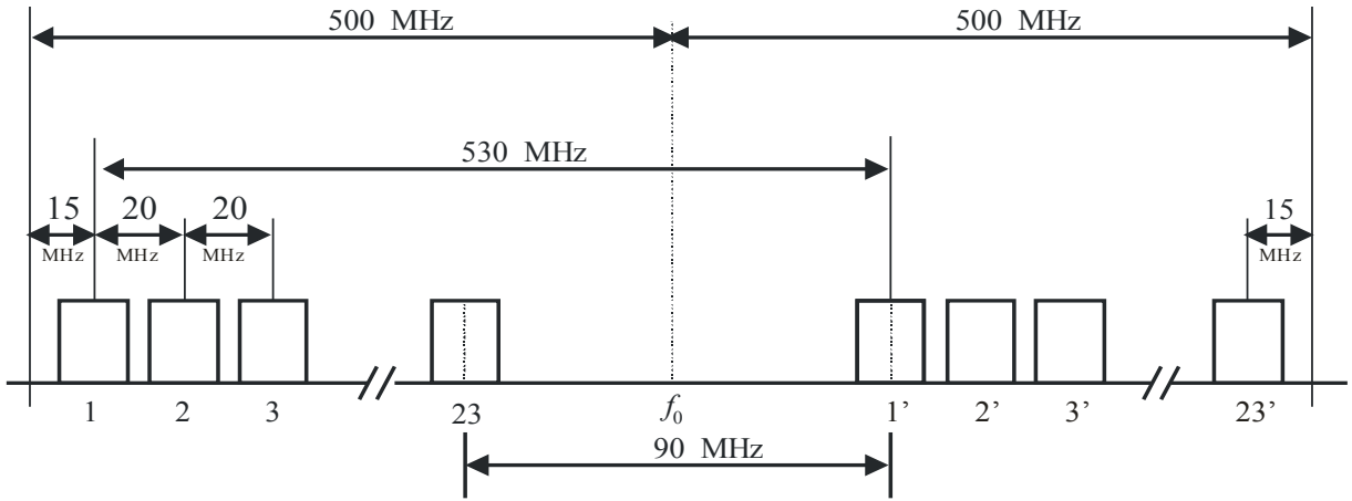
a) 载波间隔为 20 MHz 的系统
