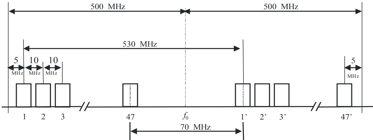
b) 载波间隔为 10 MHz 的系统
