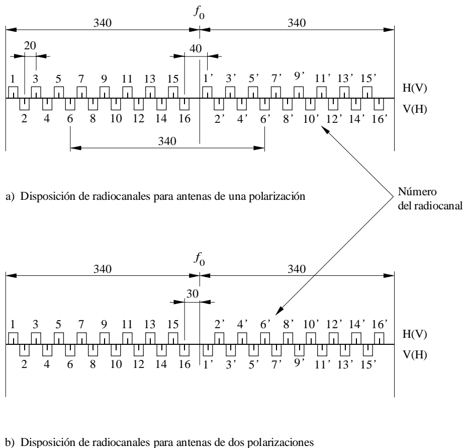
FIGURA 2 Disposición de radiocanales para antenas de una y dos polarizaciones (Todas las frecuencias en MHz)
