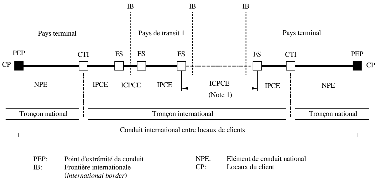
Configuration conceptuelle des éléments d'un conduit international entre locaux de clients
