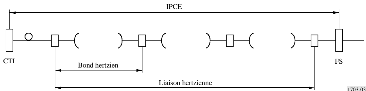
FIGURE 3 Exemple de liaison hertzienne comprenant un tronçon d'élément IPCE
