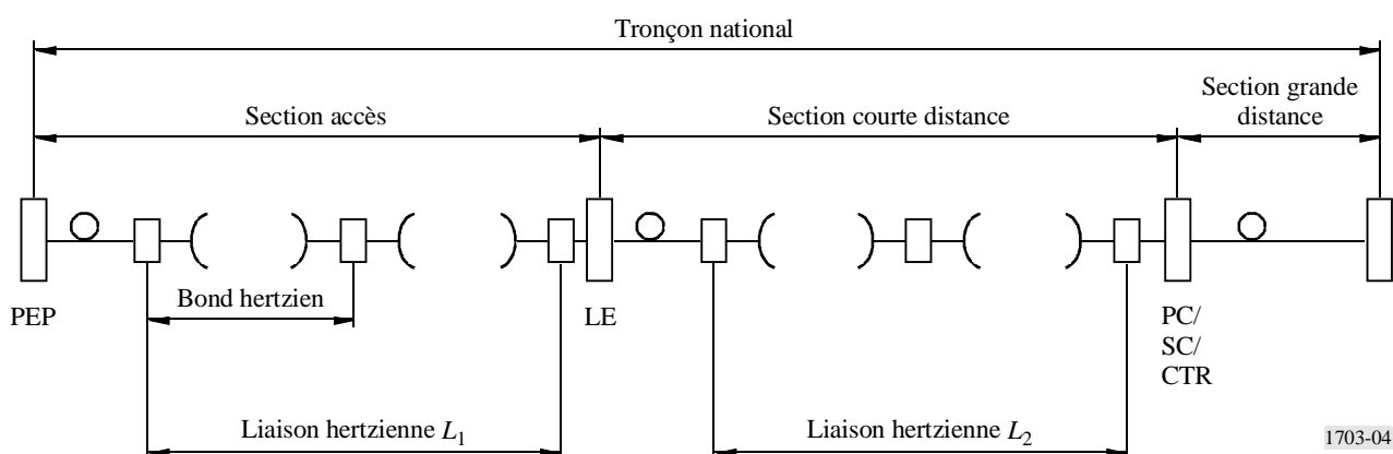
FIGURE 4 Exemple de liaisons hertziennes utilisées dans la section accès et dans la section courte distance d'un élément NPE
