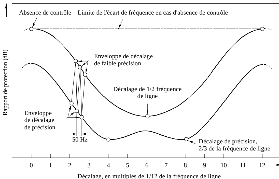
Courbes schématiques du rapport de protection pour différentes positions de décalage
