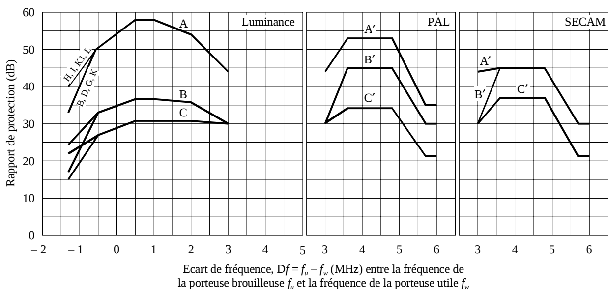
FIGURE 3 et TABLEAU 12 Systèmes à 625 lignes – Brouillage continu
