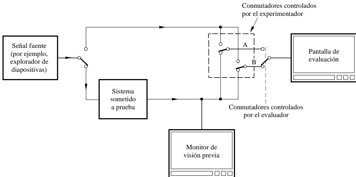
Disposición general del sistema de prueba para el método DSCQS
