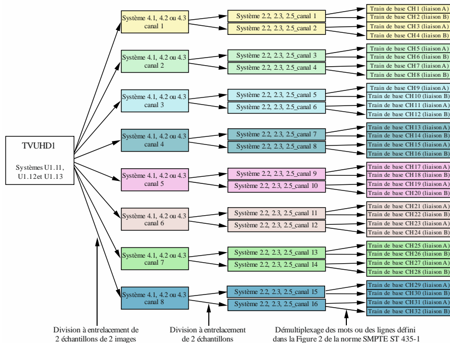
Division en 32 pour les systèmes U1.11, U1.12 et U1.13
