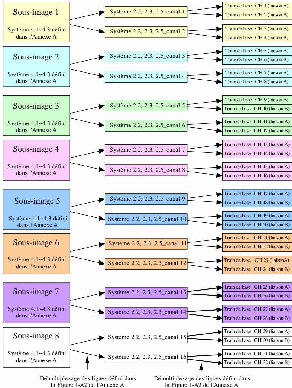
FIGURE 1-7 Division en 32 pour les systèmes U1.11, U1.12 et U1.13
