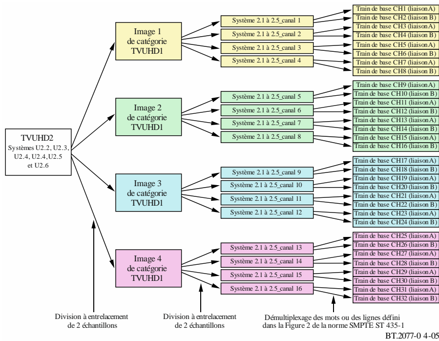
Division en 16 pour les systèmes U2.2, U2.3, U2.4, U2.4, U2.5 et U2.6
