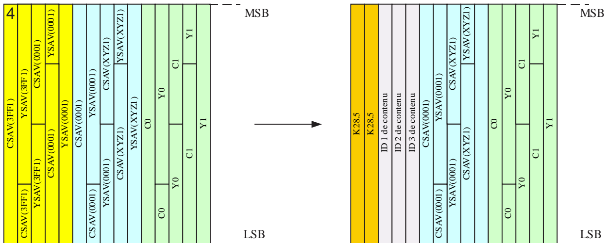
Remplacement de données SAV dans le canal CH1
