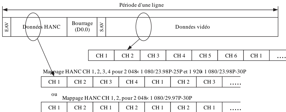
Structure d'alignement des données pour le train en mode B
