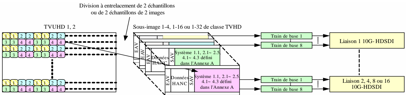
FIGURE 1-1 Aperçu du mappage pour la TVUHD
