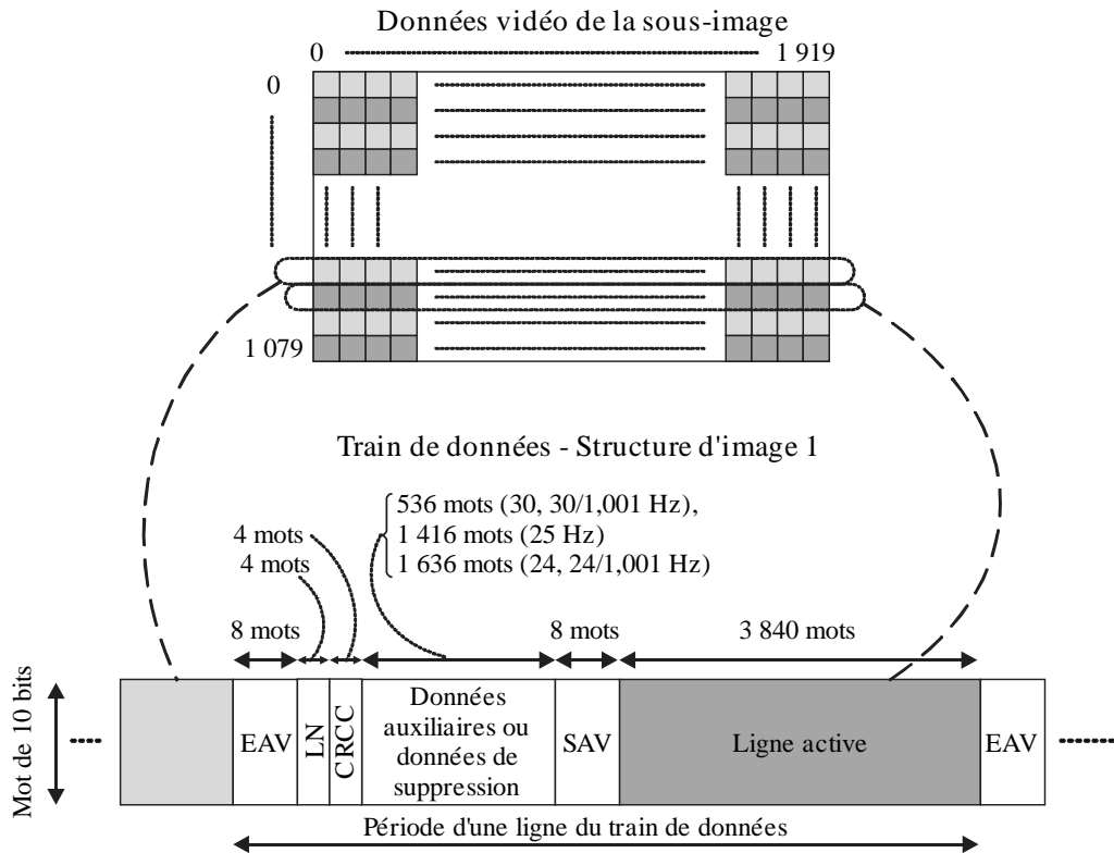
FIGURE 3-8 Structure de ligne de chaque train de données pour les fréquences d'image de 30 Hz, 30/1,001 Hz, 25 Hz, 24 Hz et 24/1,001 Hz – Structure d'image 1
