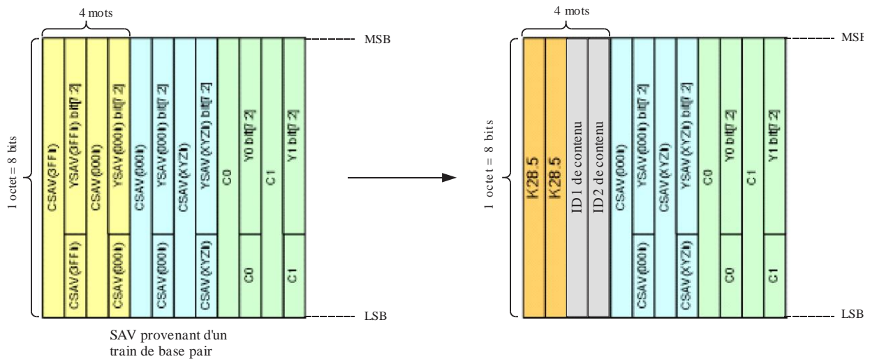
FIGURE 1-25 Remplacement de données SAV dans le canal CH2
