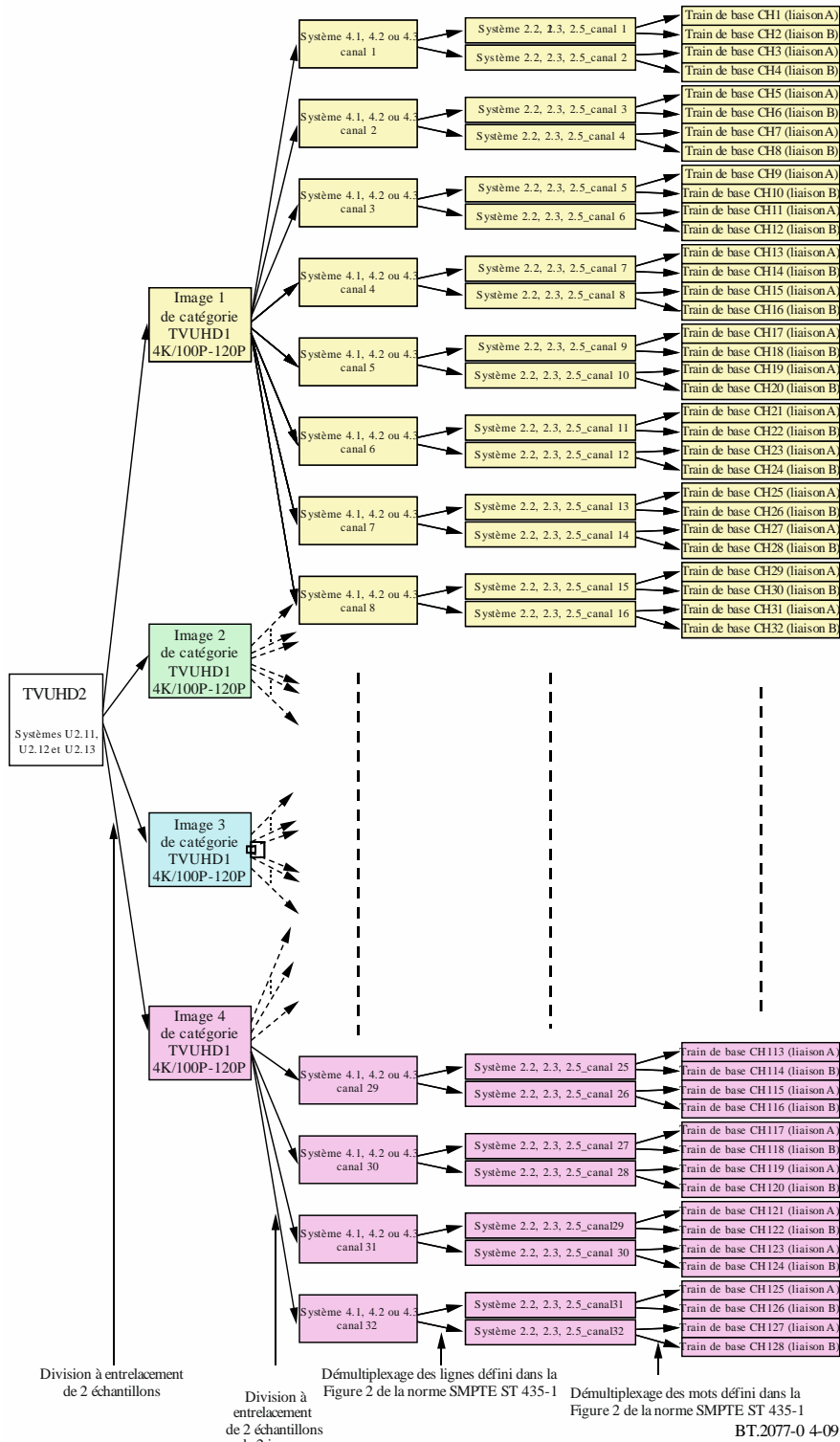
Division en 128 pour les systèmes U2.11, U2.12 et U2.13
