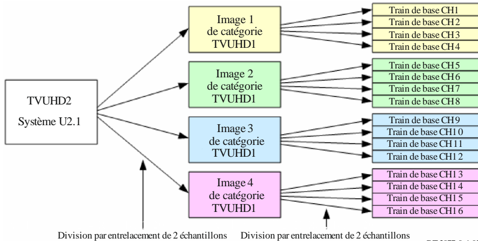
Division en 16 pour le système U2.1
