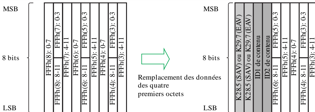
Remplacement de données SAV et EAV multiplexées par un bloc de synchronisation (30, 30/1,001, 25, 24 ou 24/1.001 Hz)
