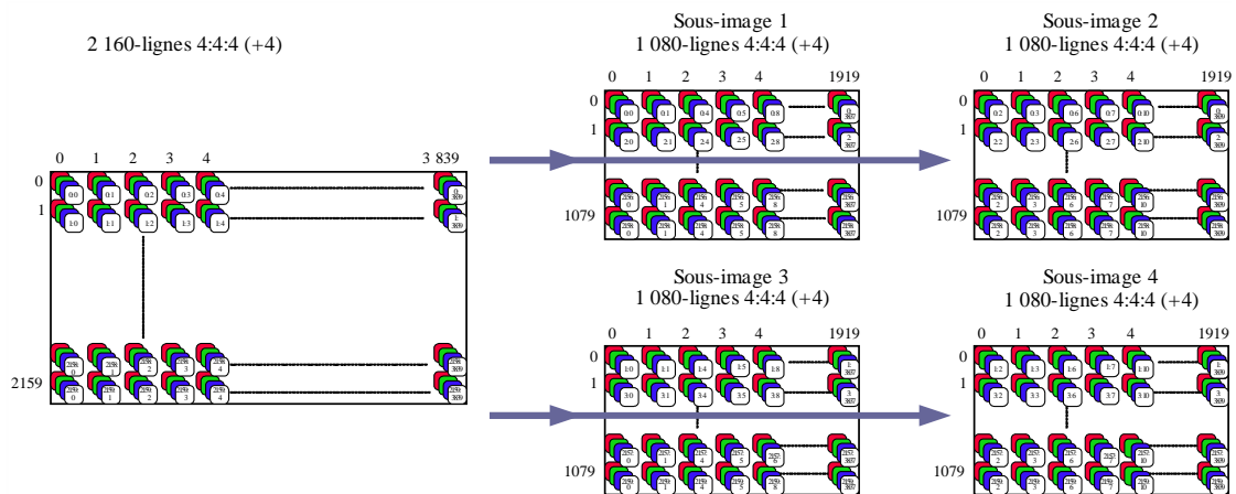
FIGURE 3-23 Division d'une image 4:4:4(+4)
