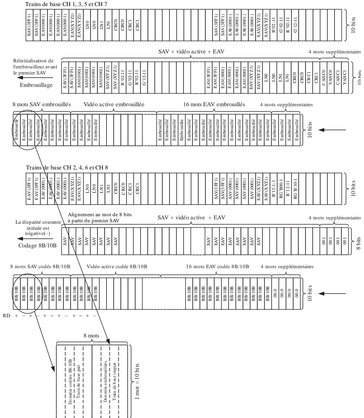
FIGURE 1-23 Mise en blocs de 80 bits en mode D
