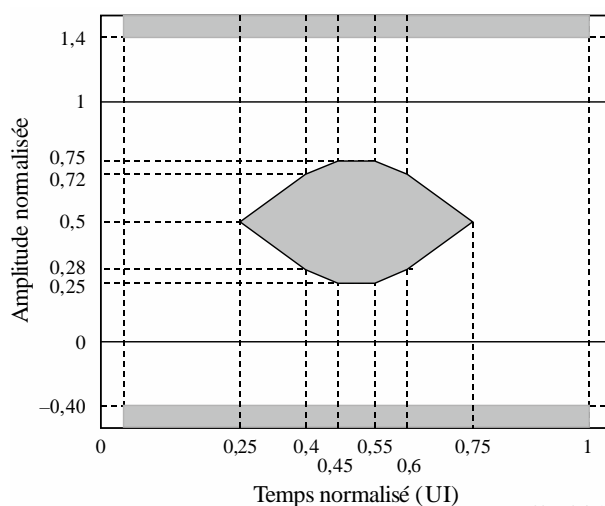
Gabarit de l'œil pour la sortie optique de l'émetteur pour l'interface 106.92G-SDI
