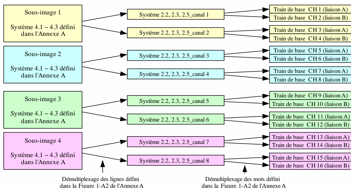
FIGURE 1-3 Division en 16 pour les systèmes U1.7, U1.8 et U1.9
