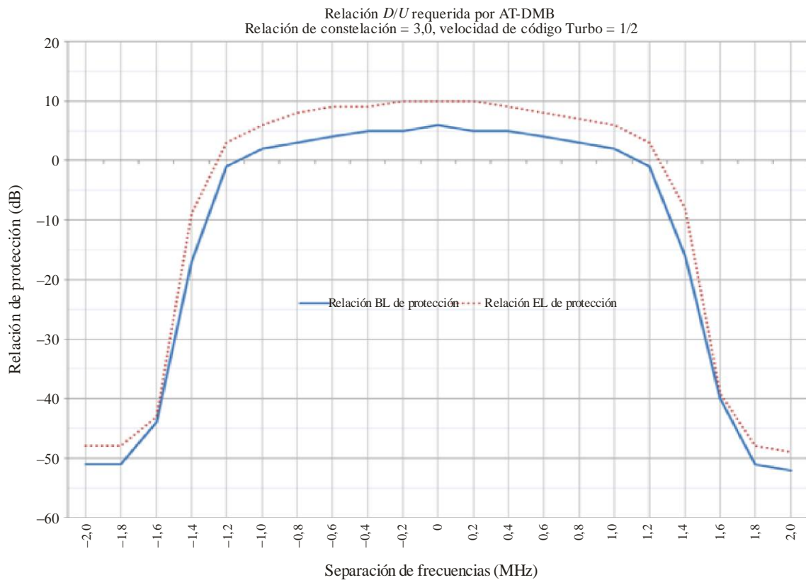
Gráfico de la relación D/U requerida para la señal AT-DMB deseada (Relación de constelación 3,0, velocidad de código Turbo 1/2)
