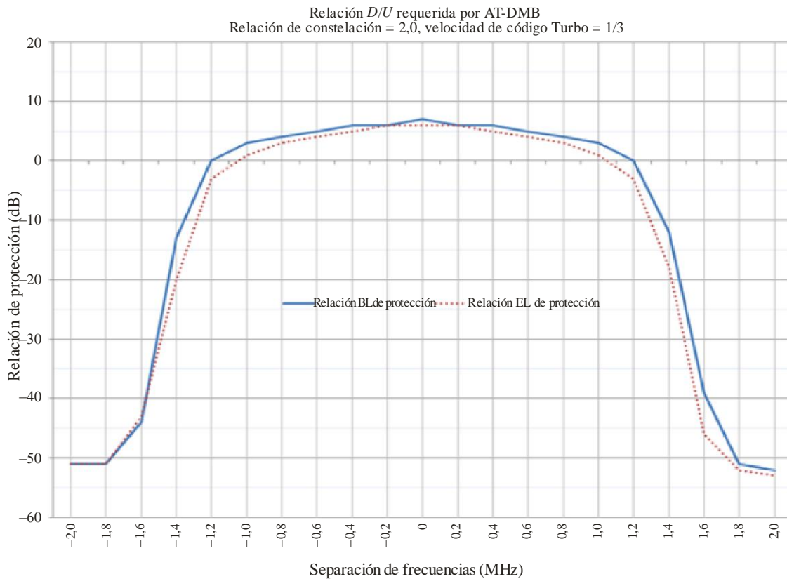
Gráfico de la relación D/U requerida para la señal AT-DMB deseada (Relación de constelación 2,0, velocidad de código Turbo 1/3)
