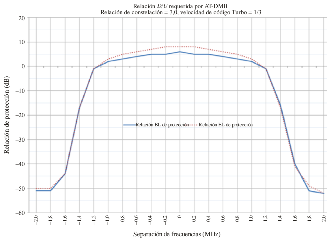
Gráfico de la relación D/U requerida para la señal AT-DMB deseada (Relación de constelación 3,0, velocidad de código Turbo 1/3)
