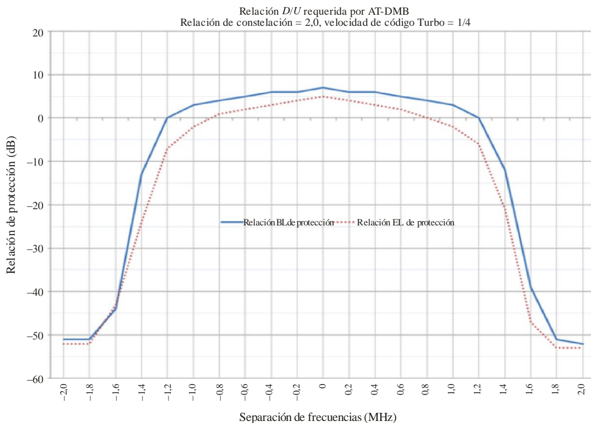
Gráfico de la relación D/U requerida para la señal AT-DMB deseada (Relación de constelación 2,0, velocidad de código Turbo 1/4)
