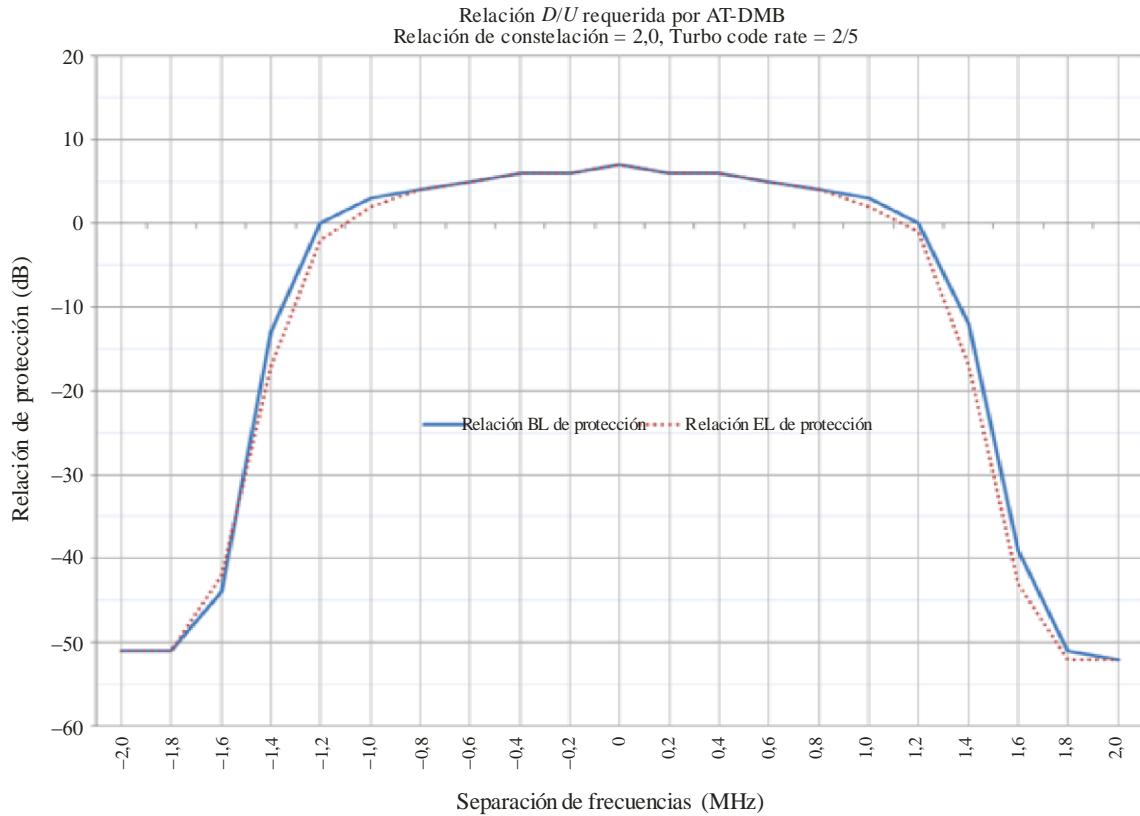
Gráfico de la relación D/U requerida para la señal AT-DMB deseada (Relación de constelación 2,0, velocidad de código Turbo 2/5)
