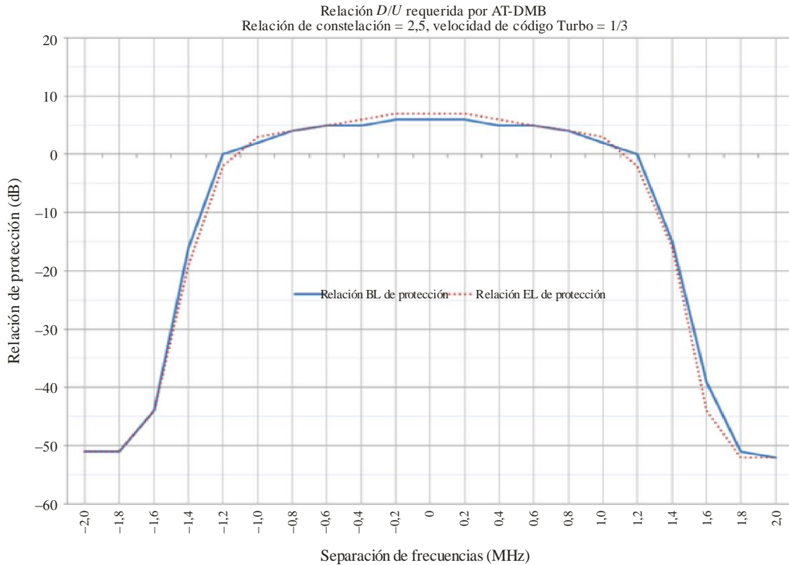
Gráfico de la relación D/U requerida para la señal AT-DMB deseada (Relación de constelación 2,5, velocidad de código Turbo 1/3)
