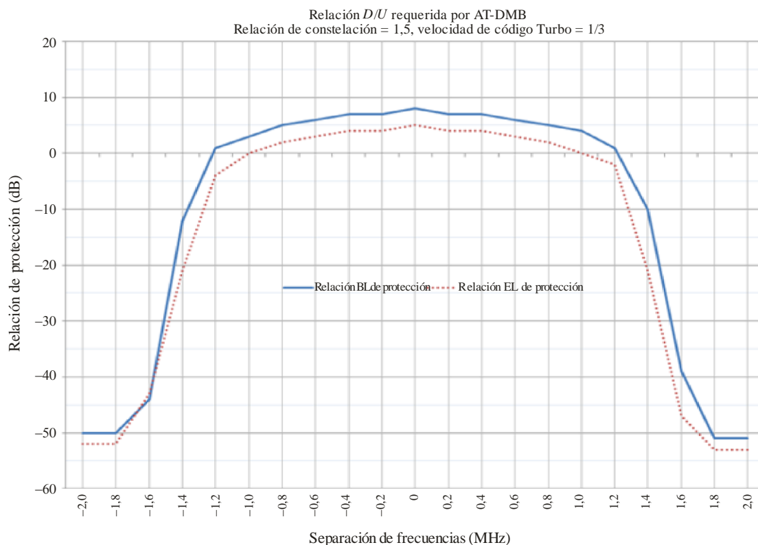
Gráfico de la relación D/U requerida para la señal AT-DMB deseada (Relación de constelación 1,5, velocidad de código Turbo 1/3)
