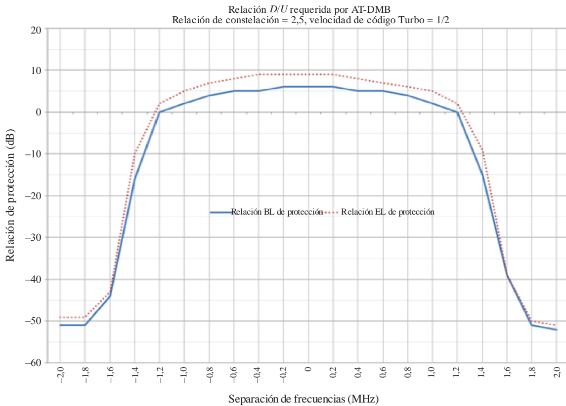
Gráfico de la relación D/U requerida para la señal AT-DMB deseada (Relación de constelación 2,5, velocidad de código Turbo 1/2)
