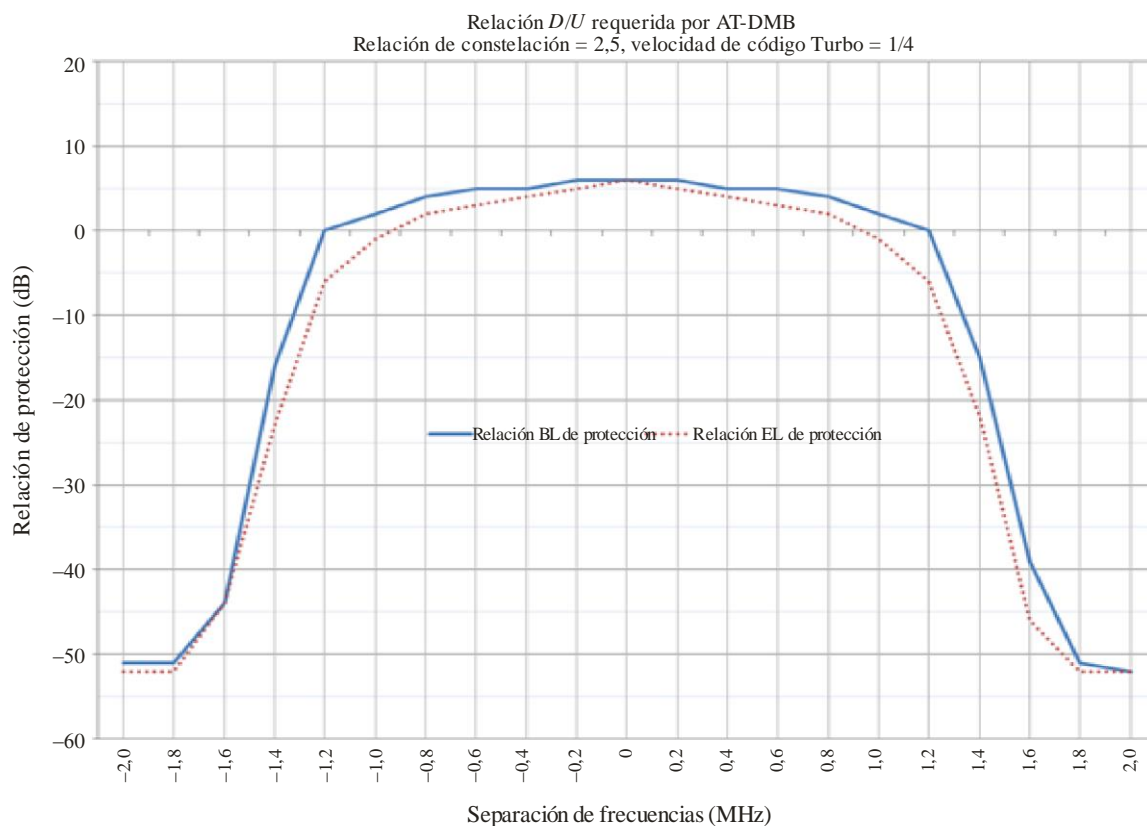
Gráfico de la relación D/U requerida para la señal AT-DMB deseada (Relación de constelación 2,5, velocidad de código Turbo 1/4)
