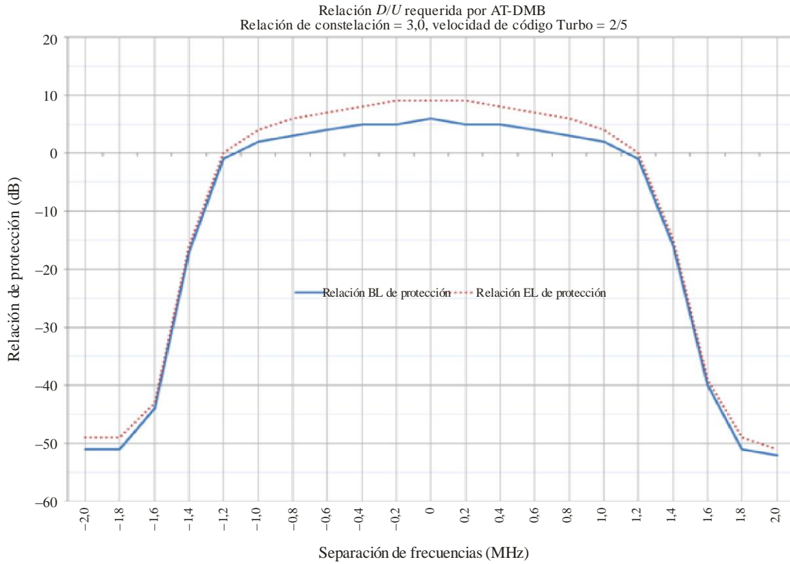
Gráfico de la relación D/U requerida para la señal AT-DMB deseada (Relación de constelación 3,0, velocidad de código Turbo 2/5)
