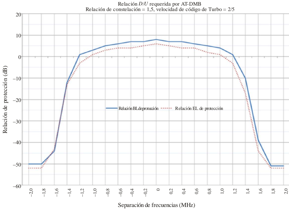
Gráfico de la relación D/U requerida para la señal AT-DMB deseada (Relación de constelación 1,5, velocidad de código Turbo 2/5)
