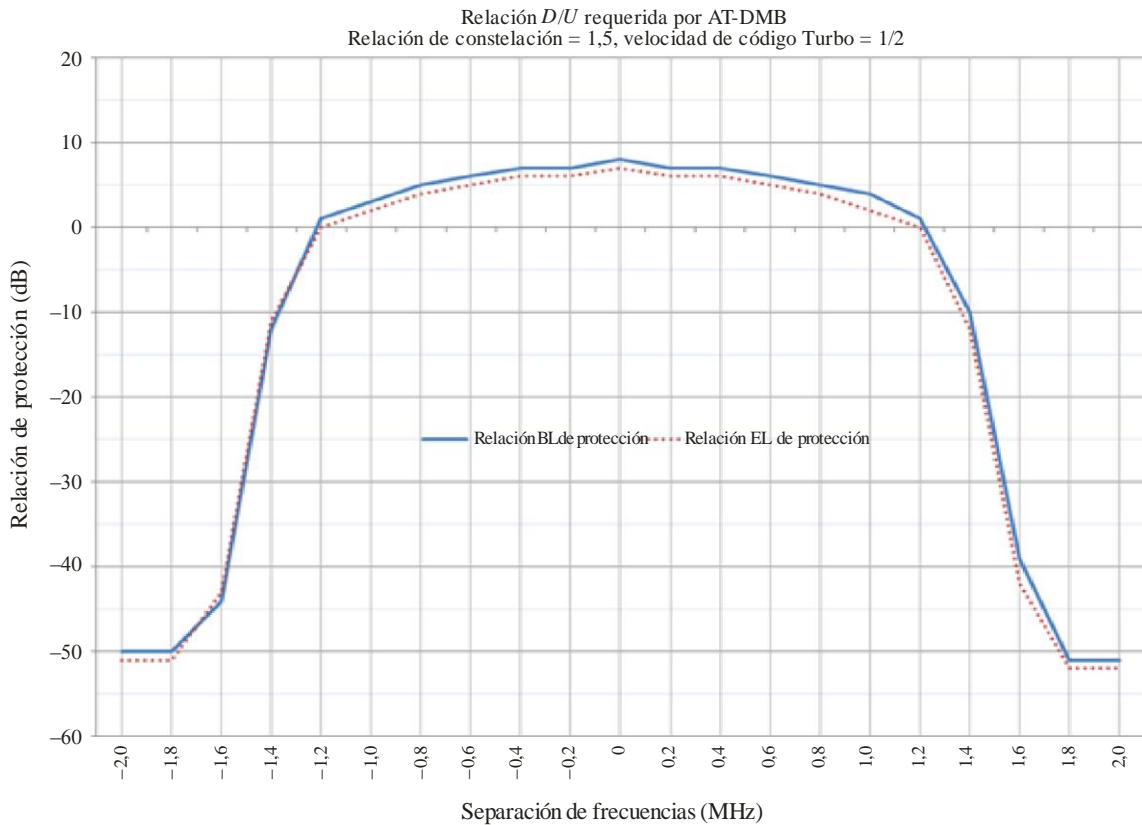
Gráfico de la relación D/U requerida para la señal AT-DMB deseada (Relación de constelación 1,5, velocidad de código Turbo 1/2)
