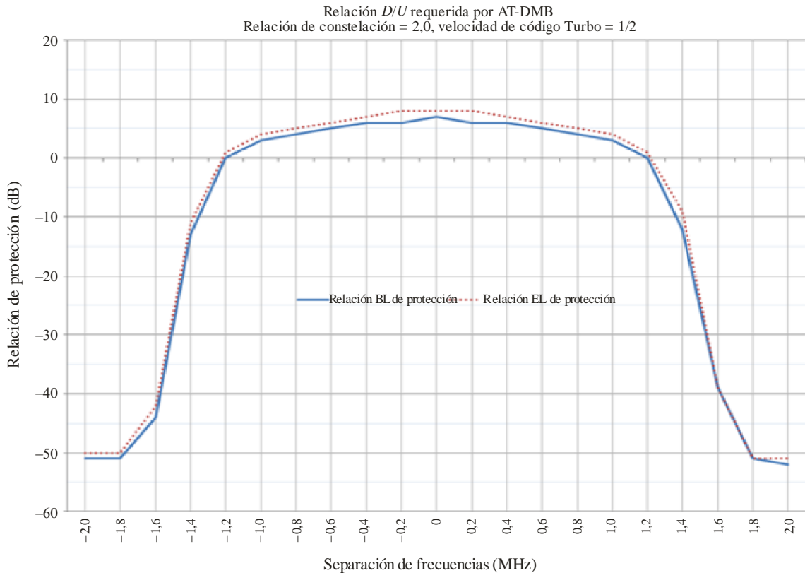
Gráfico de la relación D/U requerida para la señal AT-DMB deseada (Relación de constelación 2,0, velocidad de código Turbo 1/2)
