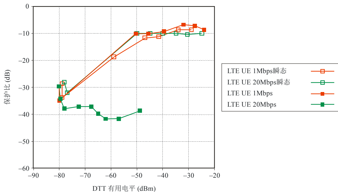
接收机R1 11 MHz偏移
