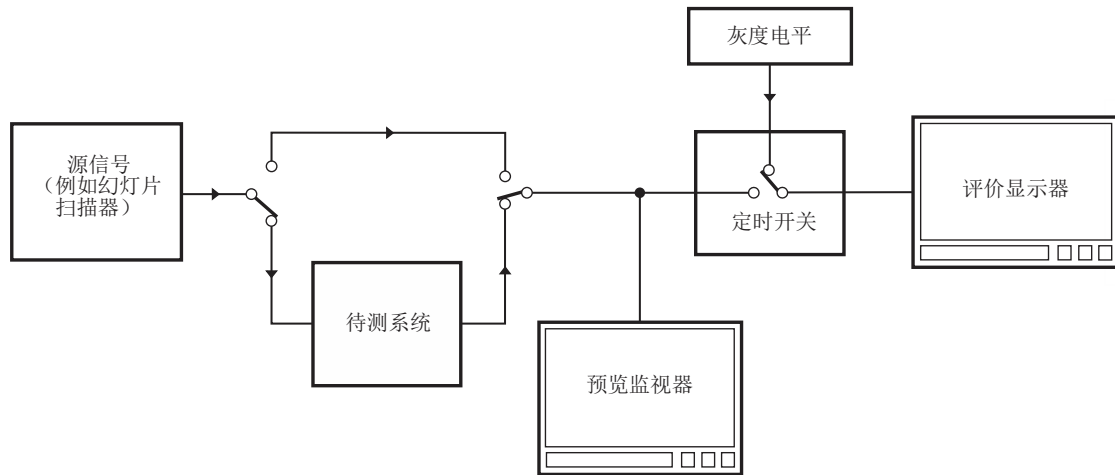
DSIS法中测试系统的总体布置
