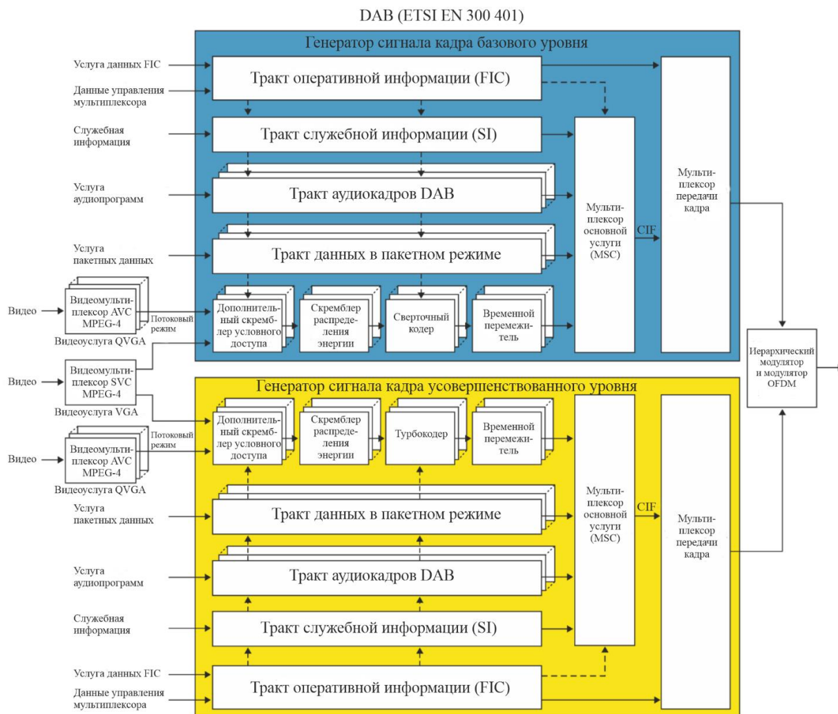
РИСУНОК A1-2 Концептуальная архитектура системы передачи AT-DMB
