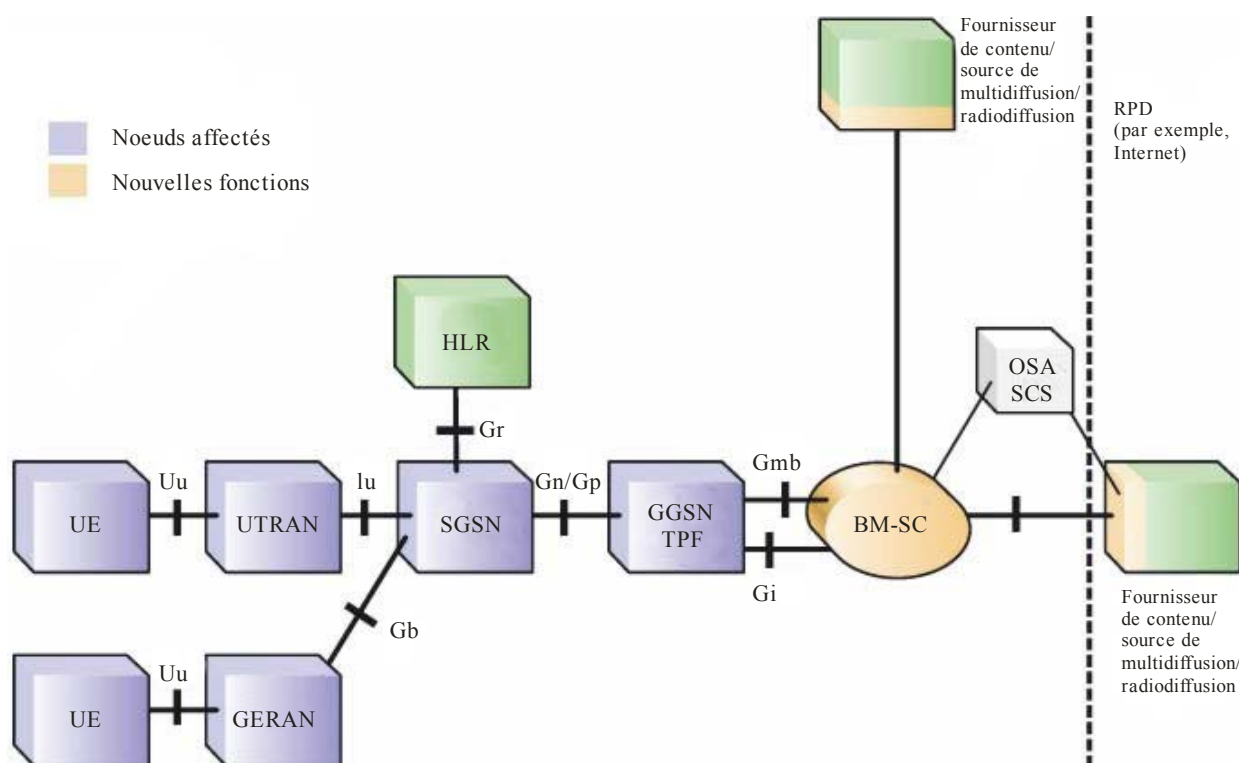
FIGURE 15 Architecture du réseau MBMS
