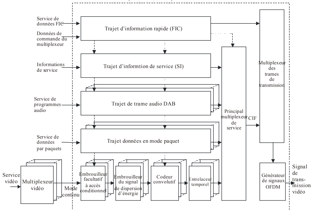
FIGURE 6 Architecture de transmission théorique des services vidéo DAB (ETSI EN 300 401)
