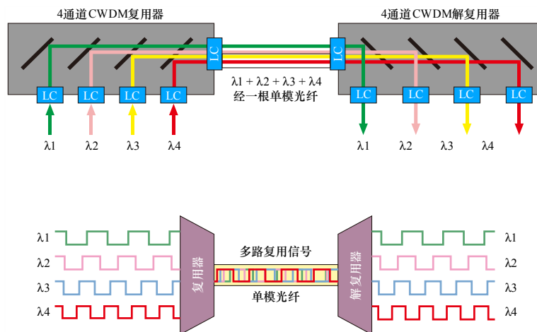
WDM 系统
