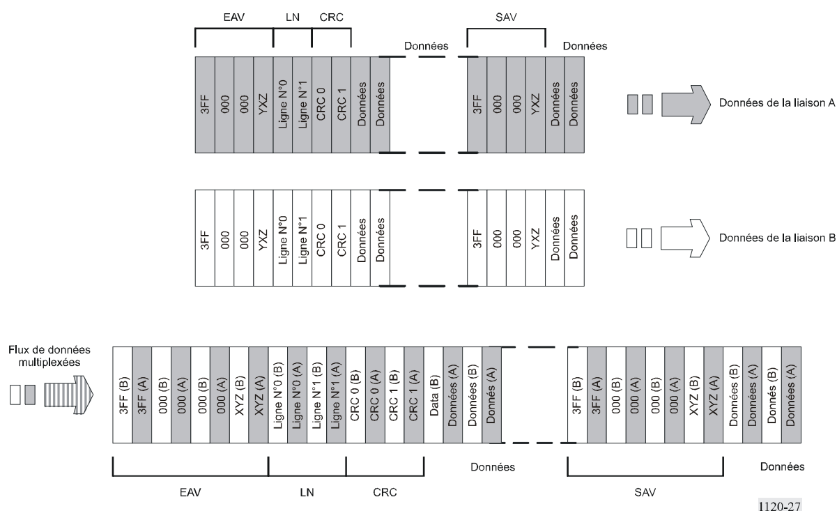
FIGURE 27 Multiplexage liaison double - liaison unique
