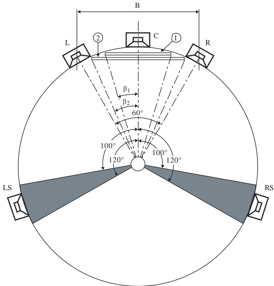
FIGURA 1 Disposición de los altavoces de referencia L/C/R y LS/RS
