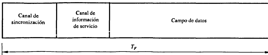
Estructura de la trama múltiplex
