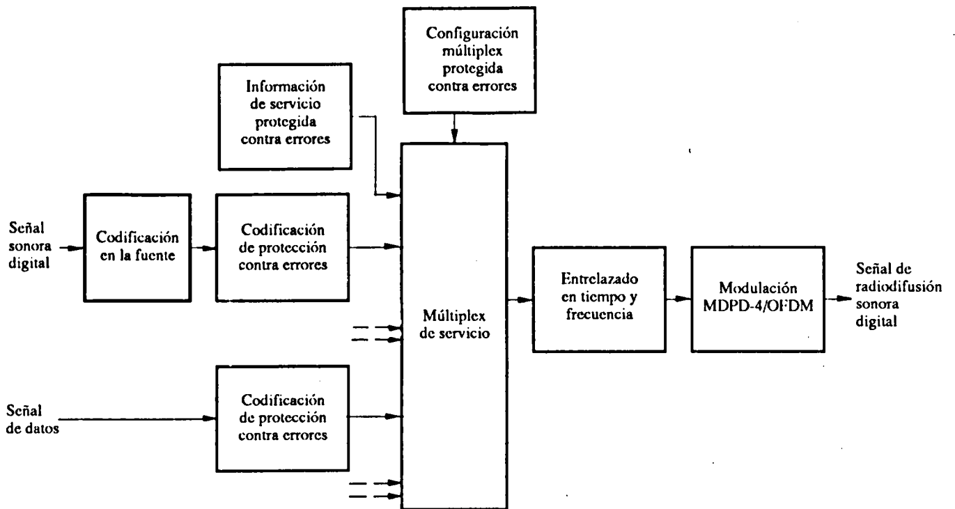
FIGURA 1 Diagrama de bloques conceptual del transmisor de sistema digital A
