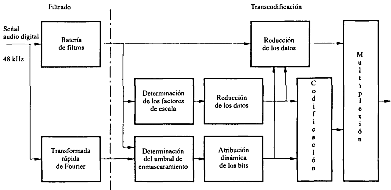
Diagrama de bloques de un codificador de sonido básico del sistema digital A
