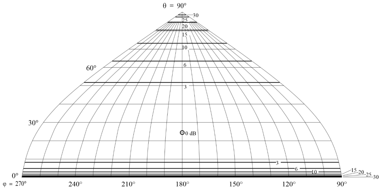
FIGURA 90D Diagrama de radiación hacia atrás
