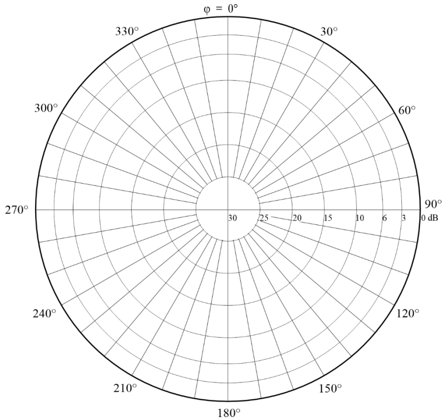
FIGURA 90B Diagrama horizontal para un ángulo de elevación de 24°
