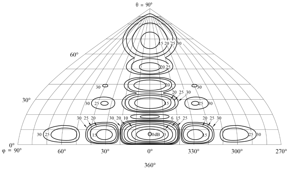
FIGURA 79C Diagrama de radiación hacia adelante
