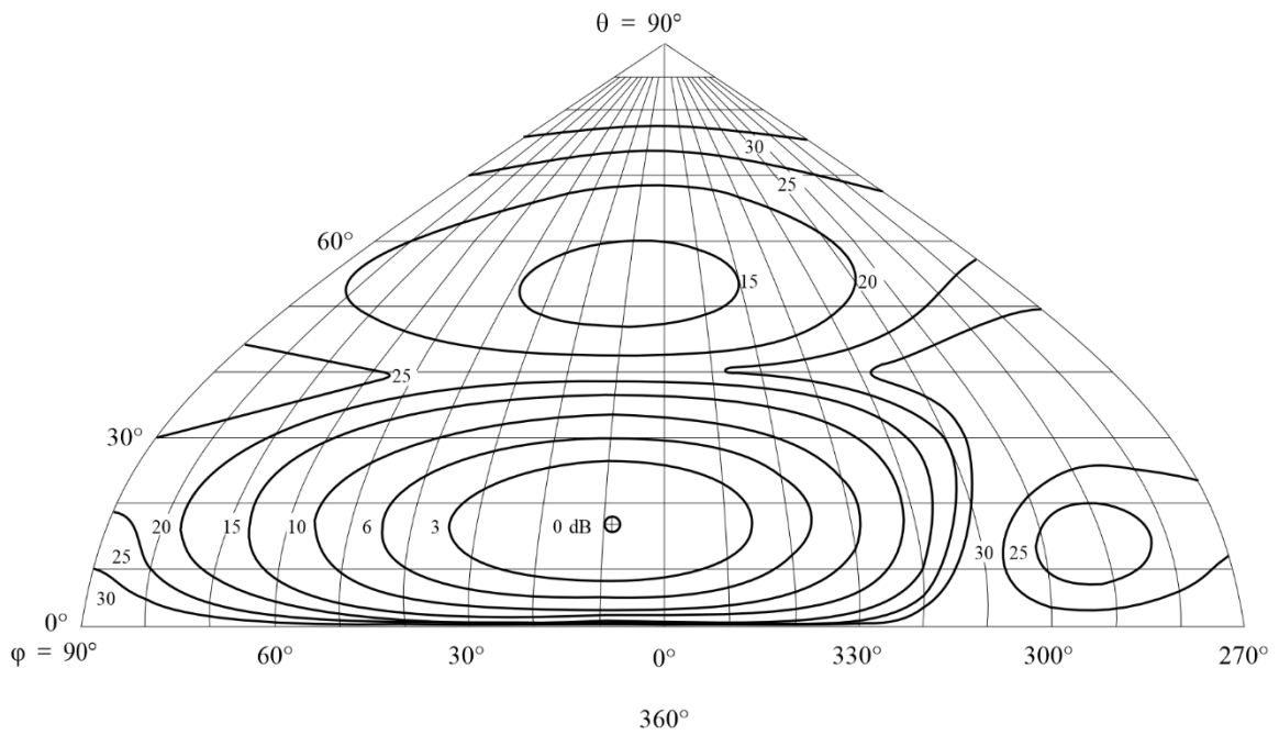
FIGURA 71C Diagrama de radiación hacia adelante
