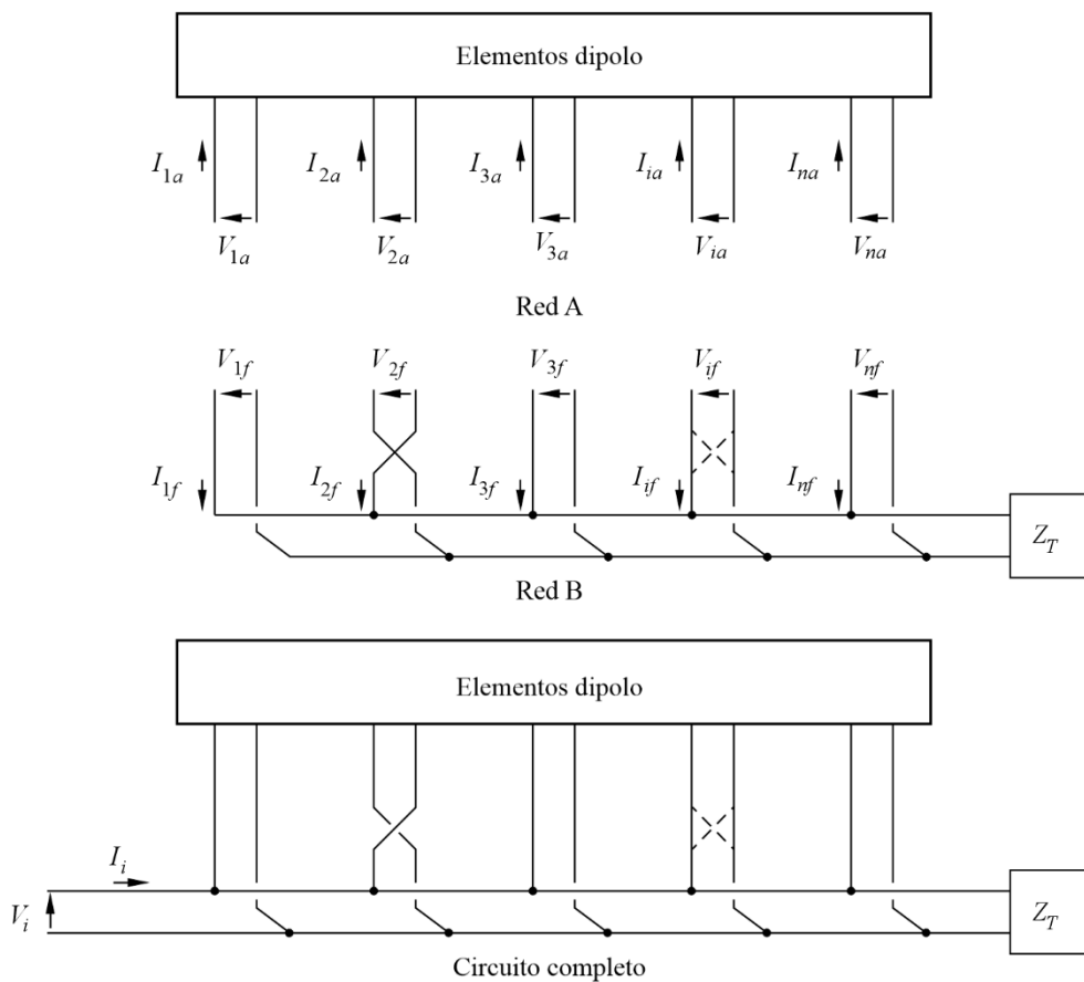
FIGURA 30 Disposición esquemática de la red del sistema
