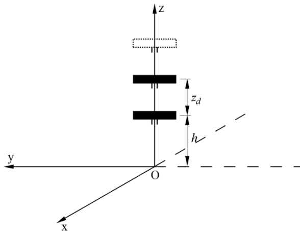
FIGURA 20 Superposición de elementos a lo largo del eje z
