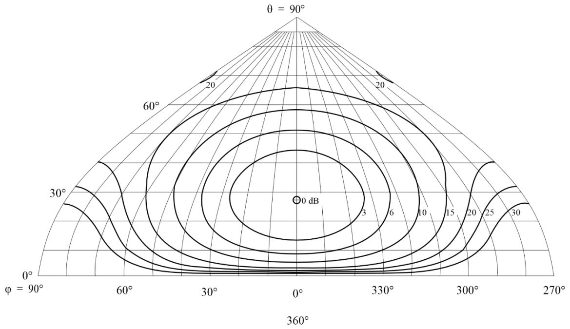
FIGURA 69C Diagrama de radiación hacia adelante
