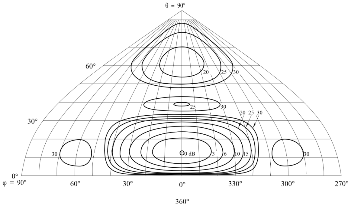
FIGURA 75C Diagrama de radiación hacia adelante
