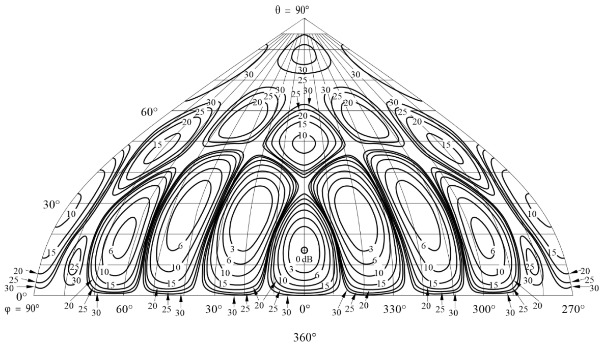
Diagrama de radiación hacia adelante
