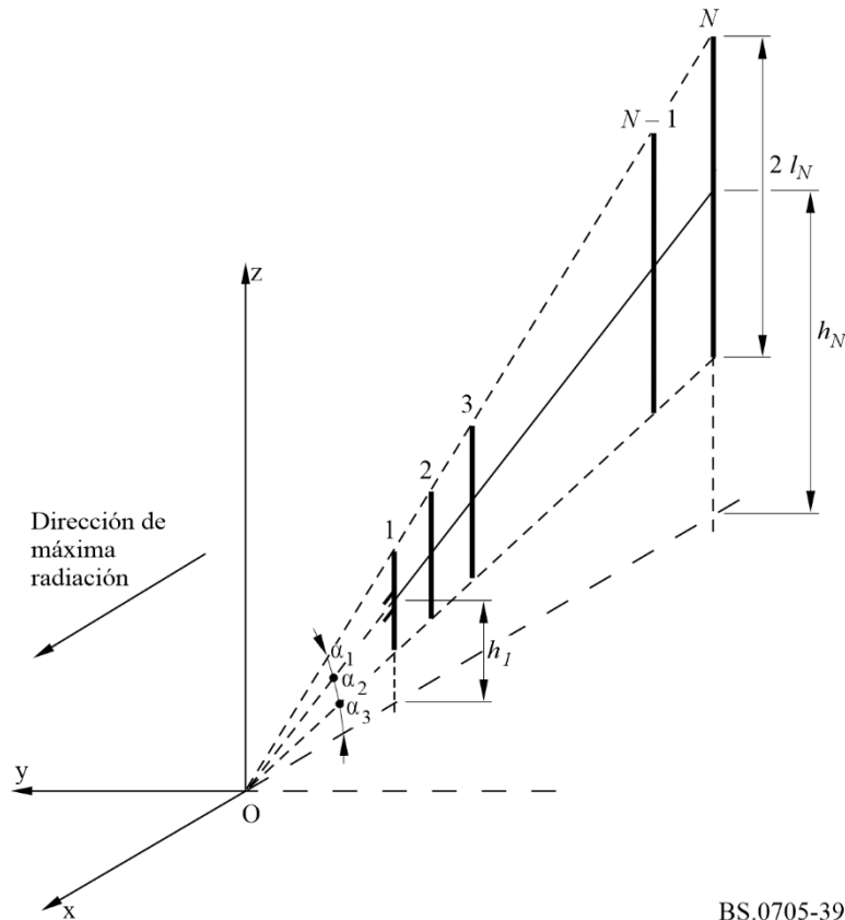
Antena log-periódica vertical (elementos a altura variable)
