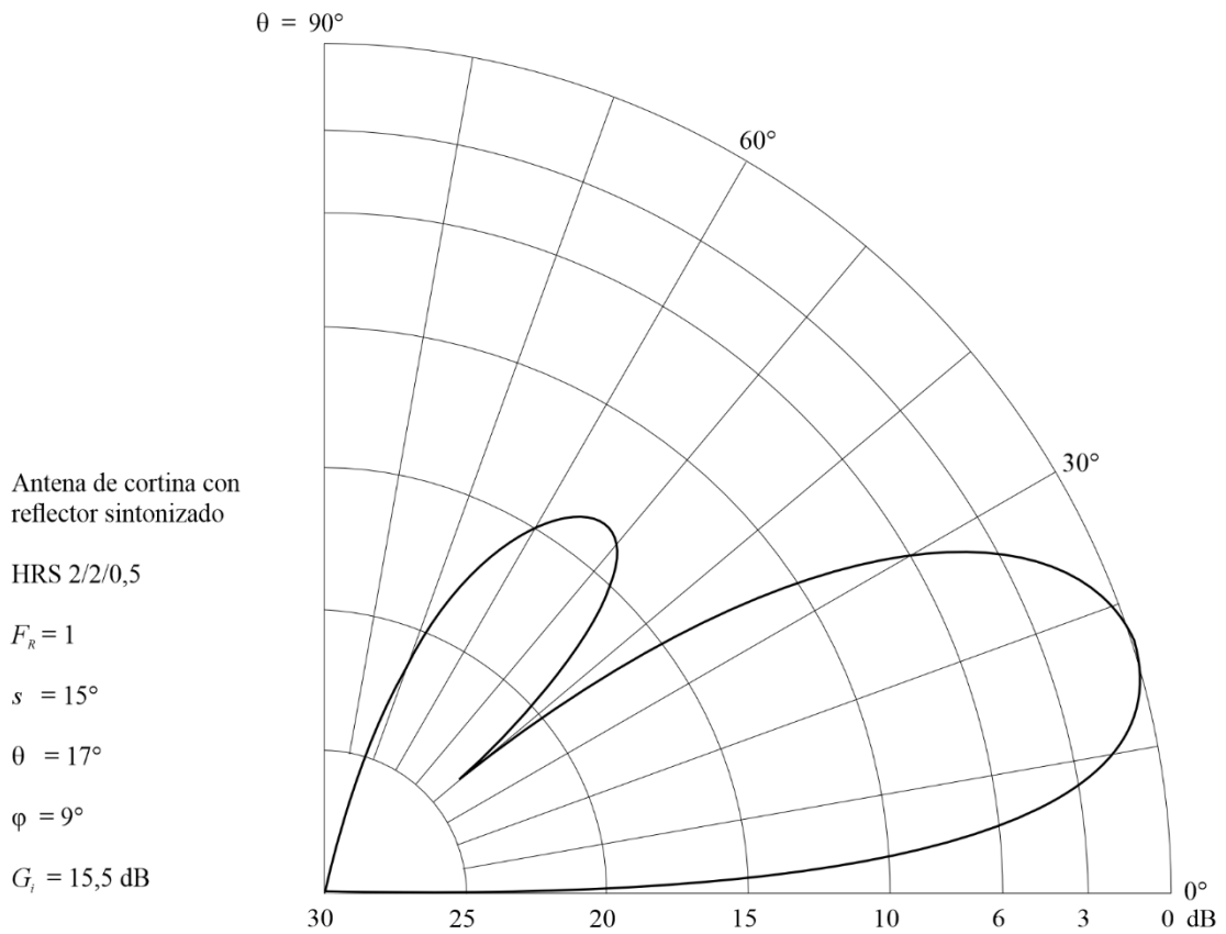
FIGURA 71A Diagrama vertical para un ángulo acimutal de 9^\circ
