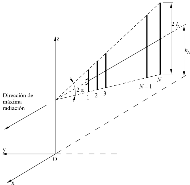
FIGURA 38 Antena log-periódica vertical (elementos a altura fija)
