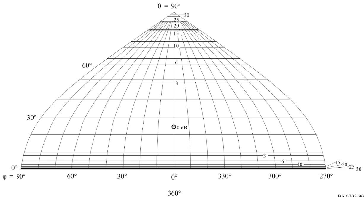
FIGURA 90C Diagrama de radiación hacia adelante
