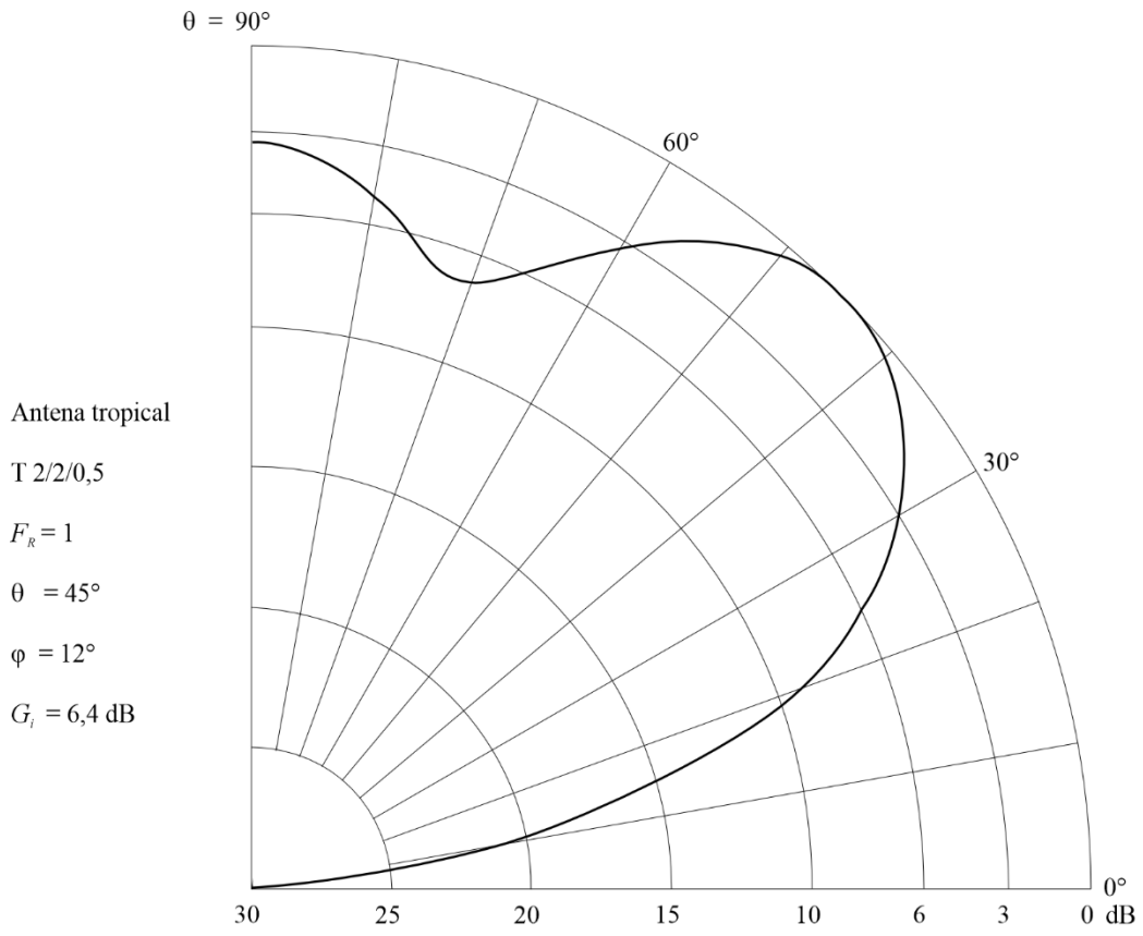
Diagrama vertical para un ángulo acimutal de 12°
