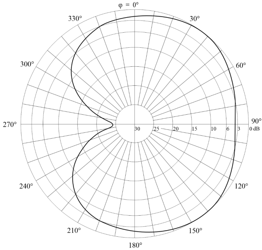
FIGURA 84B Diagrama horizontal para ángulo de elevación de 40°
