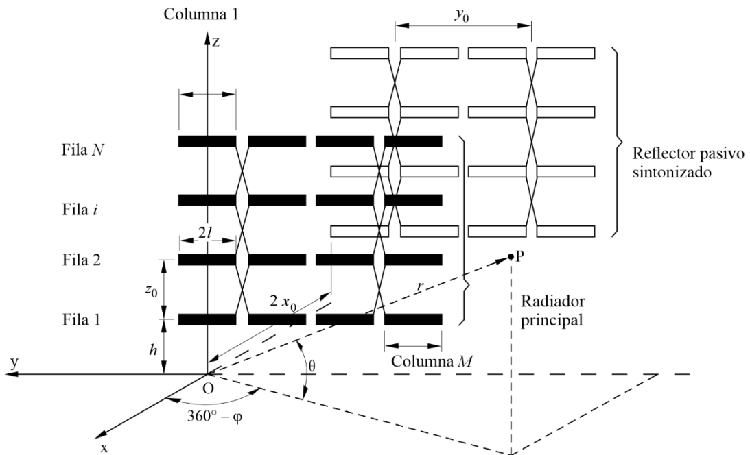
FIGURA 18 Sistema de dipolos alimentados por el extremo (HR 4/4) con reflector sintonizado
