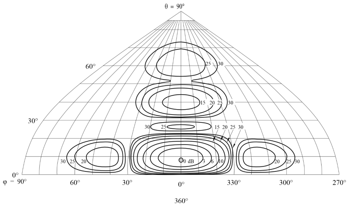
Diagrama de radiación hacia adelante
