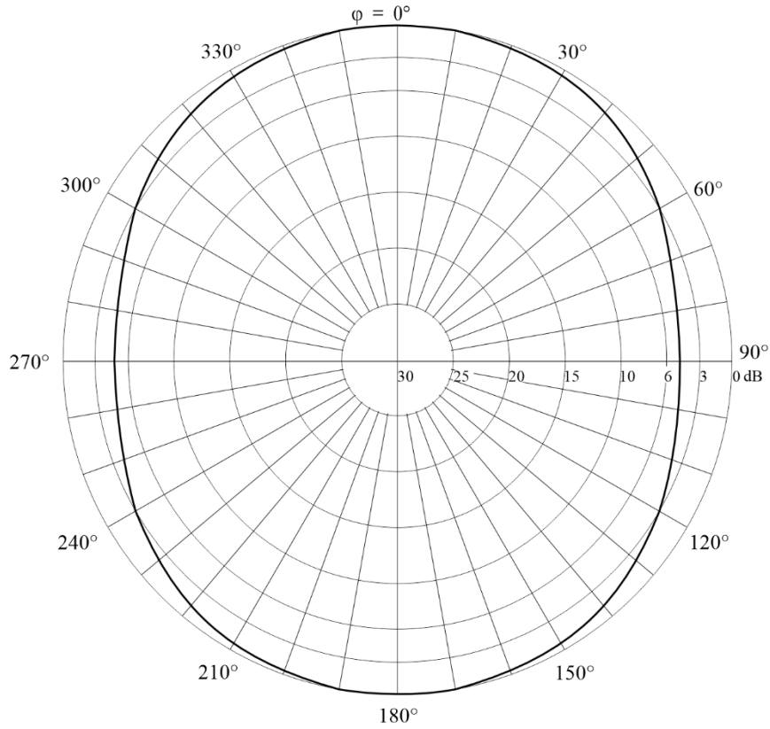
FIGURA 88B Diagrama vertical para un ángulo de elevación de 51°
