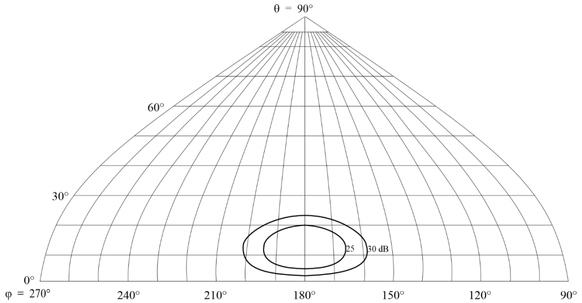
FIGURA 74D Diagrama de radiación hacia atrás
