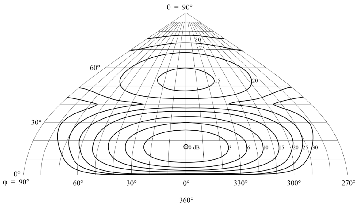
FIGURA 70C Diagrama de radiación hacia adelante
