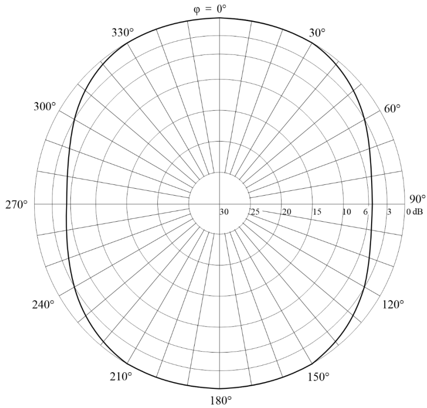
FIGURA 83B Diagrama horizontal para un ángulo de elevación de 45°
