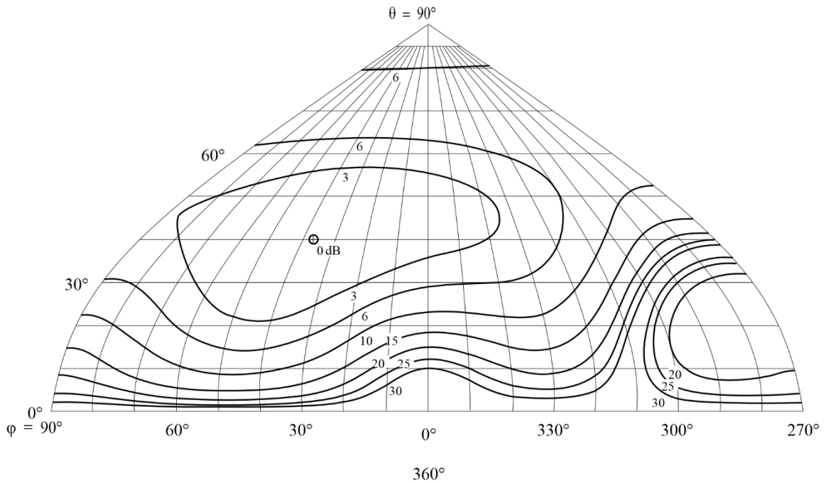
FIGURA 84C Diagrama de radiación hacia adelante
