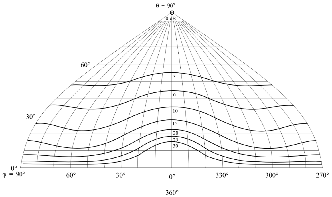
FIGURA 82C Diagrama de radiación hacia adelante
