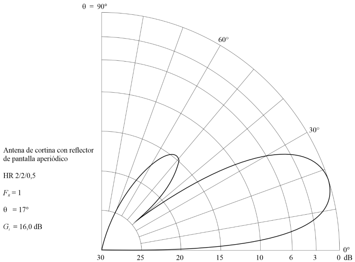
FIGURA 72A Diagrama vertical para un ángulo acimutal de 0°
