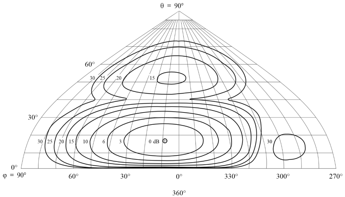
FIGURA 73C Diagrama de radiación hacia adelante
