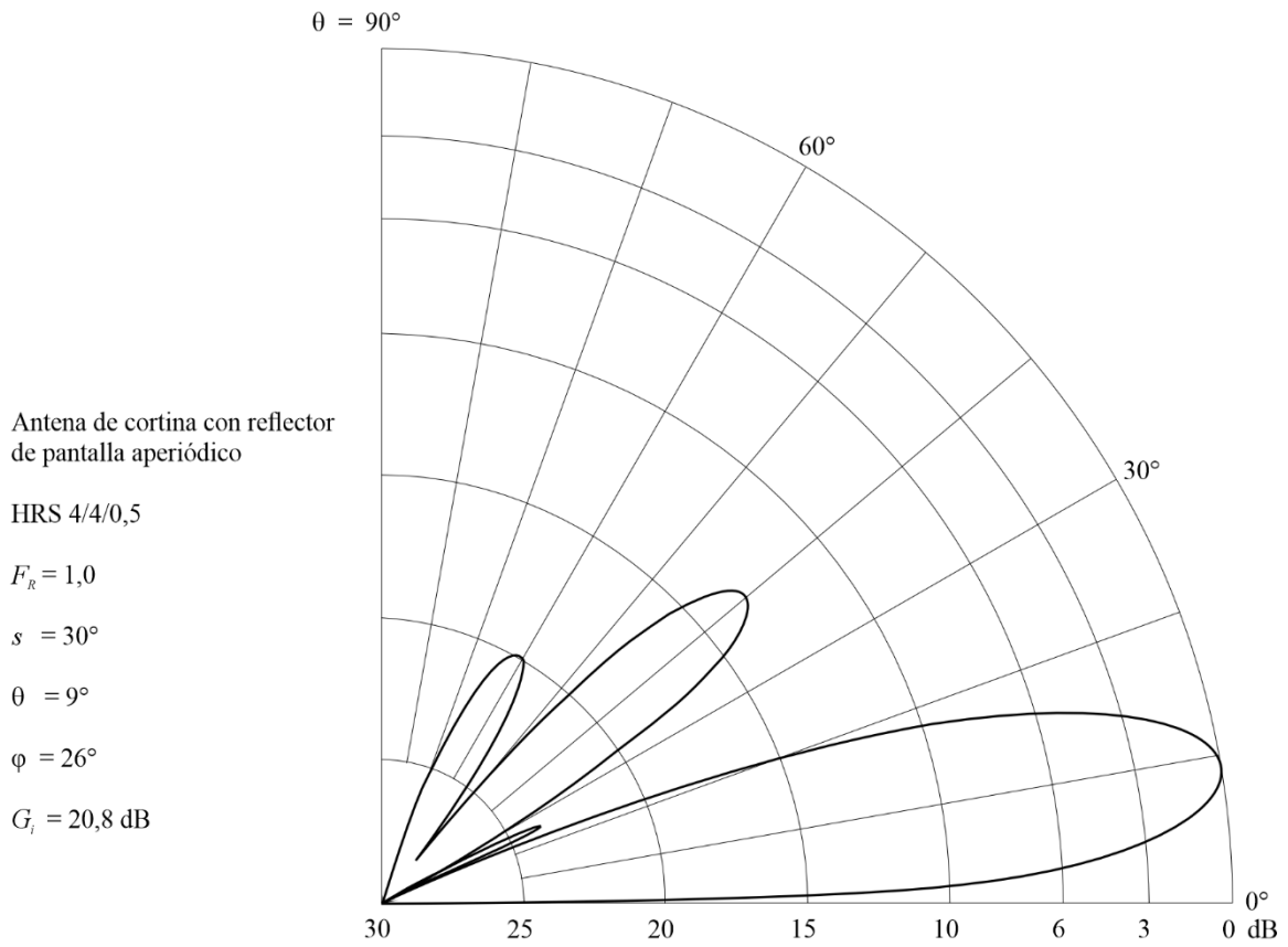
Diagrama vertical para un ángulo acimutal de 26°
