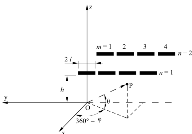
FIGURA 6 Antena tropical
