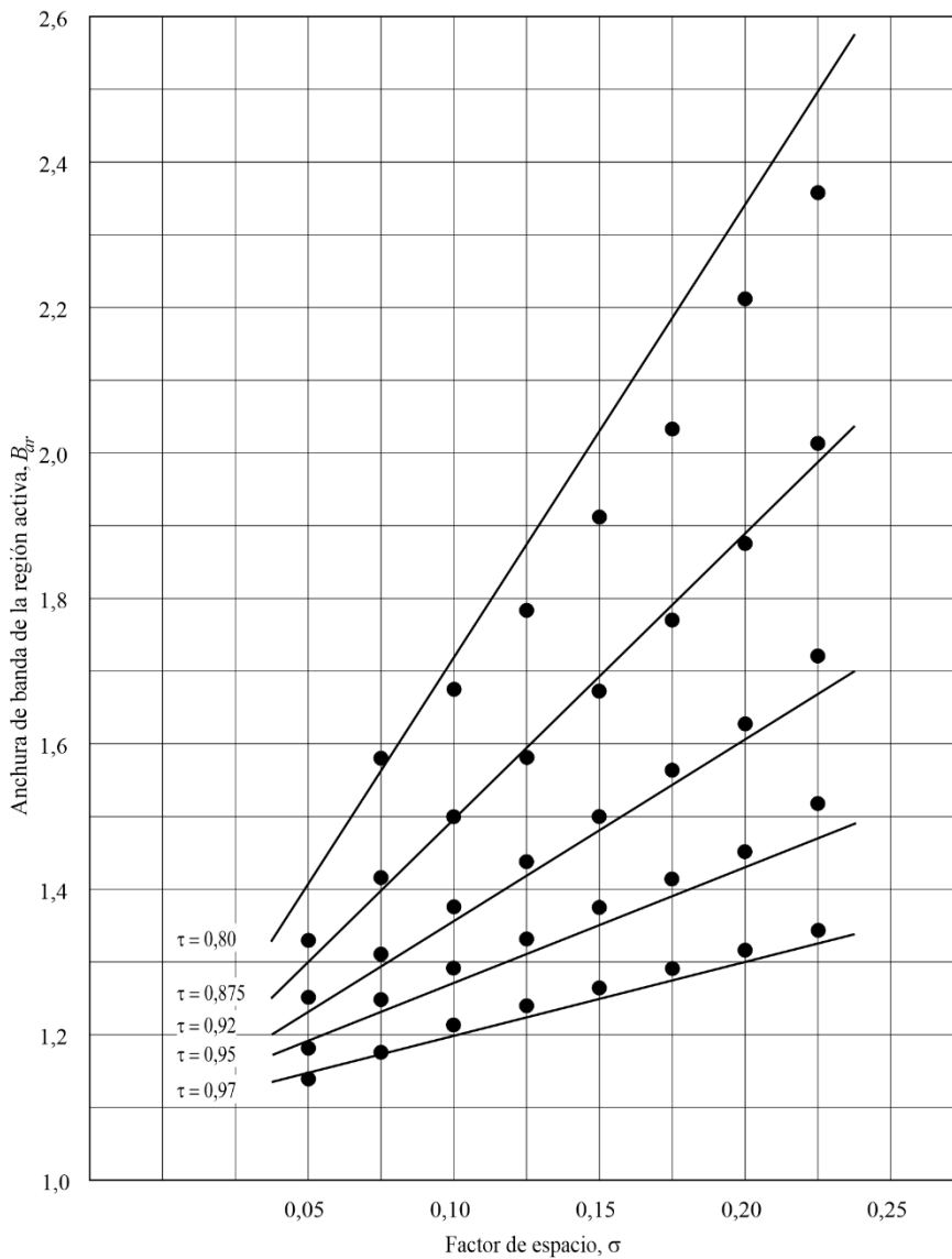
Anchura de banda de la región activa B_{ar} en función de \sigma y \tau
