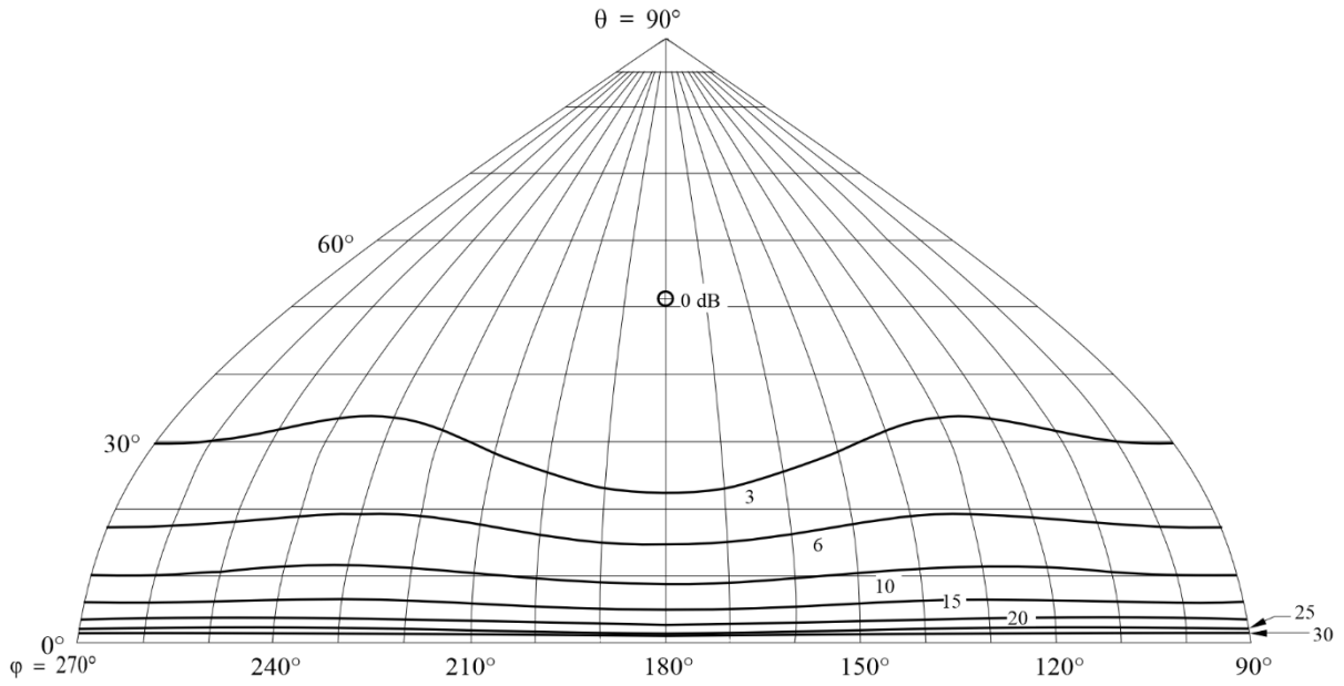
FIGURA 87D Diagrama de radiación hacia atrás
