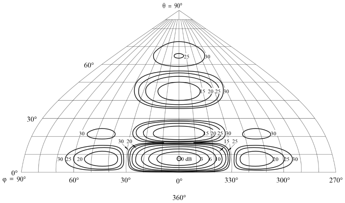
FIGURA 81C Diagrama de radiación hacia adelante
