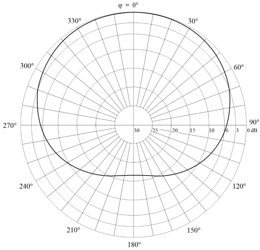
Diagrama horizontal para un ángulo de elevación de 17°
