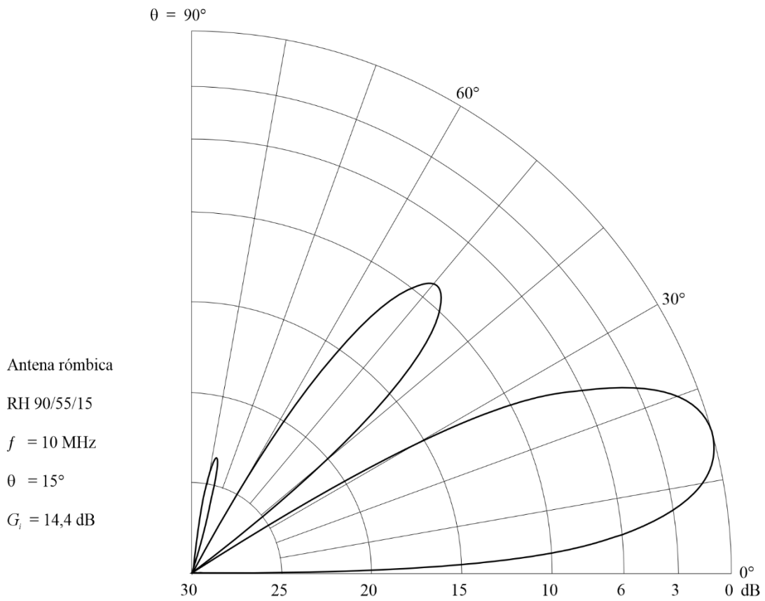
FIGURA 89A Diagrama vertical para un ángulo acimutal de 0°
