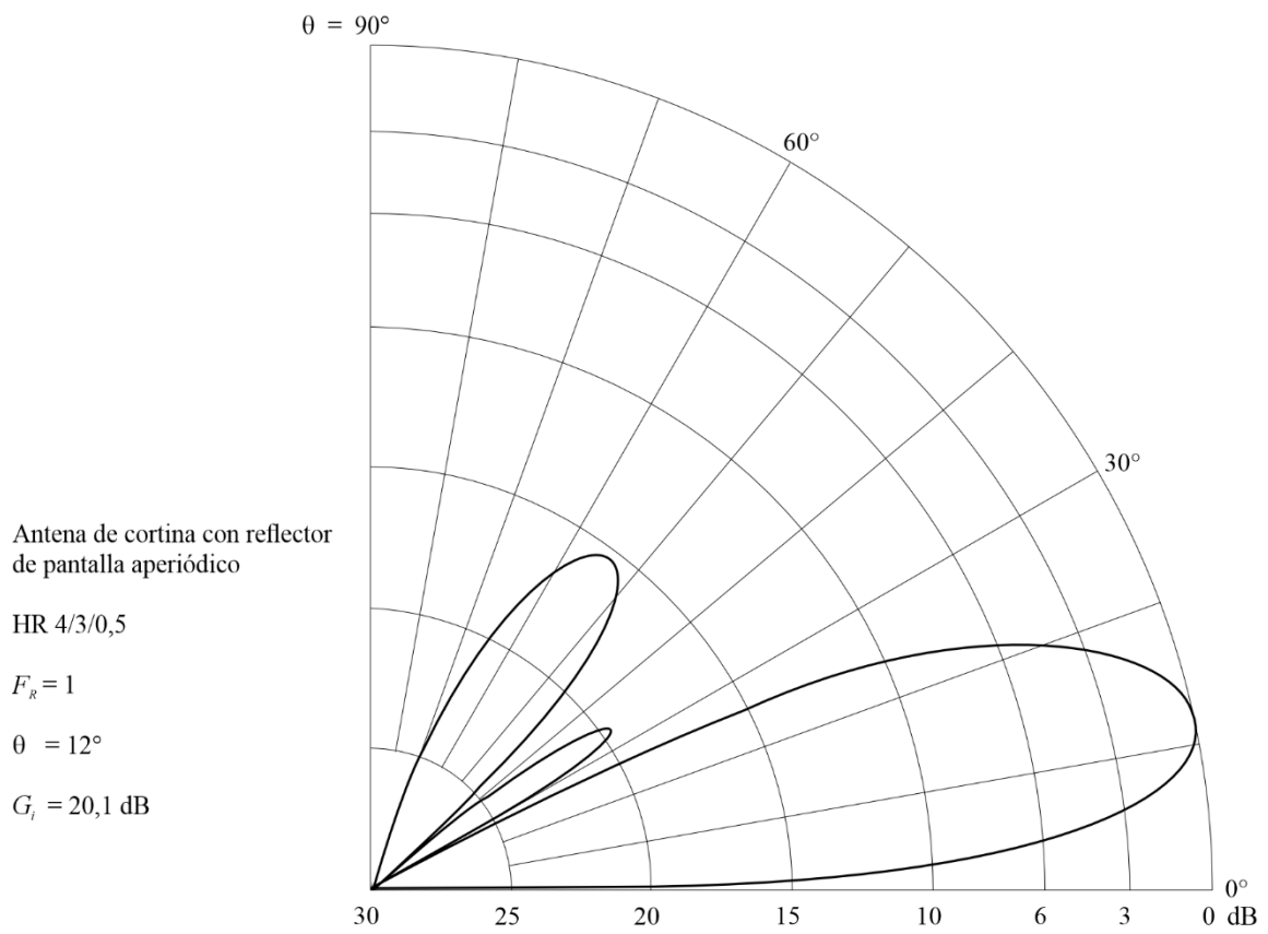
FIGURA 74A Diagrama vertical para un ángulo acimutal de 0^\circ
