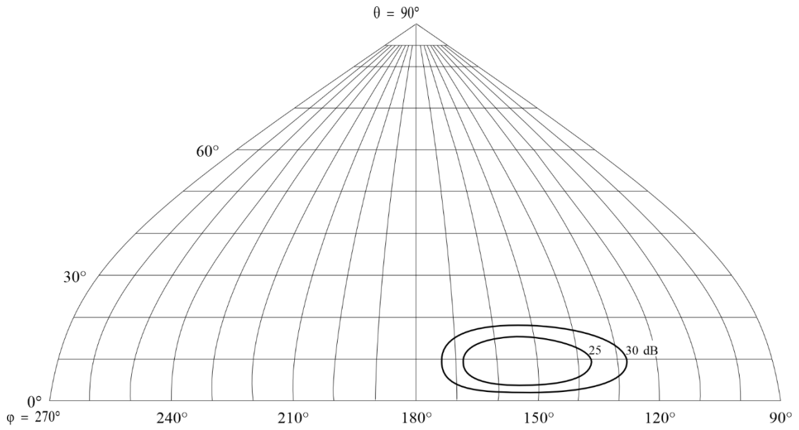
FIGURA 78D Diagrama de radiación hacia atrás
