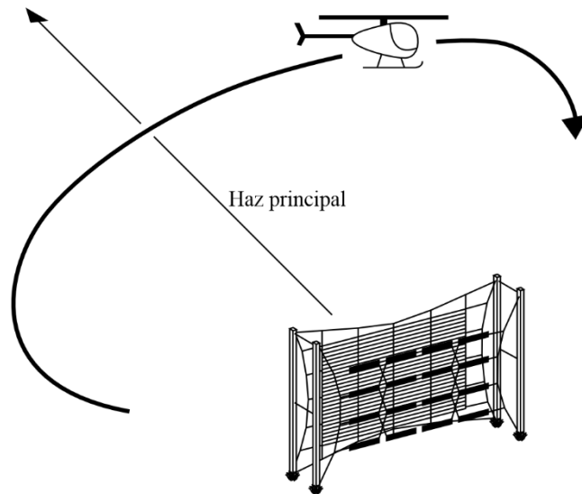
FIGURA 49 Trayecto de vuelo para la medición del DRH
