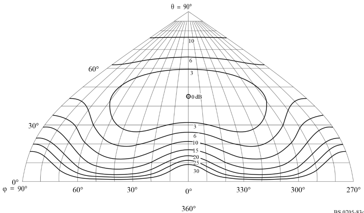
FIGURA 83C Diagrama de radiación hacia adelante
