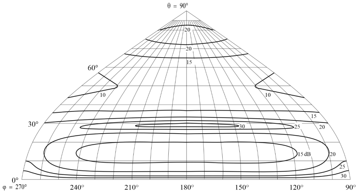
FIGURA 85D Diagrama de radiación hacia atrás
