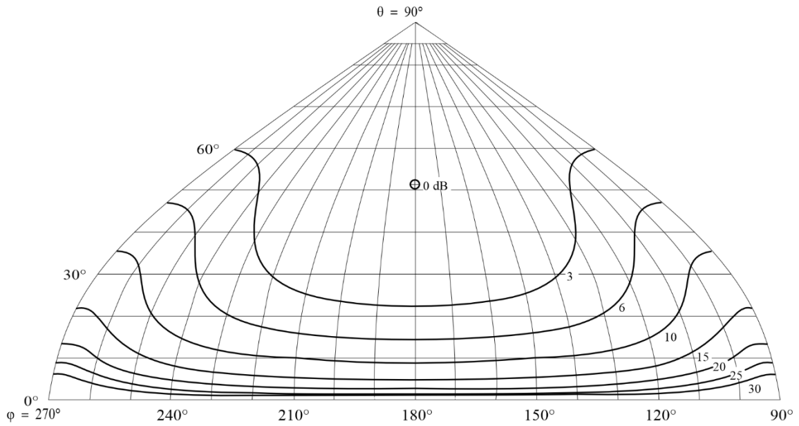
FIGURA 88D Diagrama de radiación hacia atrás
