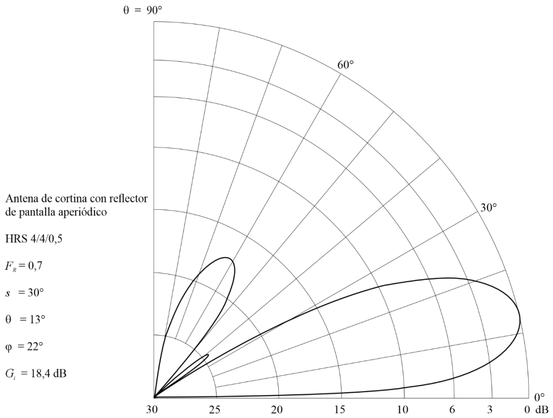
Diagrama vertical para un ángulo acimutal de 22°
