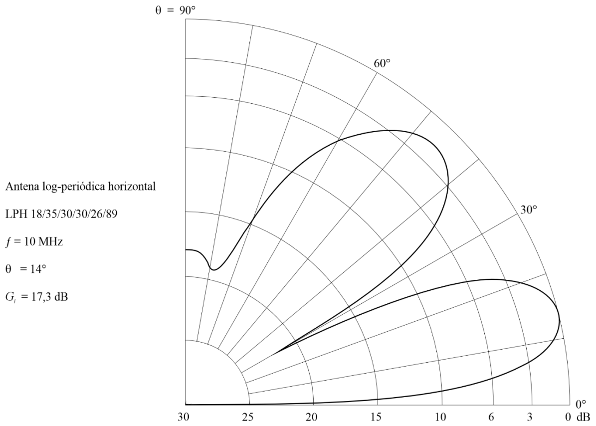
Diagrama vertical para un ángulo acimutal de 0°
