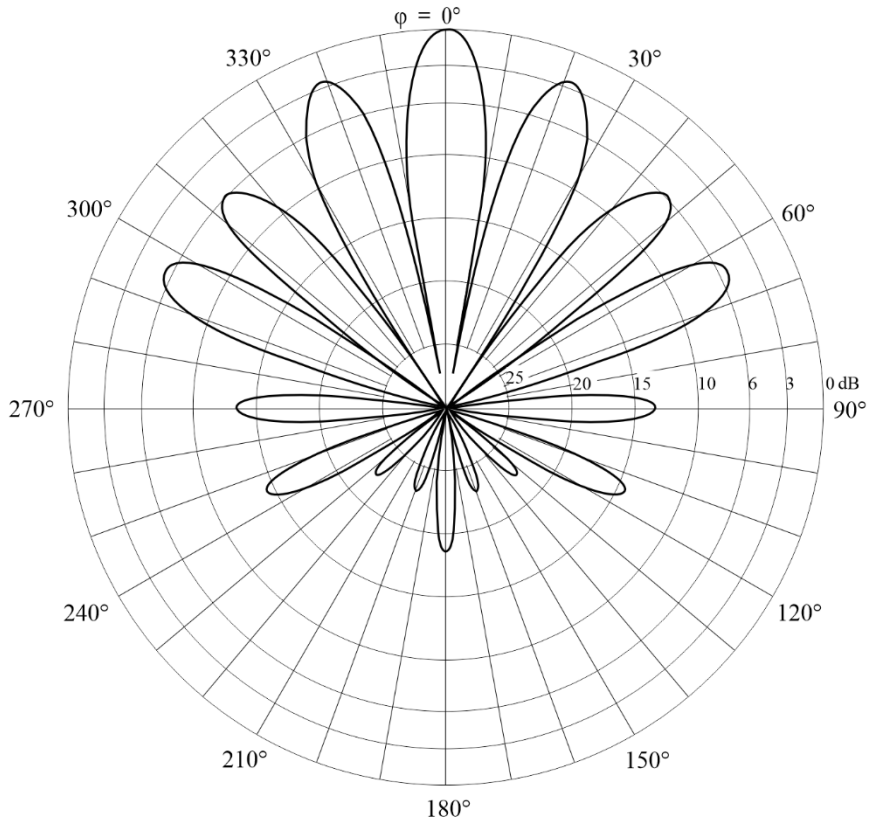
Diagrama horizontal para un ángulo de elevación de 15°
