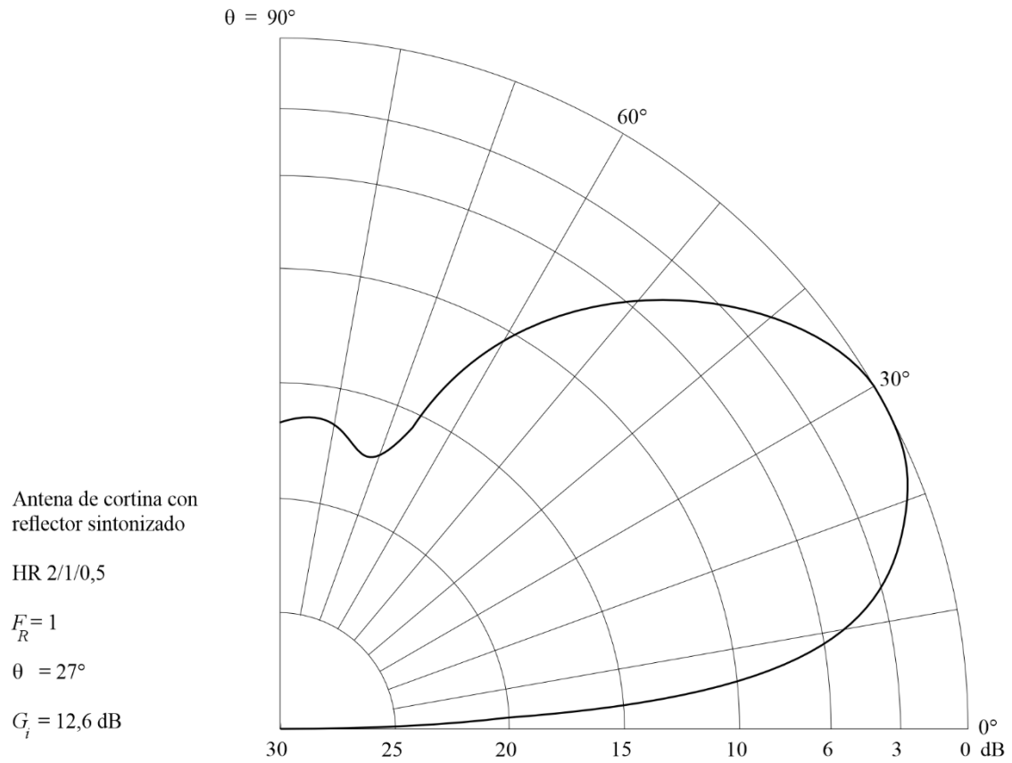
Diagrama vertical para un ángulo acimutal de 0°
