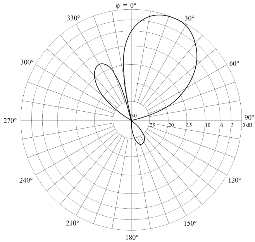
Diagrama horizontal para un ángulo de elevación de 13°
