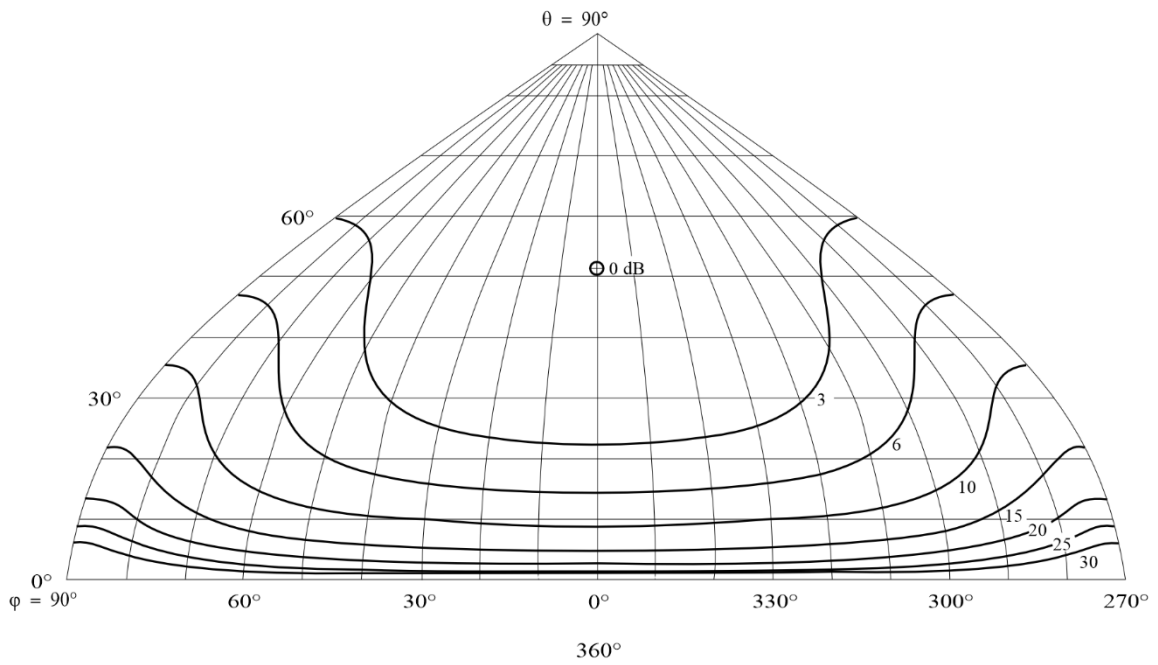
FIGURA 88C Diagrama de radiación hacia adelante
