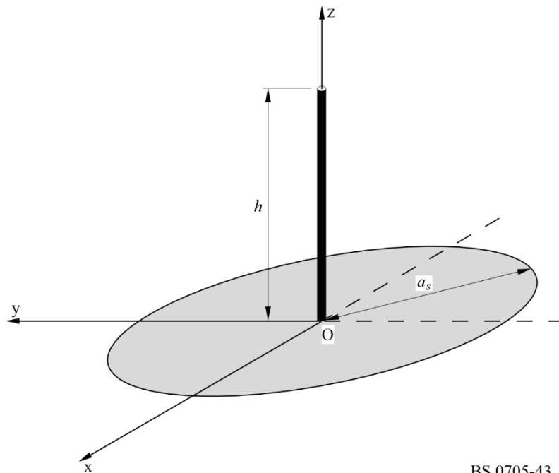
Monopolo vertical en terreno homogéneo llano, con un sistema de tierra compuesto por un disco circular sólido de conductividad infinita
