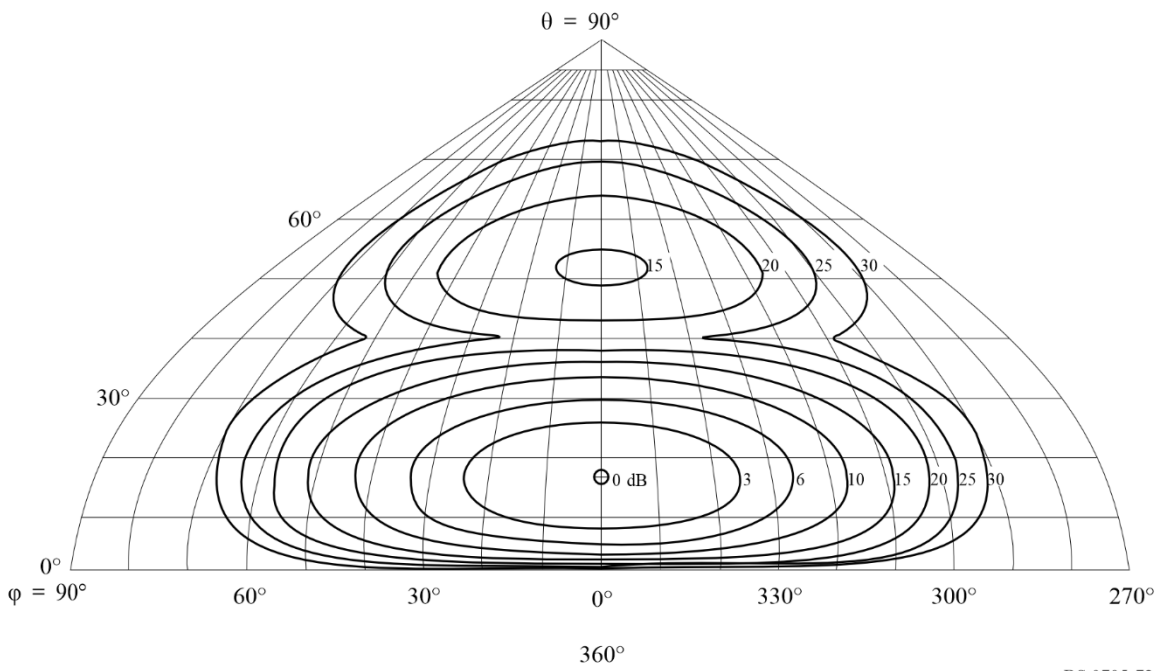
FIGURA 72C Diagrama de radiación hacia adelante
