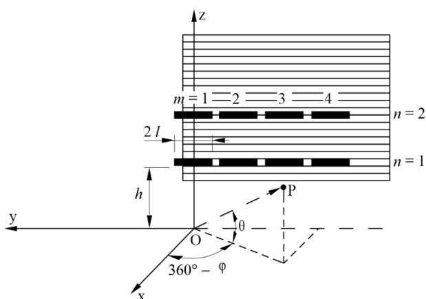
FIGURA 5 Antena de cortina
