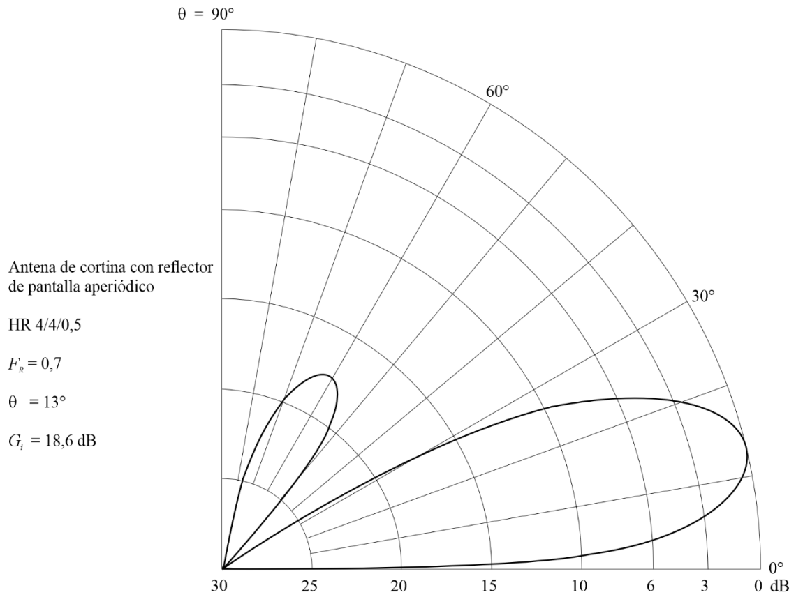
FIGURA 75A Diagrama vertical para un ángulo acimutal de 0^\circ
