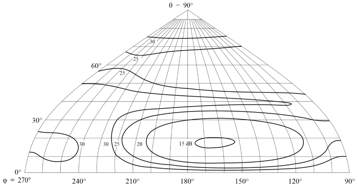
FIGURA 71D Diagrama de radiación hacia atrás
