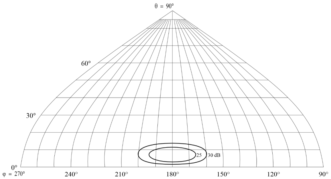
FIGURA 81D Diagrama de radiación hacia atrás
