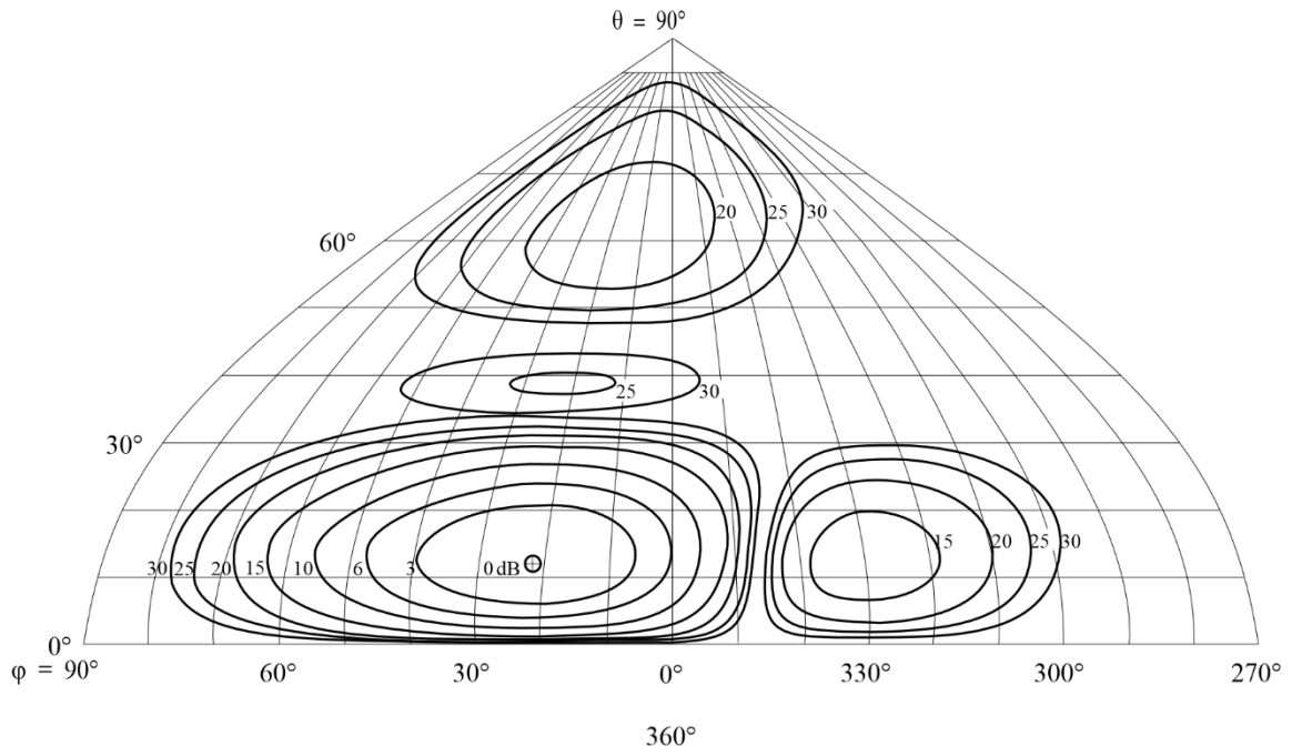
FIGURA 76C Diagrama de radiación hacia adelante
