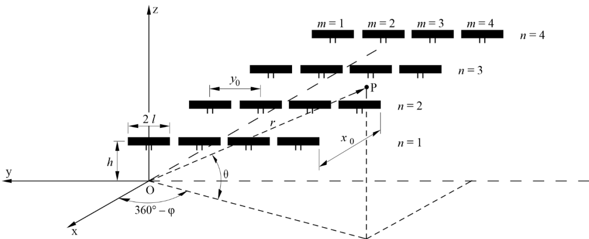
FIGURA 19 Antena de dipolos alimentados por el centro (T 4/4) para radiodifusión tropical
