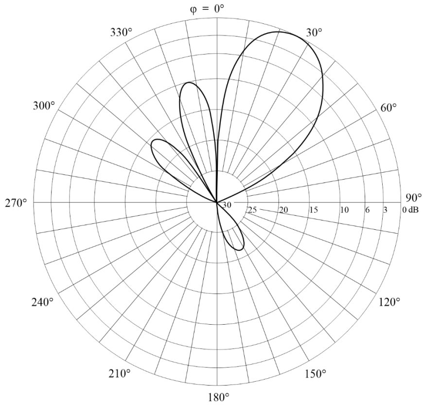
Diagrama horizontal para un ángulo de elevación de 9°
