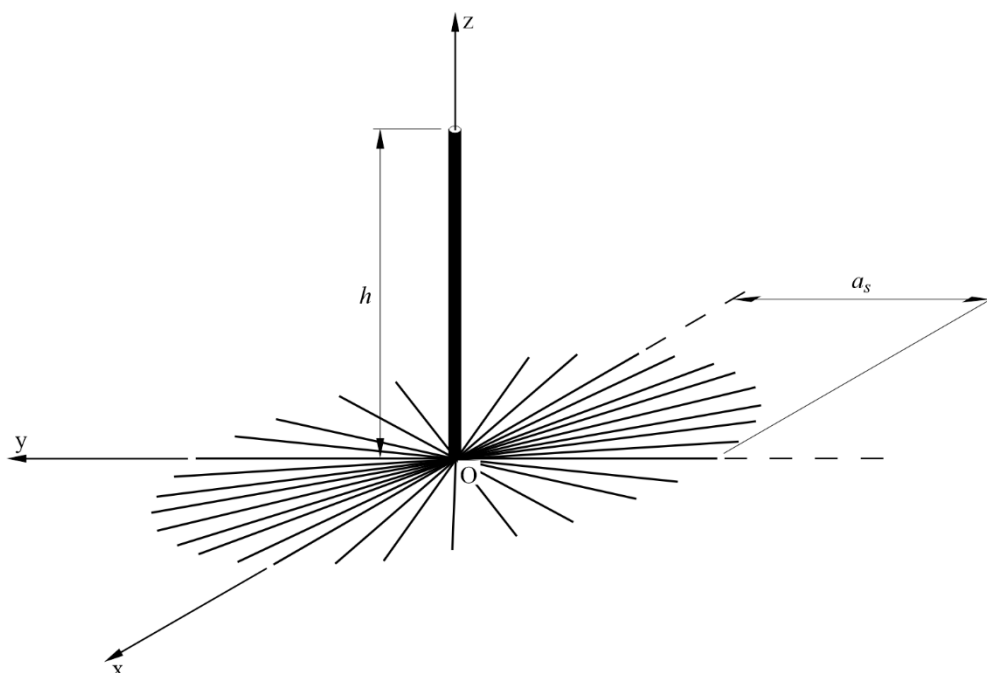
Monopolo vertical con un sistema de puesta a tierra compuesto por hilos radiales
