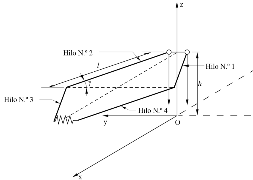
FIGURA 40 Antena rómbica horizontal
