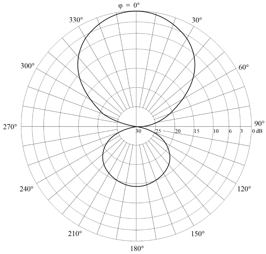
Diagrama horizontal para un ángulo de elevación de 27°
