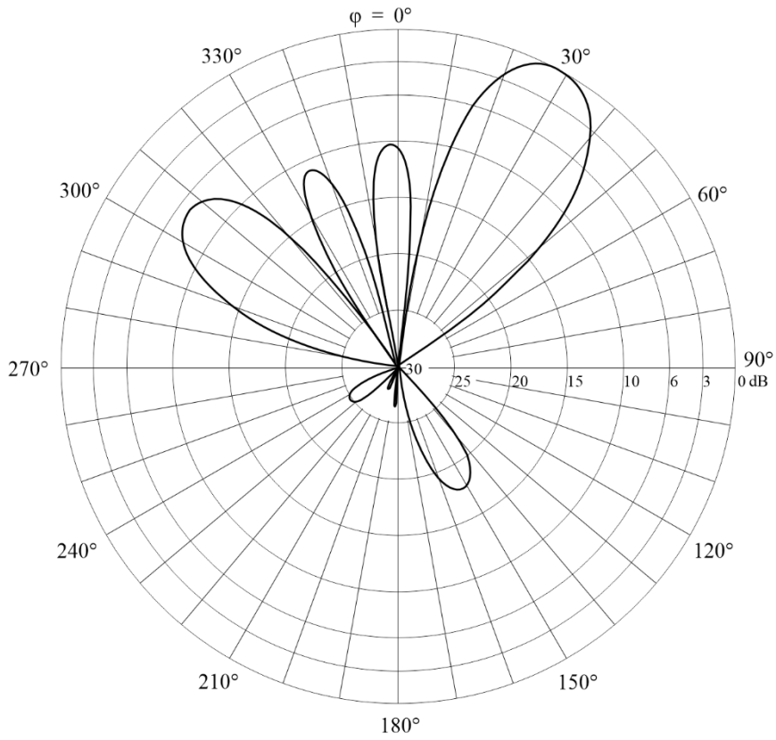
Diagrama horizontal para un ángulo de elevación de 7°
