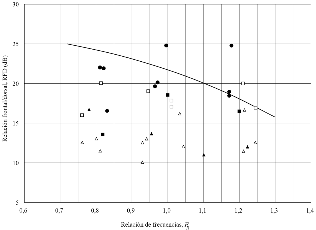
FIGURA 55 Valores de la relación frontal/dorsal (RFD) medidos y calculados para diversos tipos de antena
