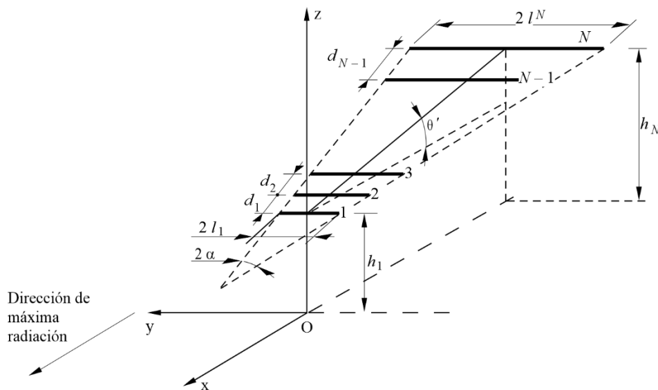
FIGURA 29 Sistema log-periódico horizontal
