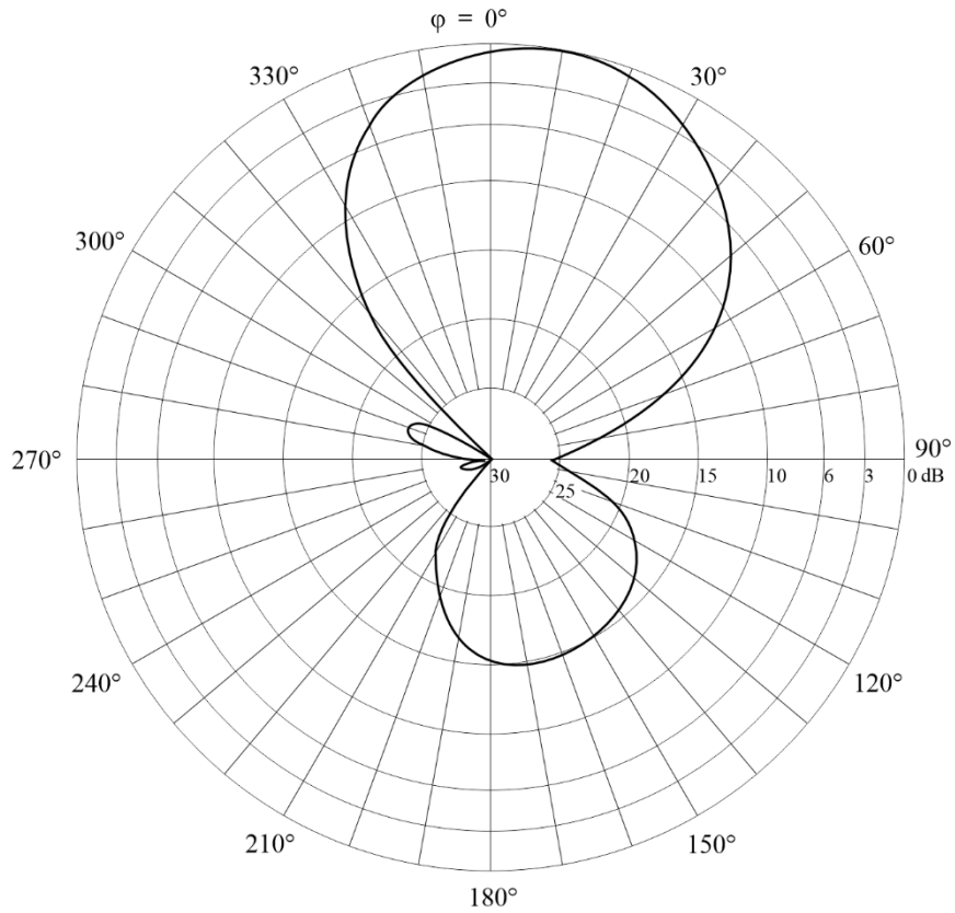
FIGURA 71B Diagrama horizontal para un ángulo de elevación de 17°
