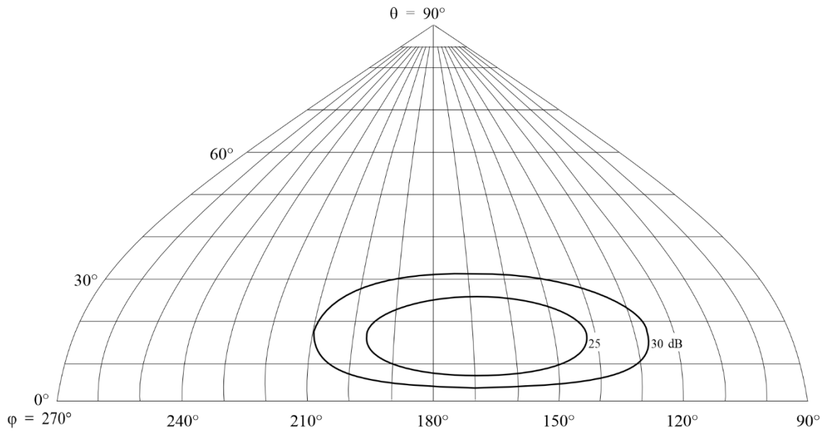
FIGURA 73D Diagrama de radiación hacia atrás
