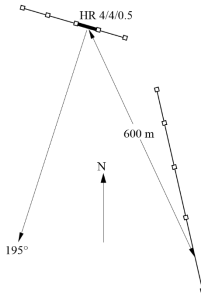
FIGURA 59 Disposición de las antenas
