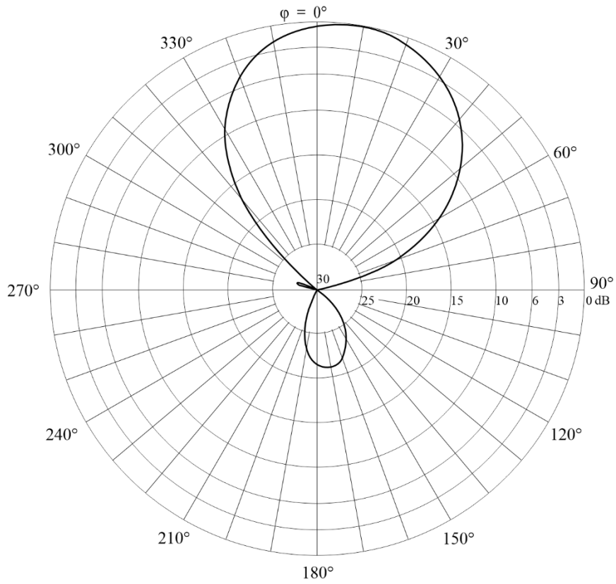
FIGURA 73B Diagrama horizontal para un ángulo de elevación de 17°
