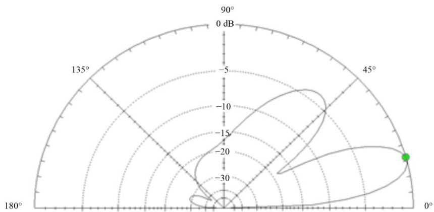
FIGURA 91A Diagrama vertical de una antena Yagi-Uda con polarización horizontal y tres elementos sintonizados en 6,8 MHz, h = 39,6 m por encima del nivel del suelo – La ganancia máxima se alcanza en un ángulo de elevación de 16^\circ
