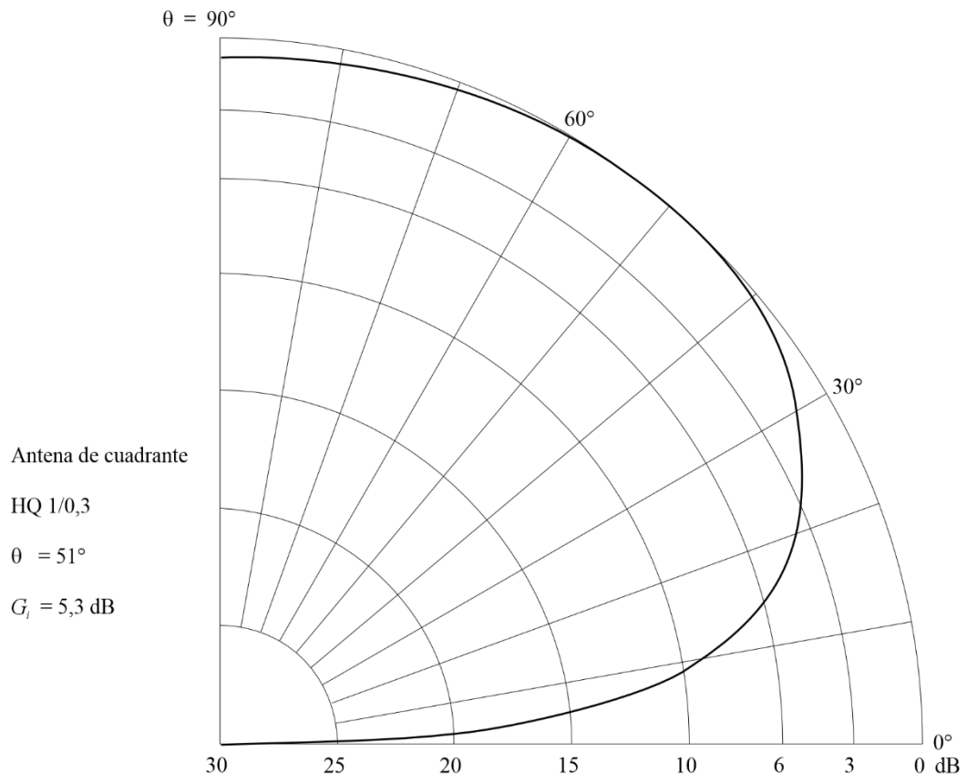
Diagrama vertical para un ángulo acimutal de 0°
