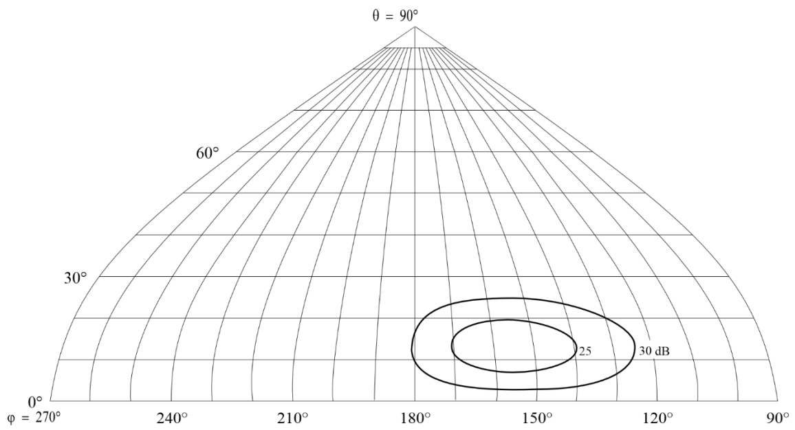
FIGURA 76D Diagrama de radiación hacia atrás
