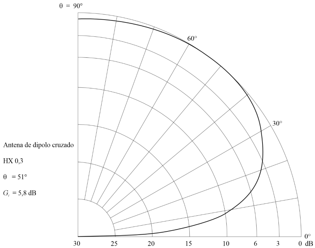
FIGURA 88A Diagrama vertical para un ángulo acimutal de 0^\circ
