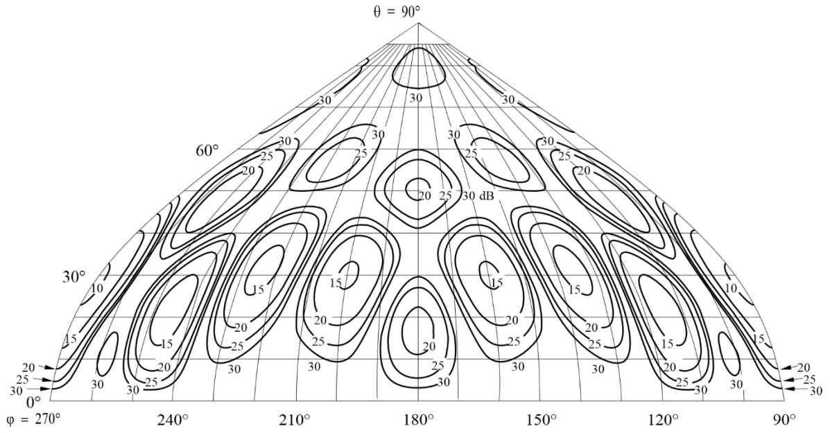
FIGURA 89D Diagrama de radiación hacia atrás
