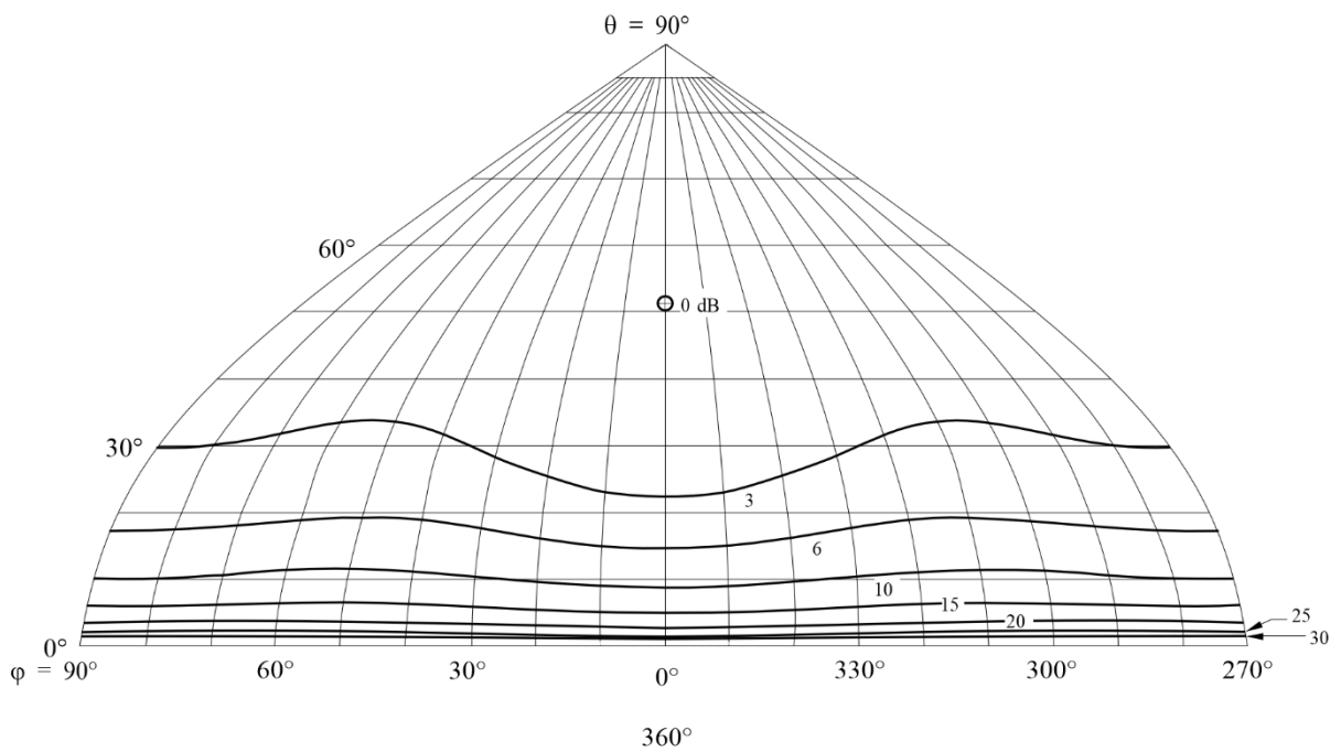
FIGURA 87C Diagrama de radiación hacia adelante
