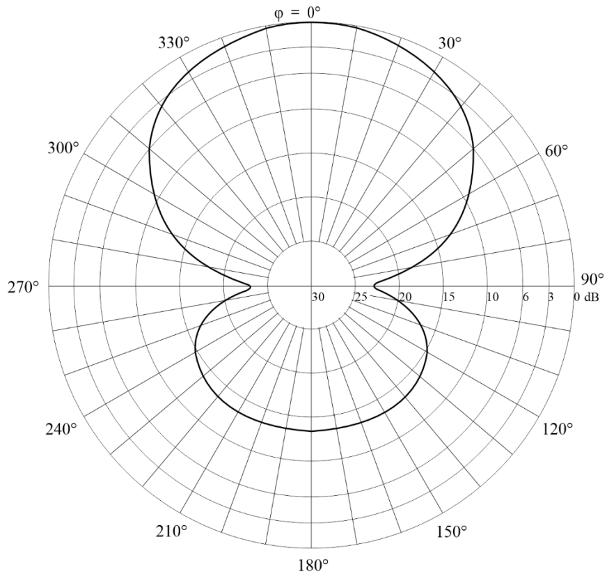
Diagrama horizontal para un ángulo de elevación de 14°
