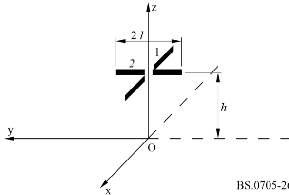
Antena de dipolo cruzado
