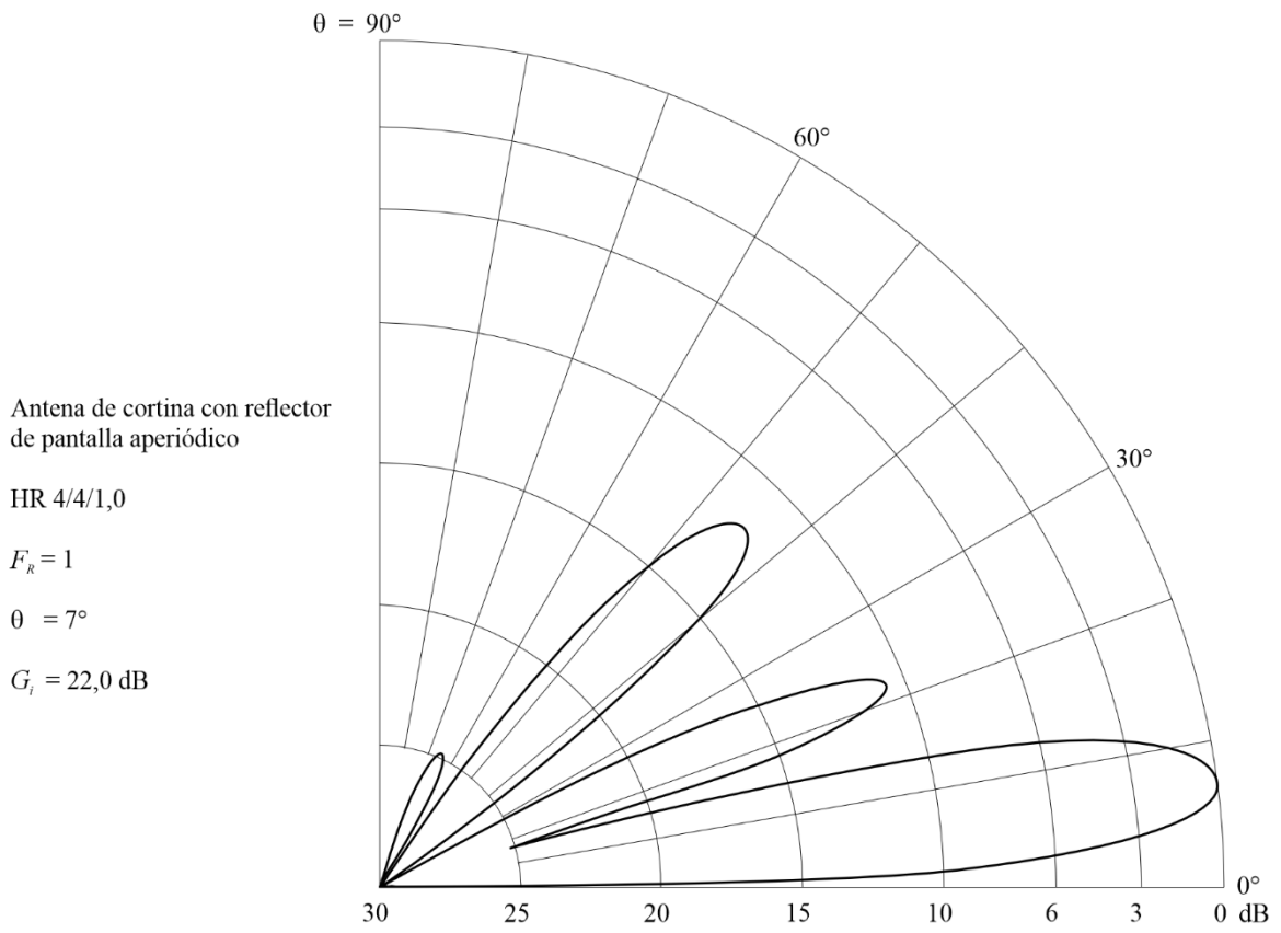
FIGURA 81A Diagrama vertical para un ángulo acimutal de 0^\circ
