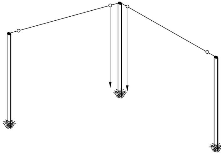
FIGURA 13 Antena de cuadrante con 2 soportes
