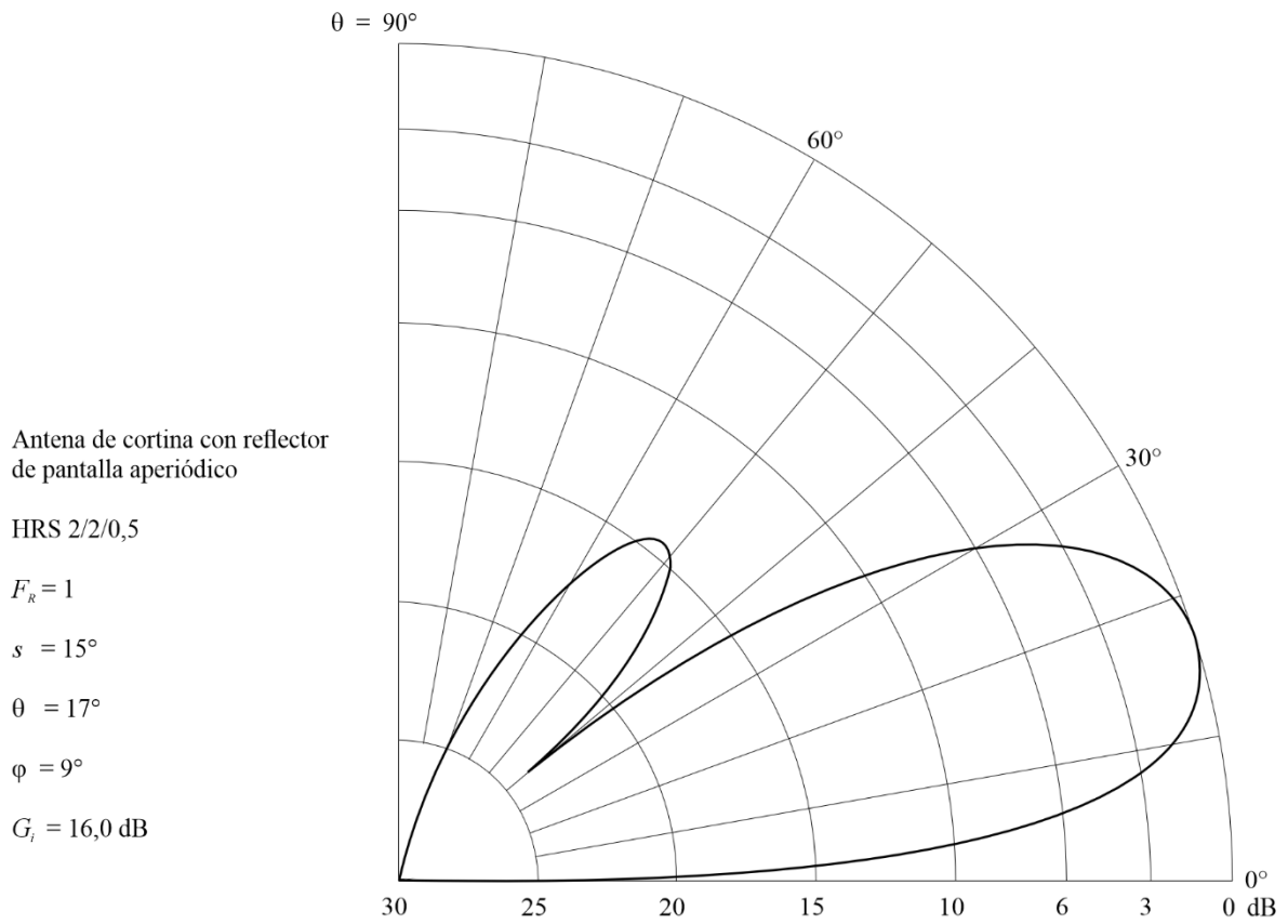
FIGURA 73A Diagrama vertical para un ángulo acimutal de 9^\circ
