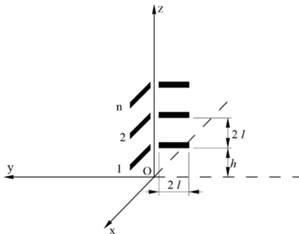
FIGURA 7 Antena de cuadrante
