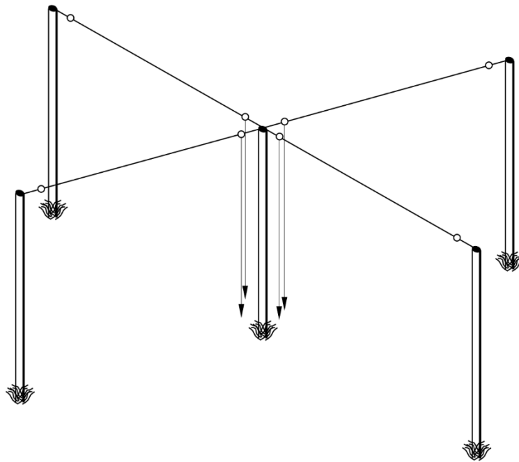
FIGURA 15 Antena de dipolos cruzados
