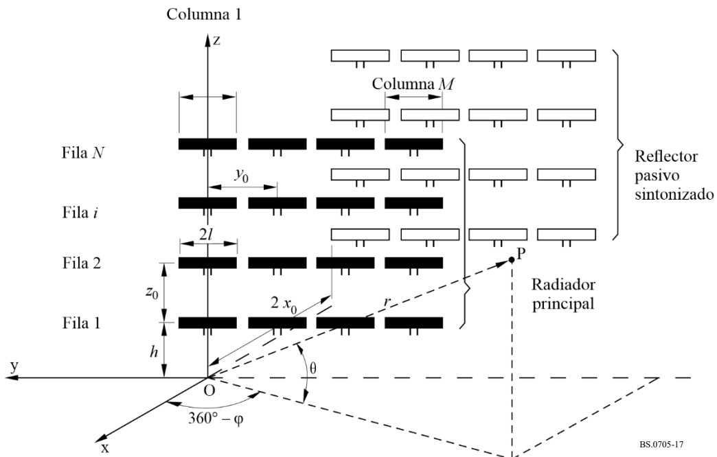
FIGURA 17 Sistema de dipolos alimentados por el centro (HR 4/4) con reflector de dipolos sintonizados
