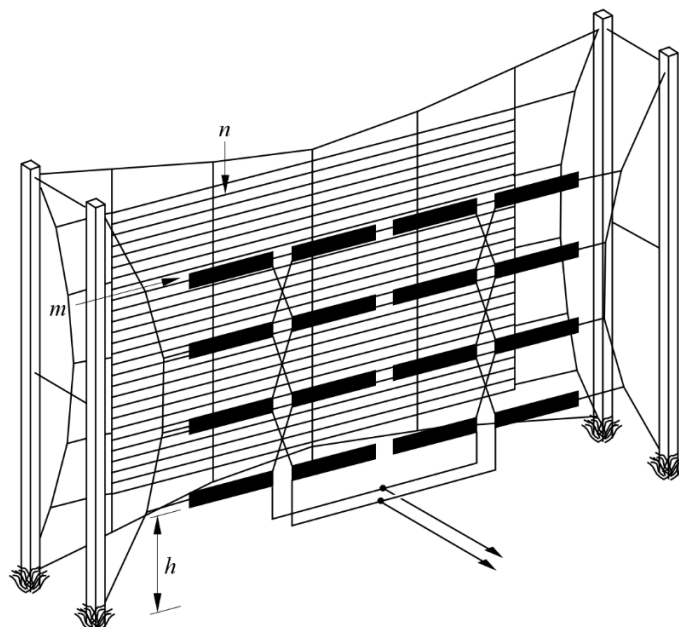
FIGURA 11 Sistema de dipolos alimentados por el extremo con reflector aperiódico
