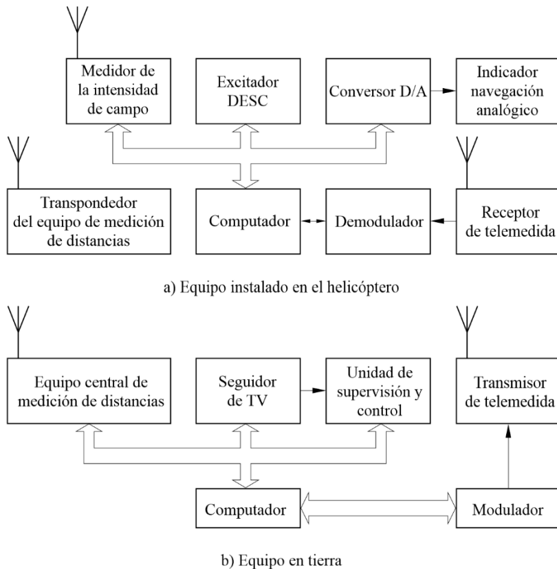
Diagrama de bloques de equipo de medición que utiliza seguimiento para la determinación de la posición
