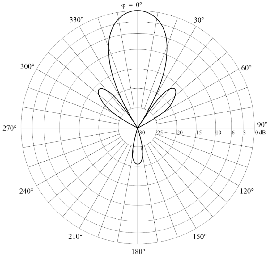
FIGURA 74B Diagrama horizontal para un ángulo de elevación de 12°
