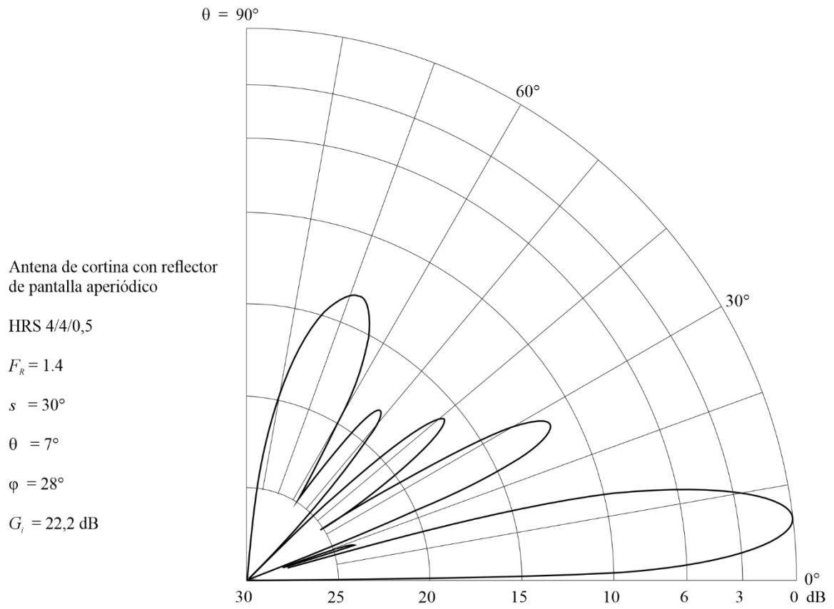
Diagrama vertical para un ángulo acimutal de 28°
