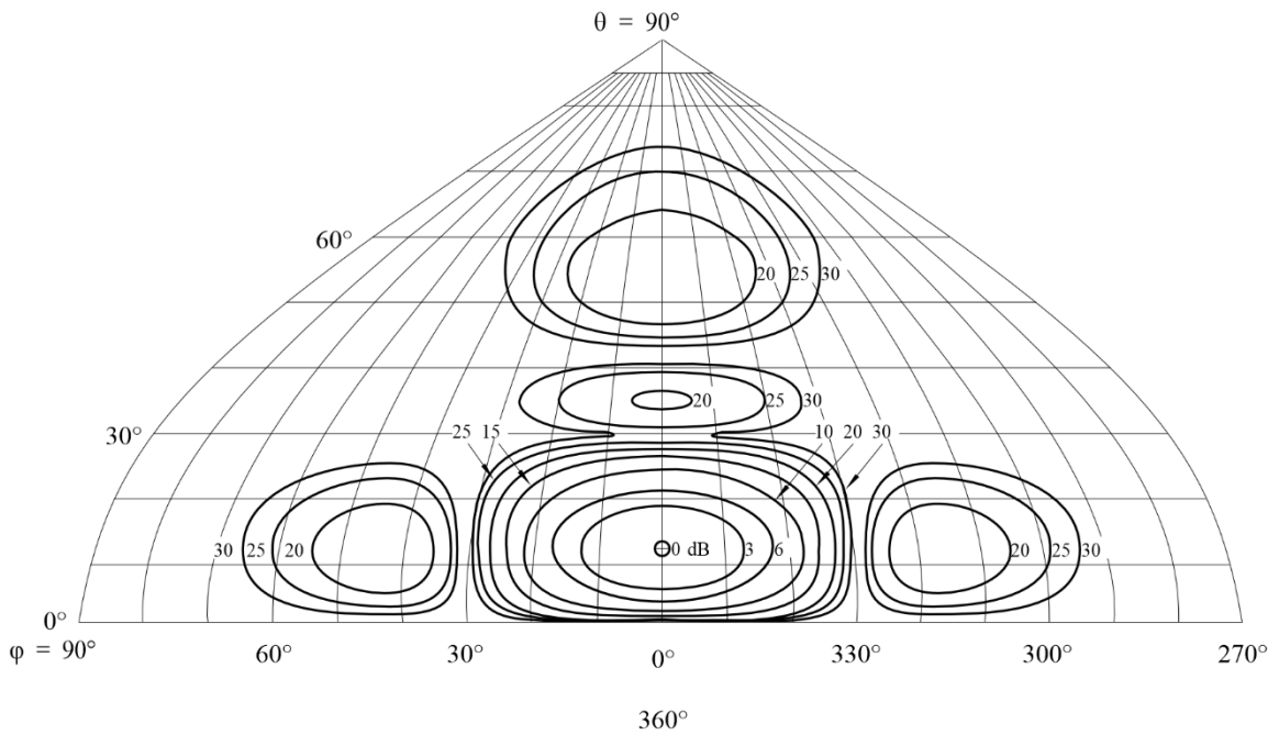
FIGURA 74C Diagrama de radiación hacia adelante
