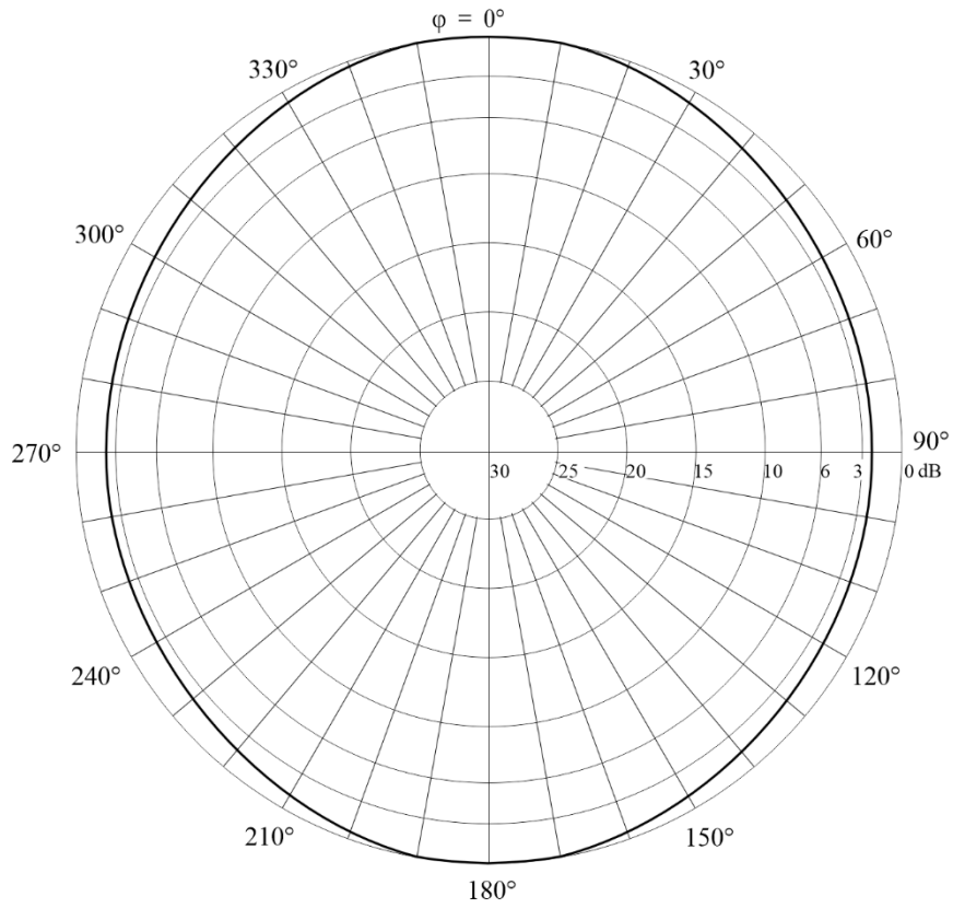
FIGURA 87B Diagrama horizontal para un ángulo de elevación de 51°
