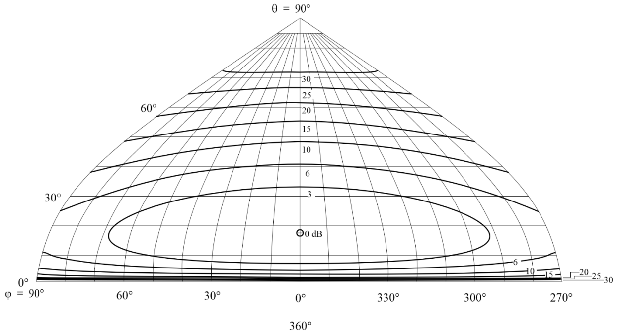
FIGURA 86C Diagrama de radiación hacia adelante
