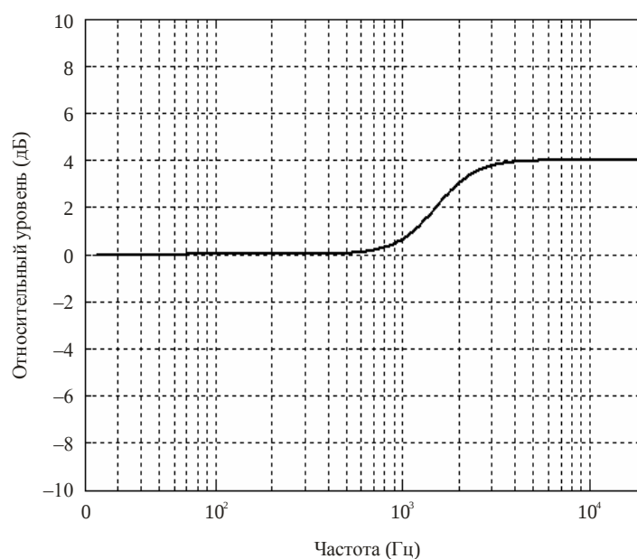
Частотная характеристика первой ступени предварительного фильтра, используемой для обеспечения учета акустического воздействия головы
