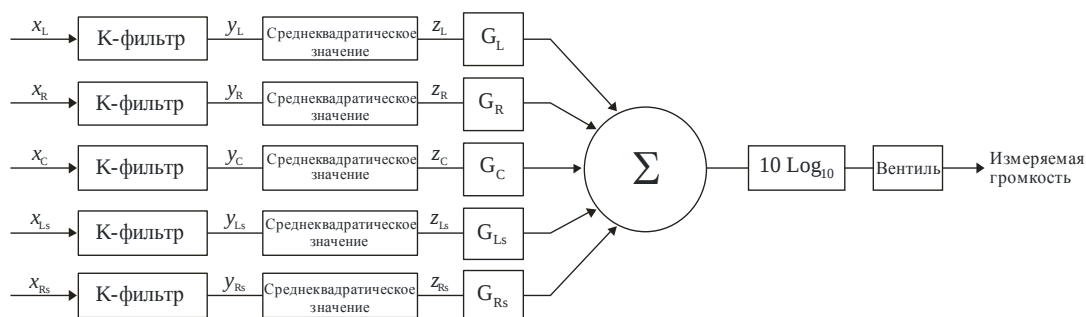
Упрощенная блок-схема алгоритма многоканального измерения громкости
