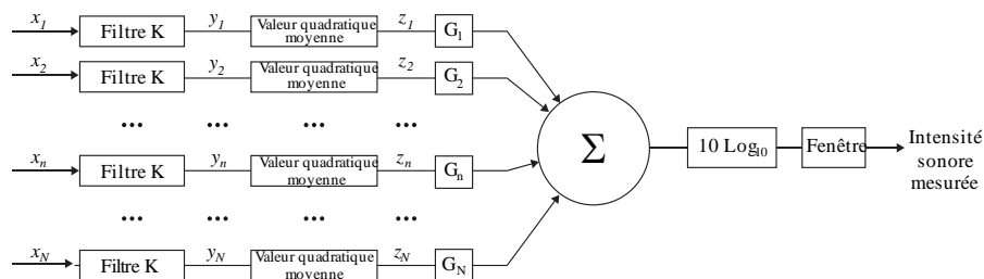
Schéma fonctionnel simplifié de l'algorithme de mesure objective de l'intensité sonore dans le cas de configurations de haut-parleurs du système sonore évolué
