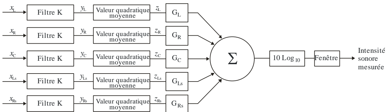
Schéma fonctionnel de l'algorithme de mesure de l'intensité sonore multicanal
