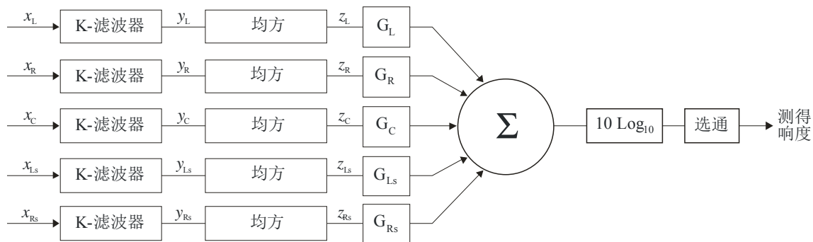
多声道响度算法简略方框图
