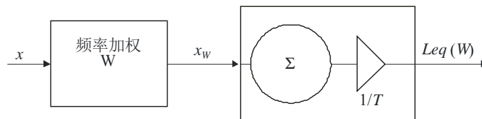
简单的基于能量响度测量方框图
