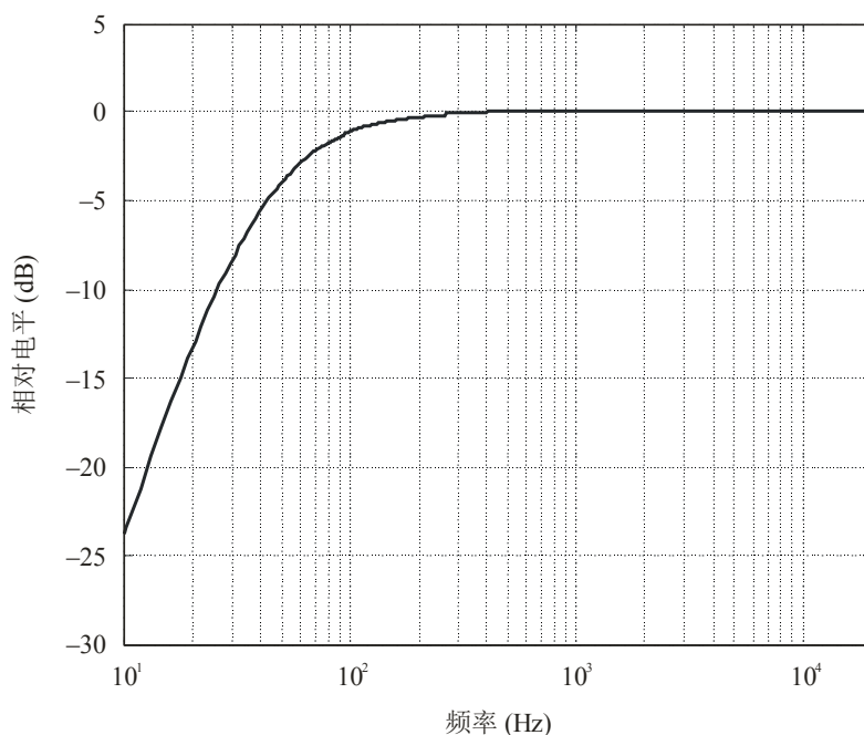
图4 第二级加权曲线
