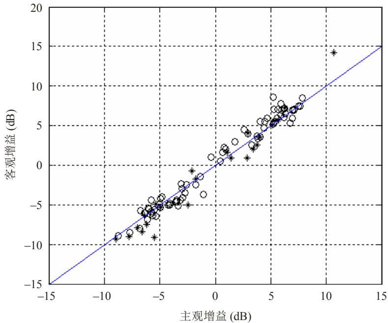
单声道Leq(RLB)响度计对比主观结果 (r = 0.982)
