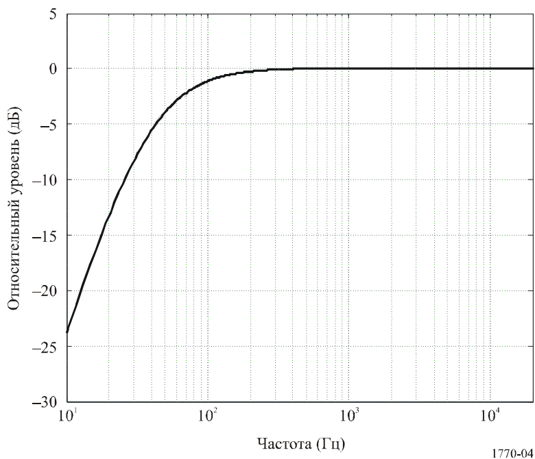
Взвешивающая кривая RLB
