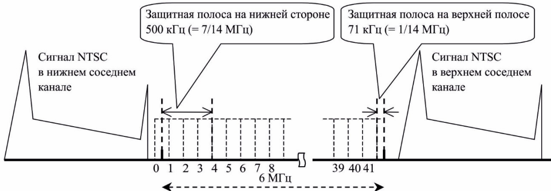
РИСУНОК 5 Защитные полосы для обеспечения возможности совместной работы с сигналом аналогового телевидения в соседнем канале
