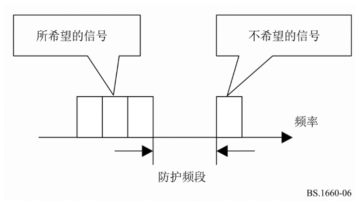
图 6 防护频段和信号安排
