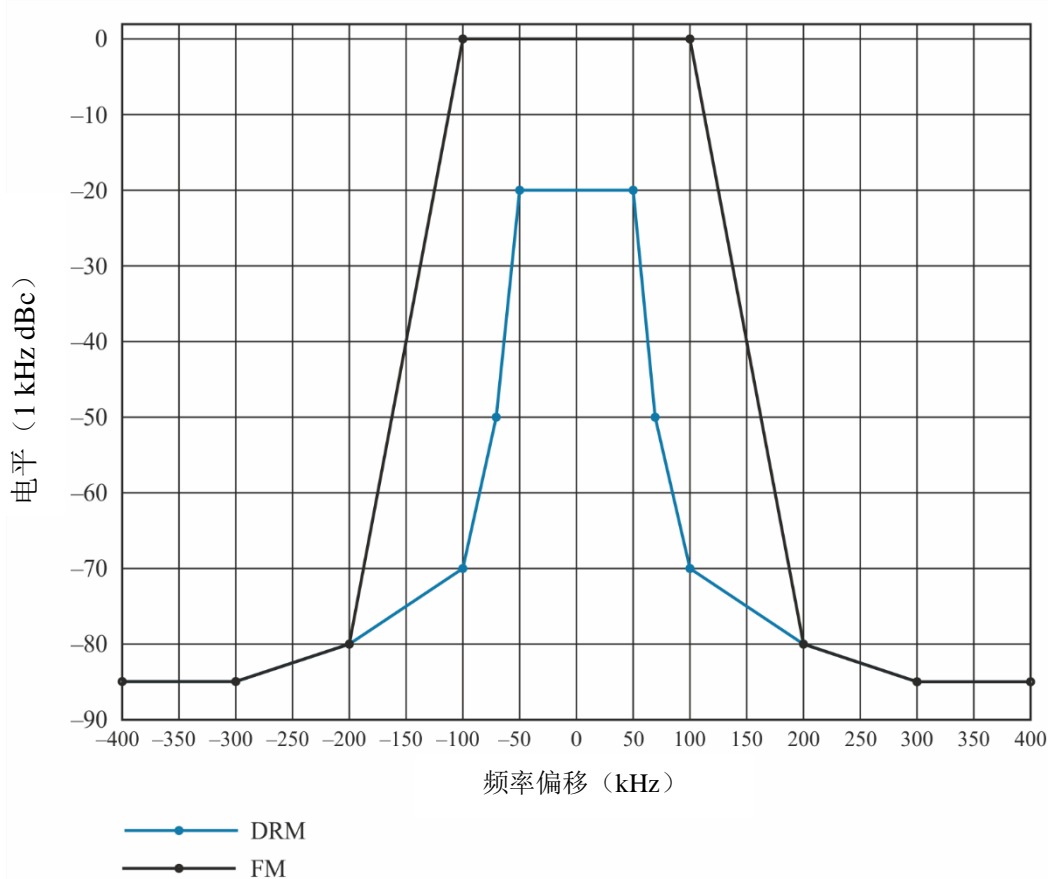
甚高频频段II的调频和甚高频频段I及甚高频频段II的DRM的带外频谱掩膜
