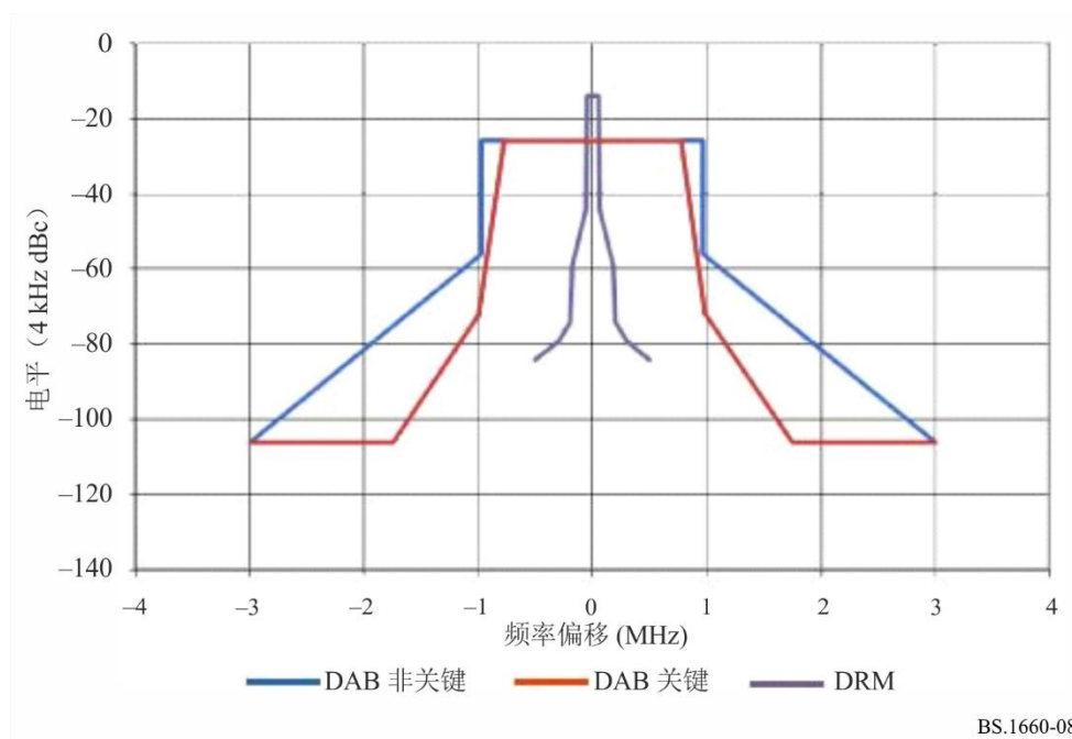
甚高频频段III的DAB和DRM带外频谱掩膜
