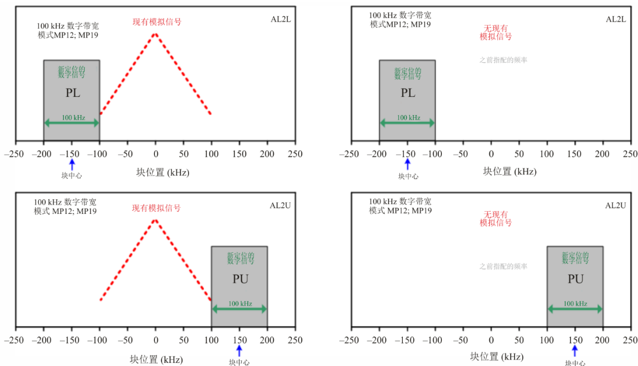
高清无线电信系统100-kHz数字块定位示例
