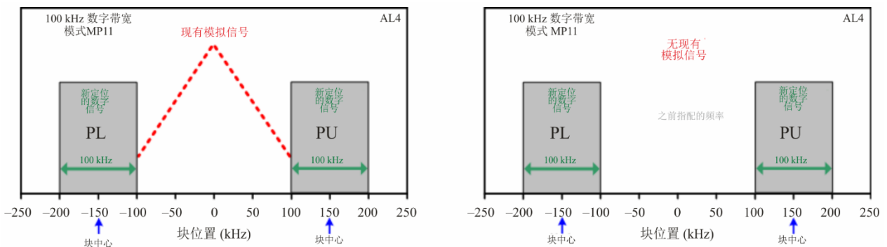
高清无线电系统2 x 100-kHz数字块定位示例
