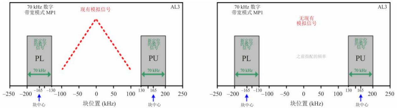
高清无线电系统2 x 70-kHz数字块定位示例
