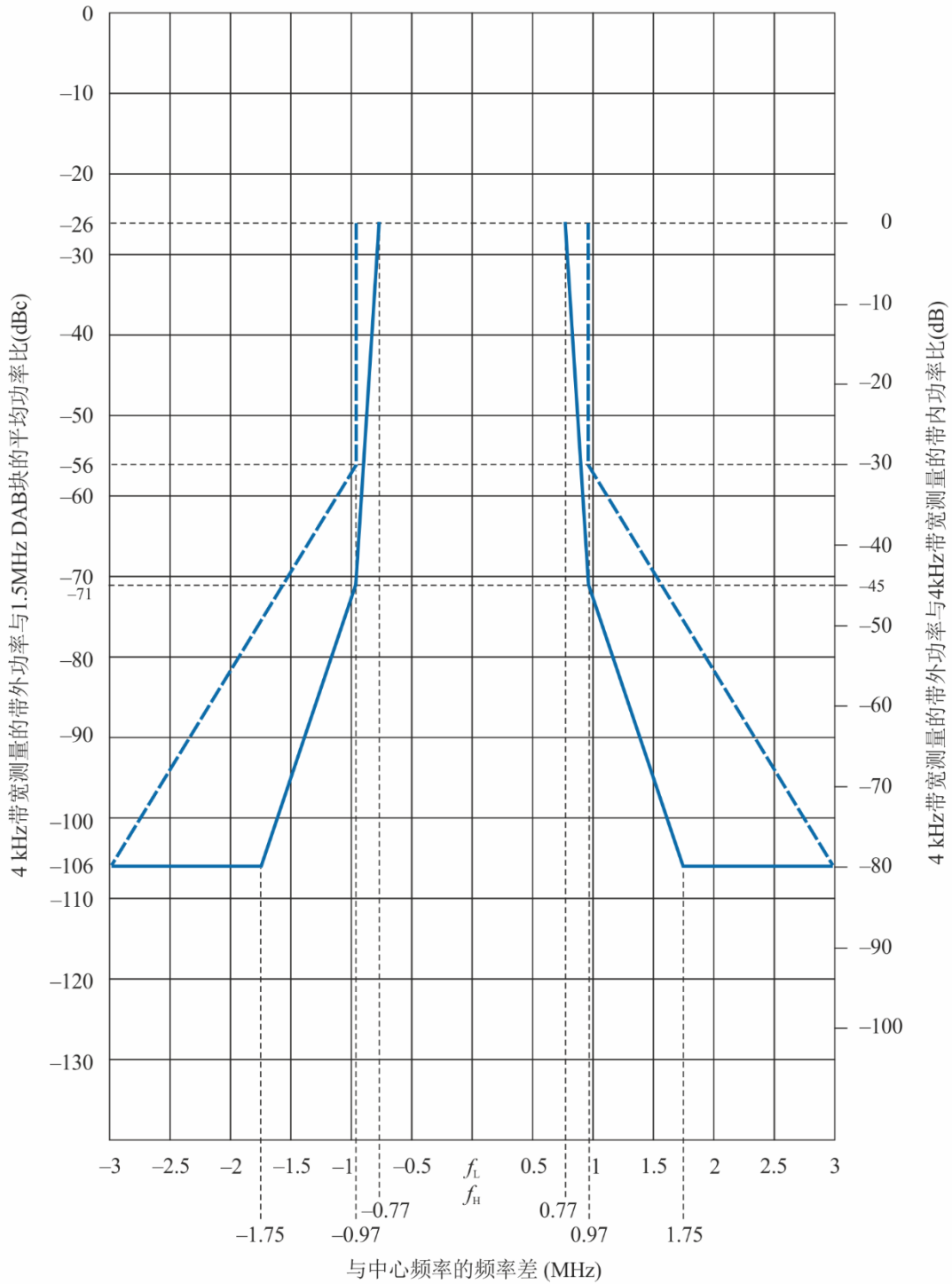
图2 用于DAB带外辐射的频谱掩膜
