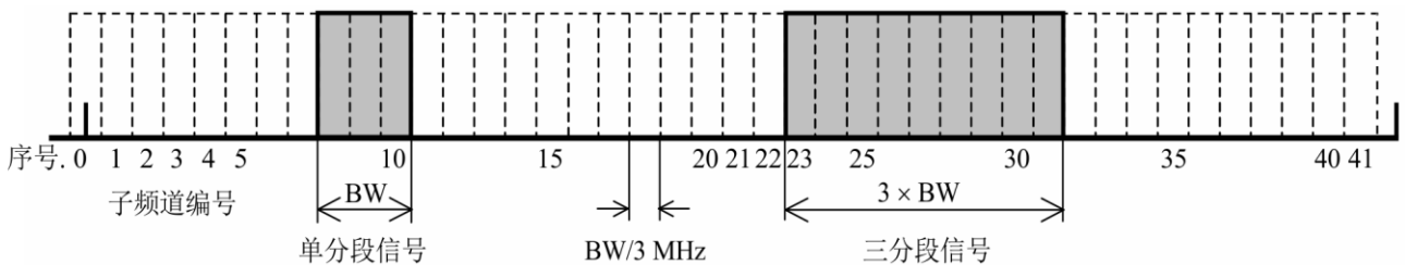
图4 关于子频道的规定
