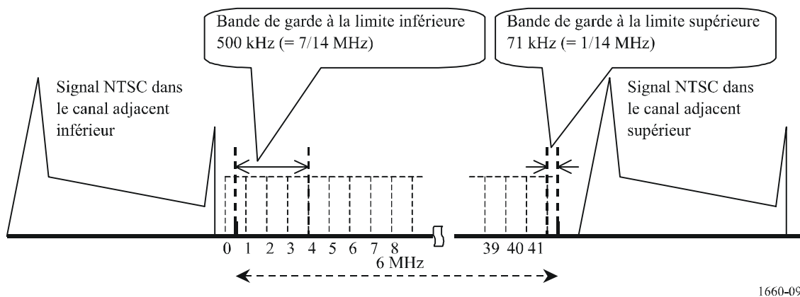
FIGURE 9 Bandes de garde pour une coexistence avec un signal de télévision analogique adjacent
