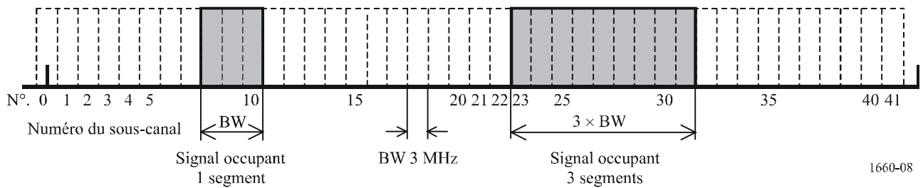
FIGURE 8 Définition d'un sous-canal
