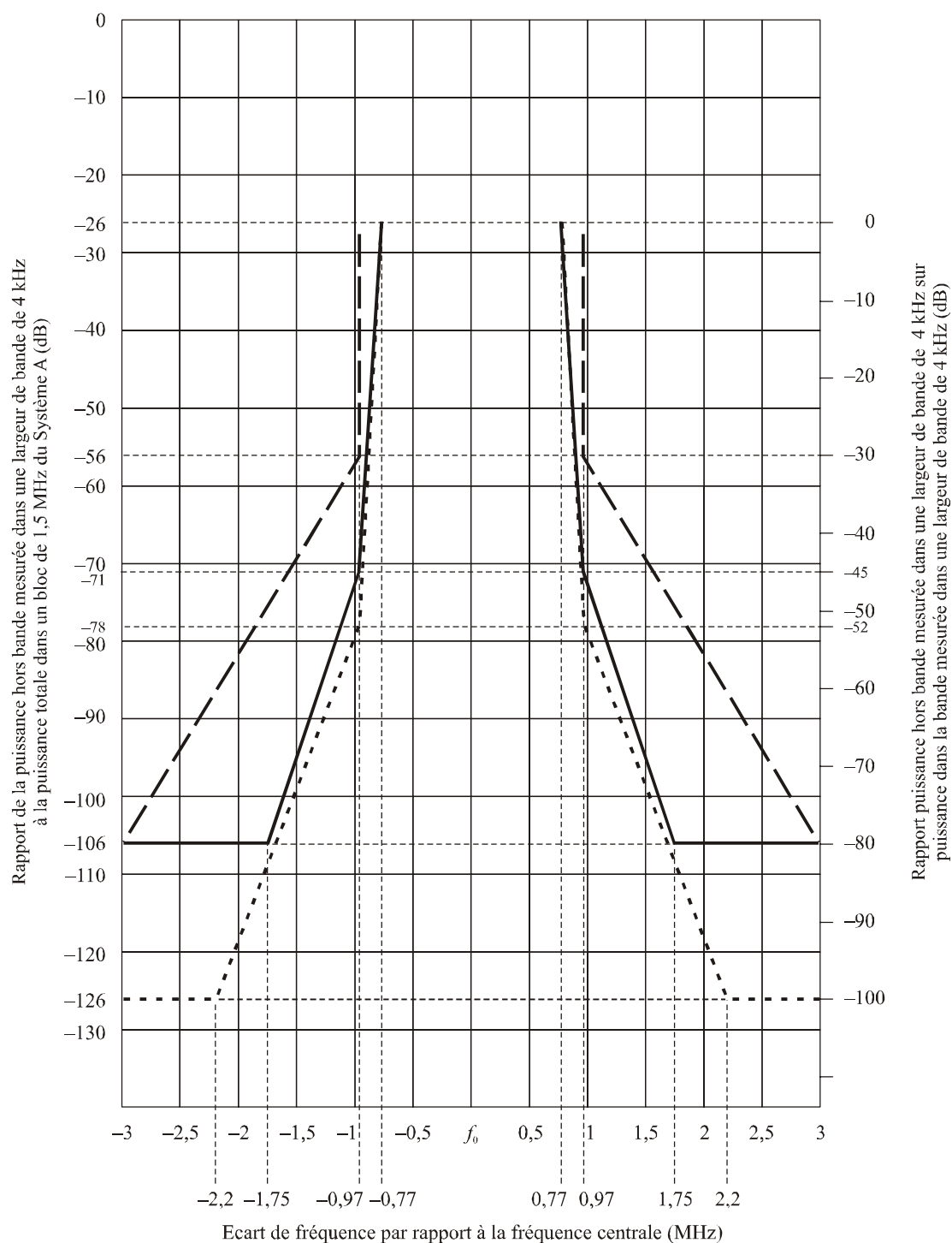
FIGURE 1 Gabarits spectraux hors bande pour un signal d'émission du Système A
