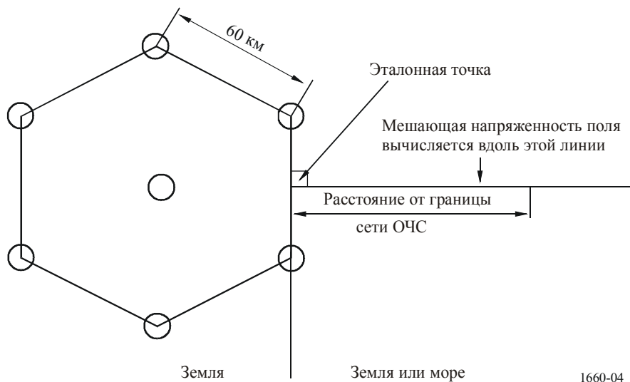
РИСУНОК 4 Информация, относящаяся к вычислению мешающей напряженности поля для эталонной сети
