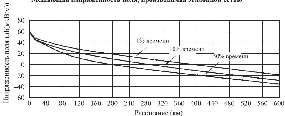
а) Изменение напряженности поля от расстояния: земля
