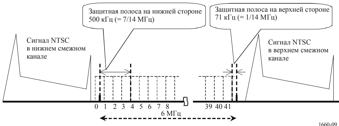
РИСУНОК 9 Защитные полосы для сосуществования со смежным сигналом аналогового телевидения
