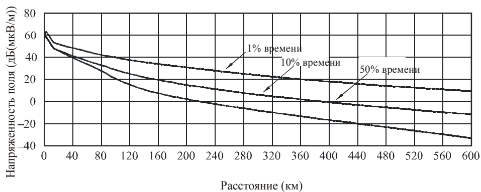
в) Изменение напряженности поля от расстояния: теплое море 1660-06
