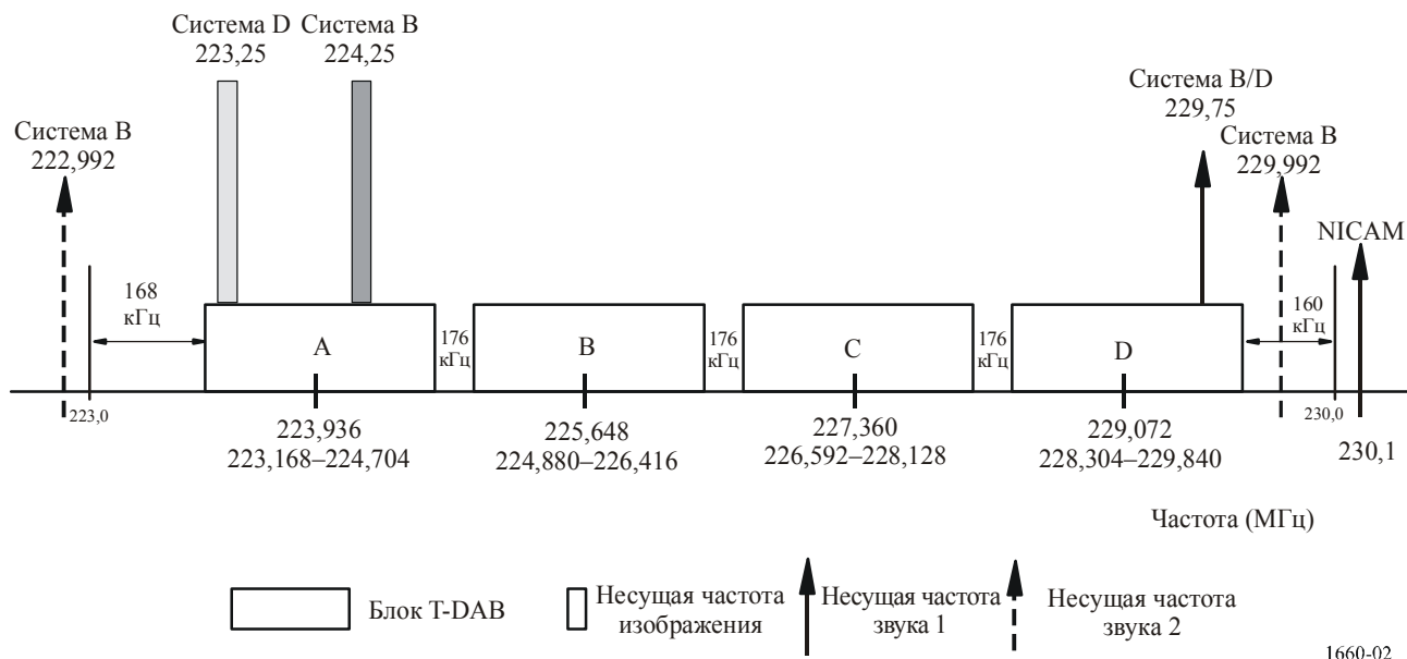
РИСУНОК 2 Позиция блоков T-DAB в канале 12
